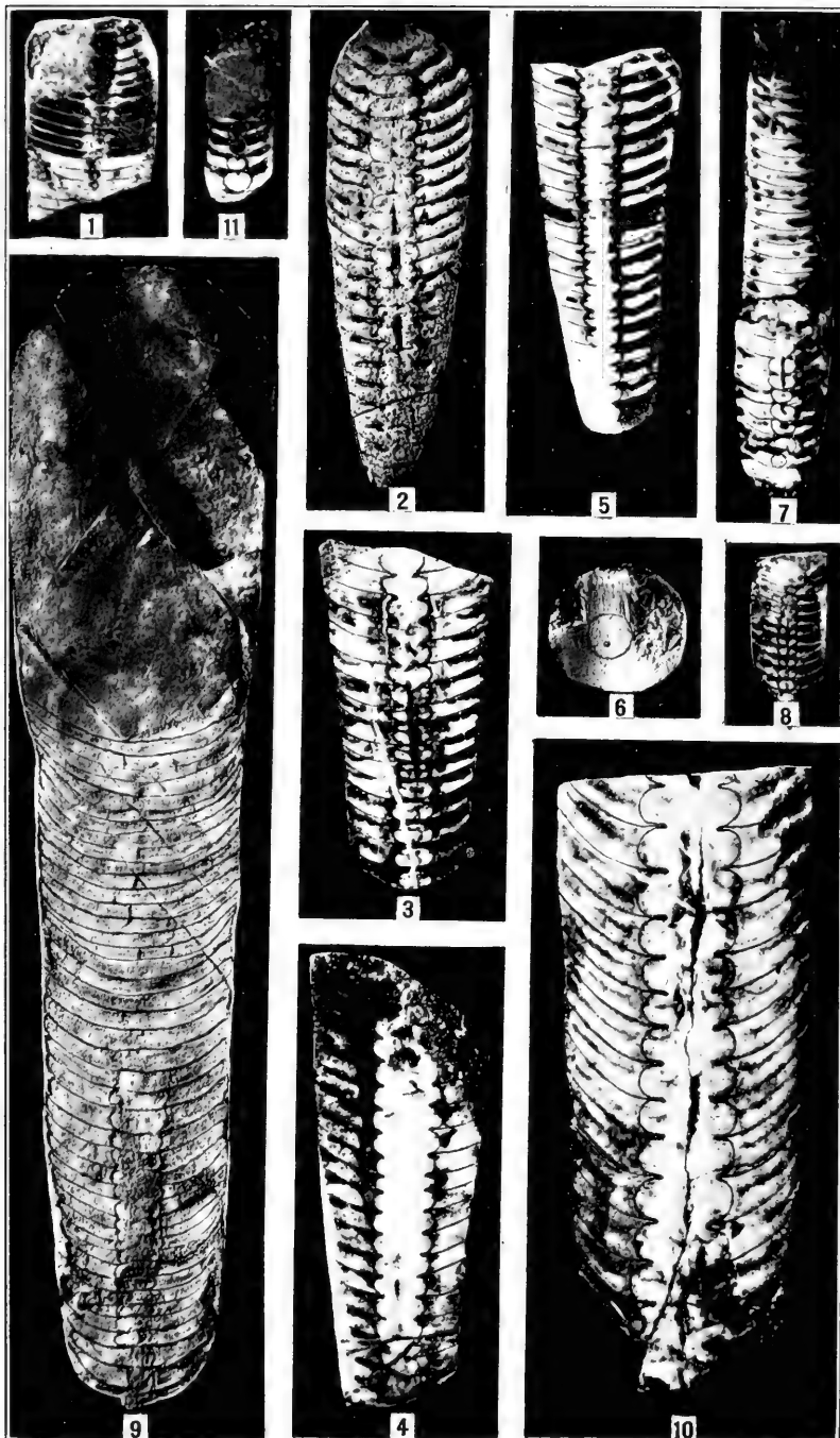
SSUYEN FORMATION
