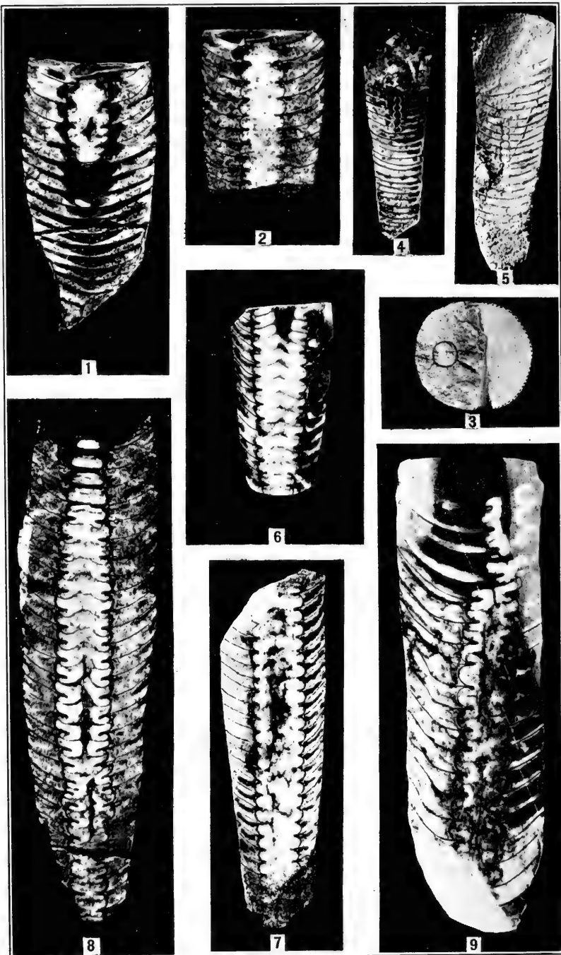
SSUYEN FORMATION
