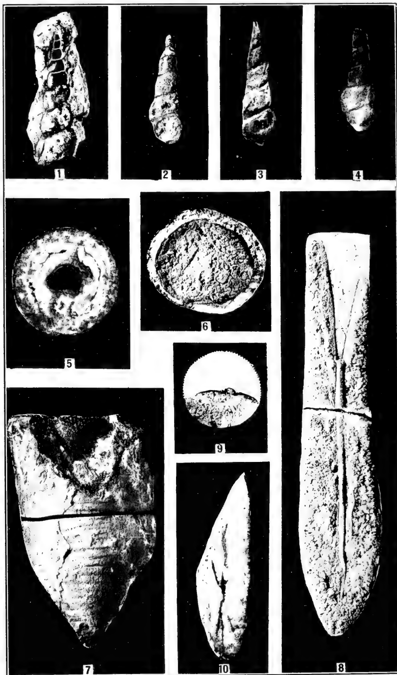
SANTAO FORMATION
