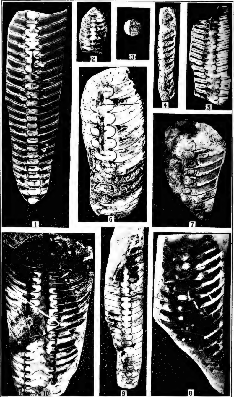
SSUYEN FORMATION
