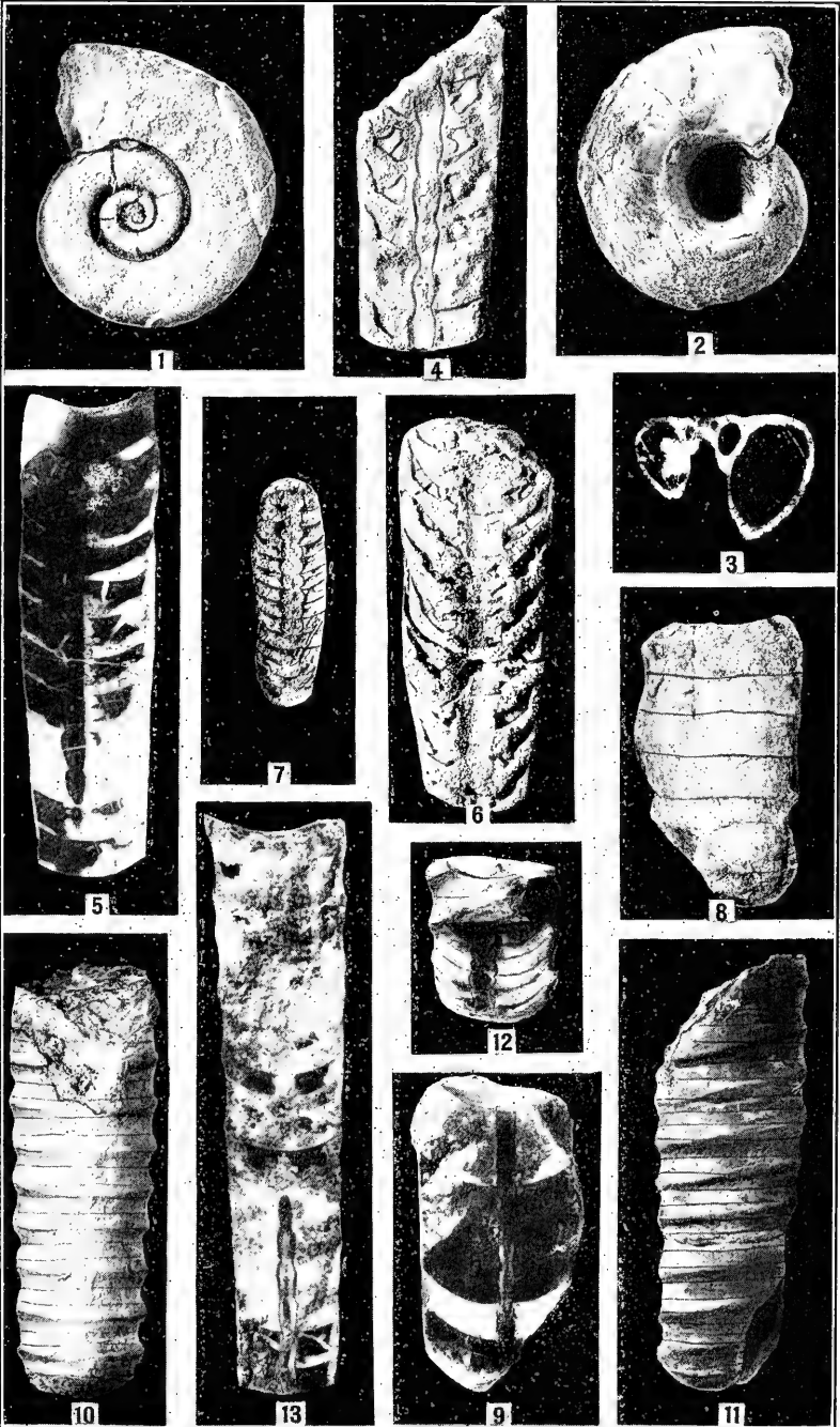
SSUYEN FORMATION
