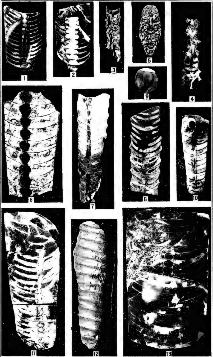
SSUYEN FORMATION
