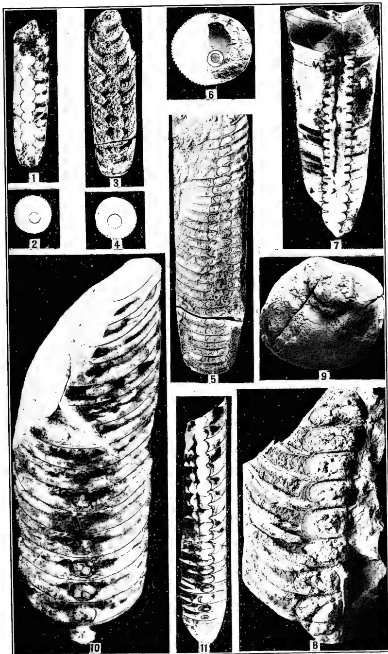
SSUYEN FORMATION
