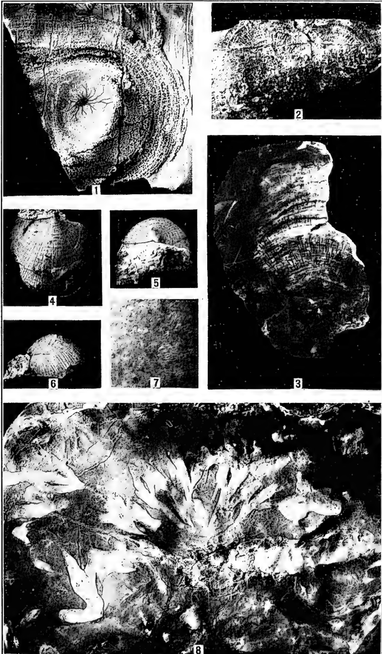
SSUYEN FORMATION
