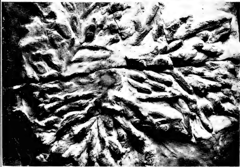
SSUYEN FORMATION
