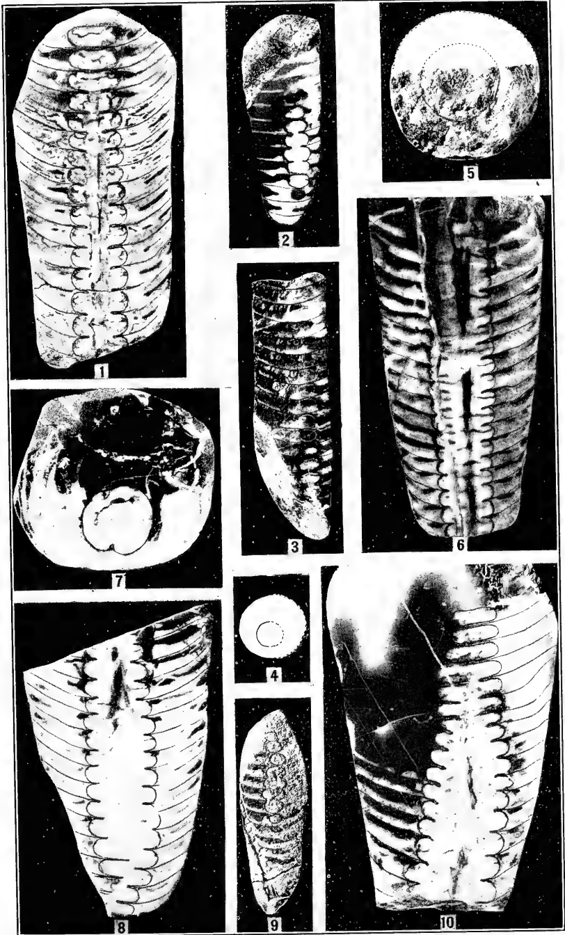
SSUYEN FORMATION
