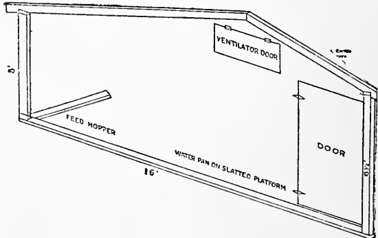
END VIEW. FIG. 27.
