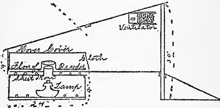
HOMEMADE BROODER. FIG. 15.
