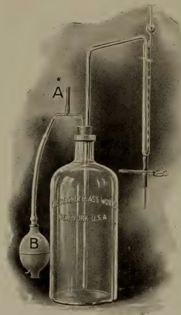
Fig. 24. Acid Tester.
