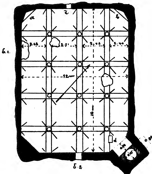
Fig. 1. Grundrifs.
