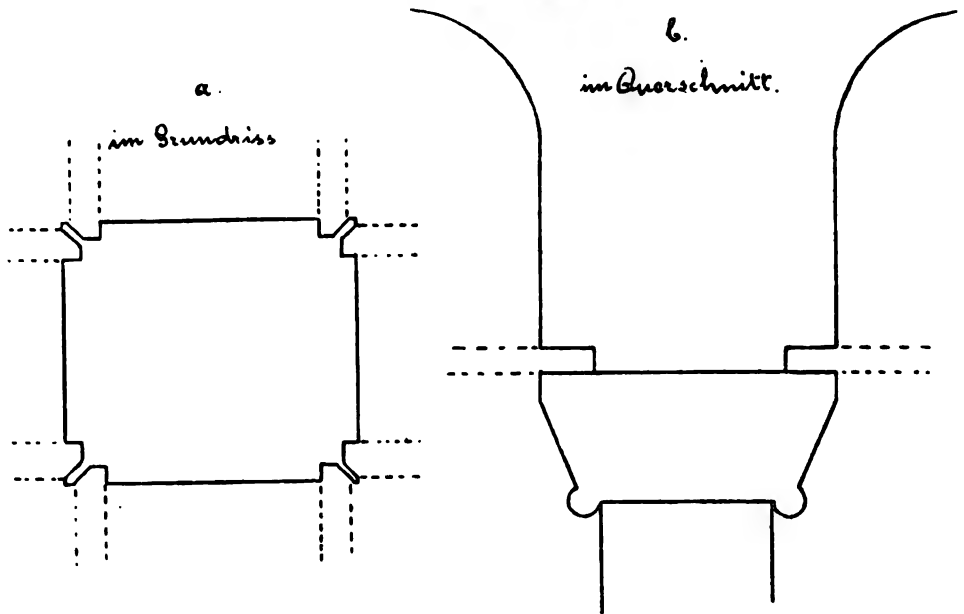
Fig. 4. Verankerungssystem.
