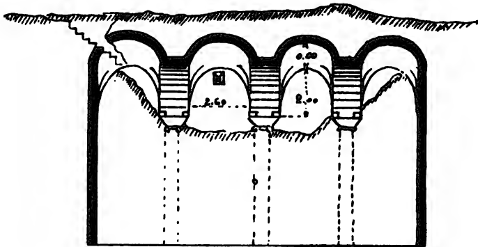
Fig. 2. Querschnitt.
