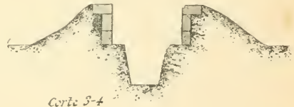
Corte 3-4
