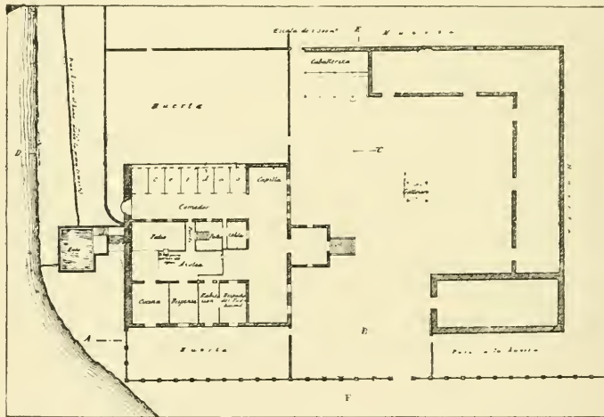
Plano de la Casa-hacienda de Imus.
