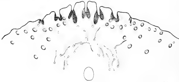
Aspidiotus Marlatti
