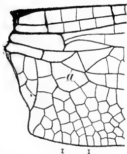
FIG. 31.— OPHIOGOMPHUS .
