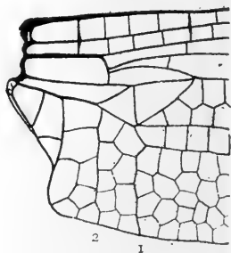
FIG. 33.— HERPETOGOMPHUS .
