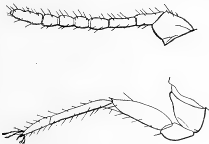
FIG. 34.— DACTYLOPIUS TRIFOLII .
