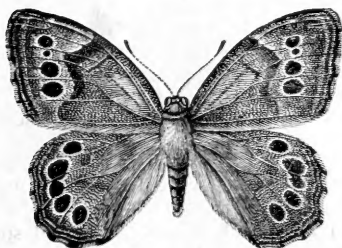
DERIS PORTLANDIA.
