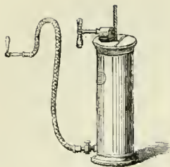
Irrigateur Éguisier.
