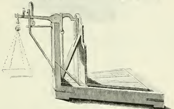
Fig. 21. Basculé triangulaire.
