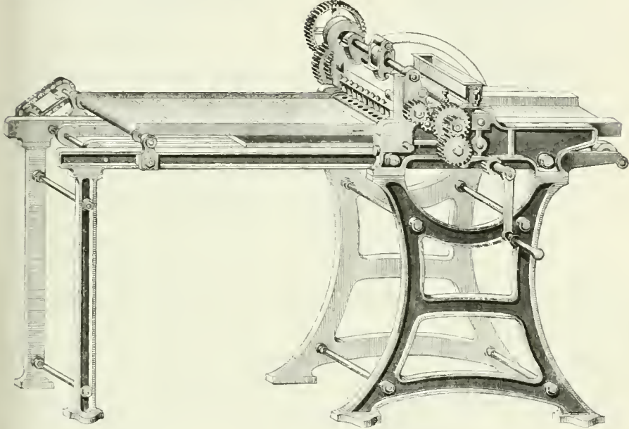
Machine à fabriquer les pastilles de notre laboratoire. (Voir pour le prix des différentes grandeurs, p. 336.)
