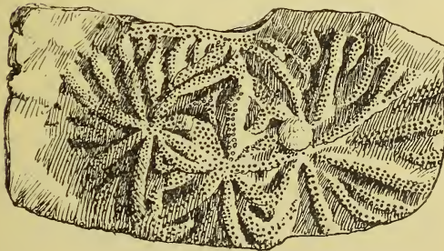
FIG. 11.— Actinopora disticha ; × 3.
