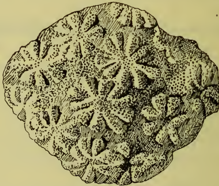
FIG. 16.— Multitubigera sulcata ; × 3.
