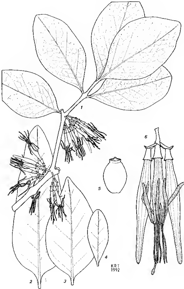
Pl. 13. - Amylotheca dictyopheba (F. Muell.) Tiegh. : 1, rameau florifère \times 1/2 ; 2-4, feuilles \times 1/2 ; 5, fruit \times 2 ; 6, triade \times 1,5 (1, MacKee 26422 ; 2, MacKee 12,352 ; 3, MacKee 12577 ; 4, MacKee 27005 ; 5, MacKee 22285 ; 6, MacKee 27192).
