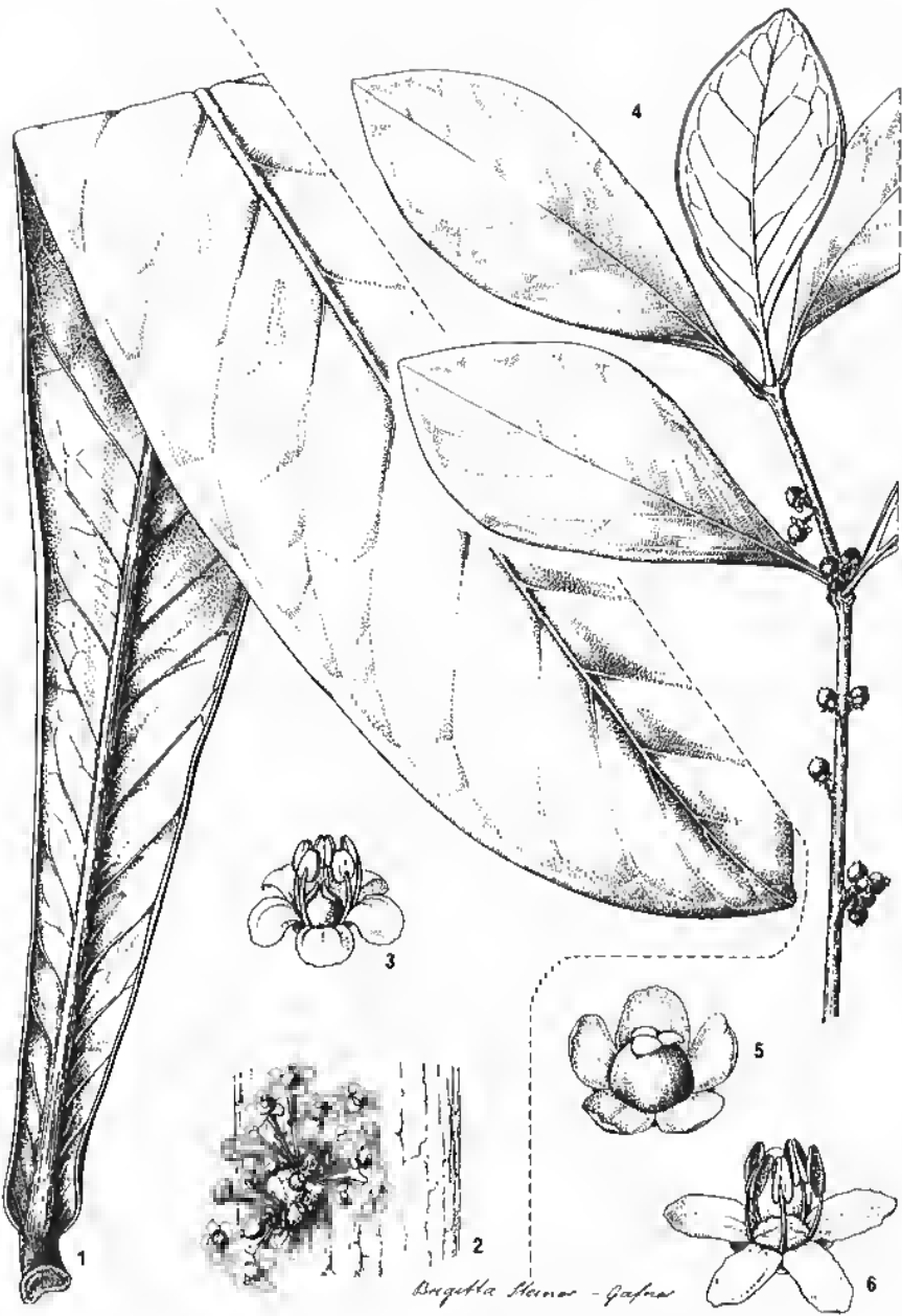
Pl. 10. - Salaciopsis megaphylla (J. Poiss. ex Guillaumin) Loes. : 1, feuille \times 2/3 ; 2, fascicule de fleurs \times 2 ; 3, fleur \times 6 (1, 2, MacKee 21140 ; 3, MacKee 17293). - S. glomerata Hürl. : 4, rameau fructifère \times 1 ; 5, fleur \times 6 ; 6, fleur \times 6 (4, 5, MacKee 27634 ; 6, MacKee 33775).
