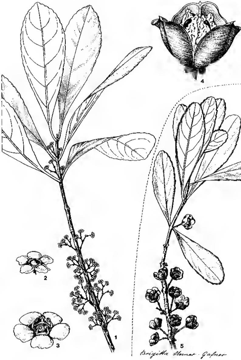
Pl. 9. — Menepetalum schlechteri Loes. subsp. schlechteri : 1, rameau florifère \times 1 ; 2, fleur ♀ \times 6 ; 3, fleur ♂ \times 6 ; 4, fruit avec les graines ailées \times 3 (1, 2, MacKee 14631; 3, McPherson 2117; 4, McPherson 4821). — Subsp. crassiusculum I.H. Müller: 5, rameau fructifère \times 1 (Müller 155).
