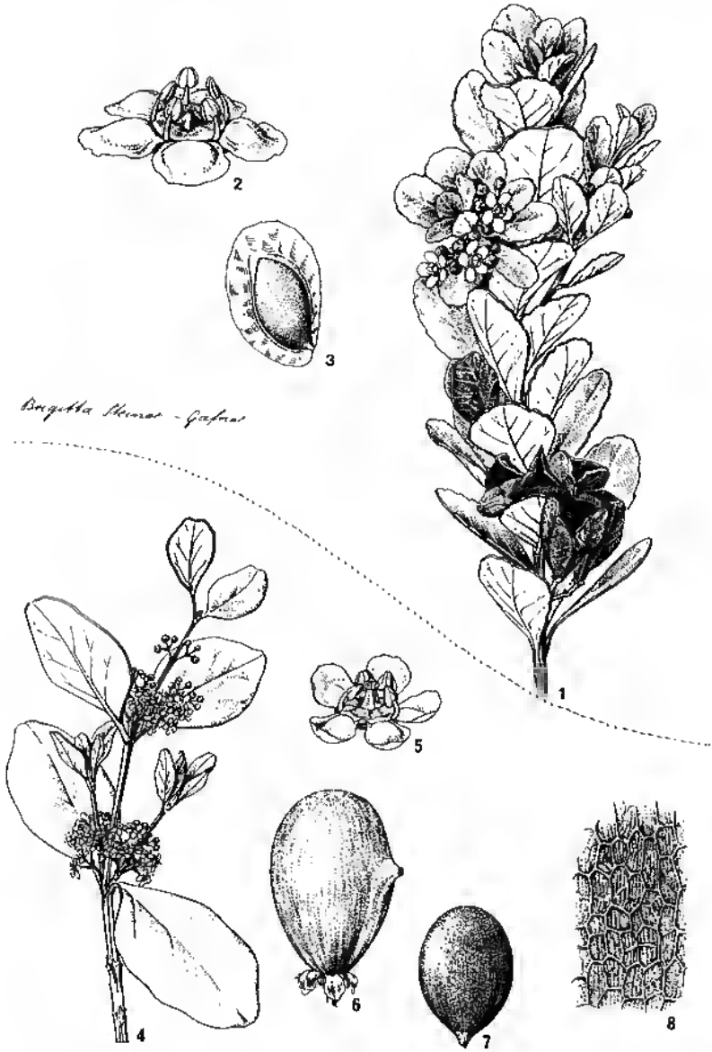
Pl. 6. — Peripterygia marginata (Baill.) Loes.: 1, rambeau feuillé avec fleurs et fruits \times 1 ; 2, fleur \times 6 ; 3, graine \times 3 (Müller 10). — Pleurostyliia opposita (Wall.) Alston: 4, rambeau florifère \times 1 ; 5, fleur \times 6 ; 6, noix \times 6 ; 7, graine \times 6 ; 8, détail du testa (4, 5, Müller 221; 6-8, MacKee 29763).
