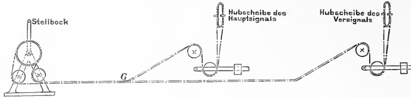
Abb. 1. Abzweigende Drahtleitung.
