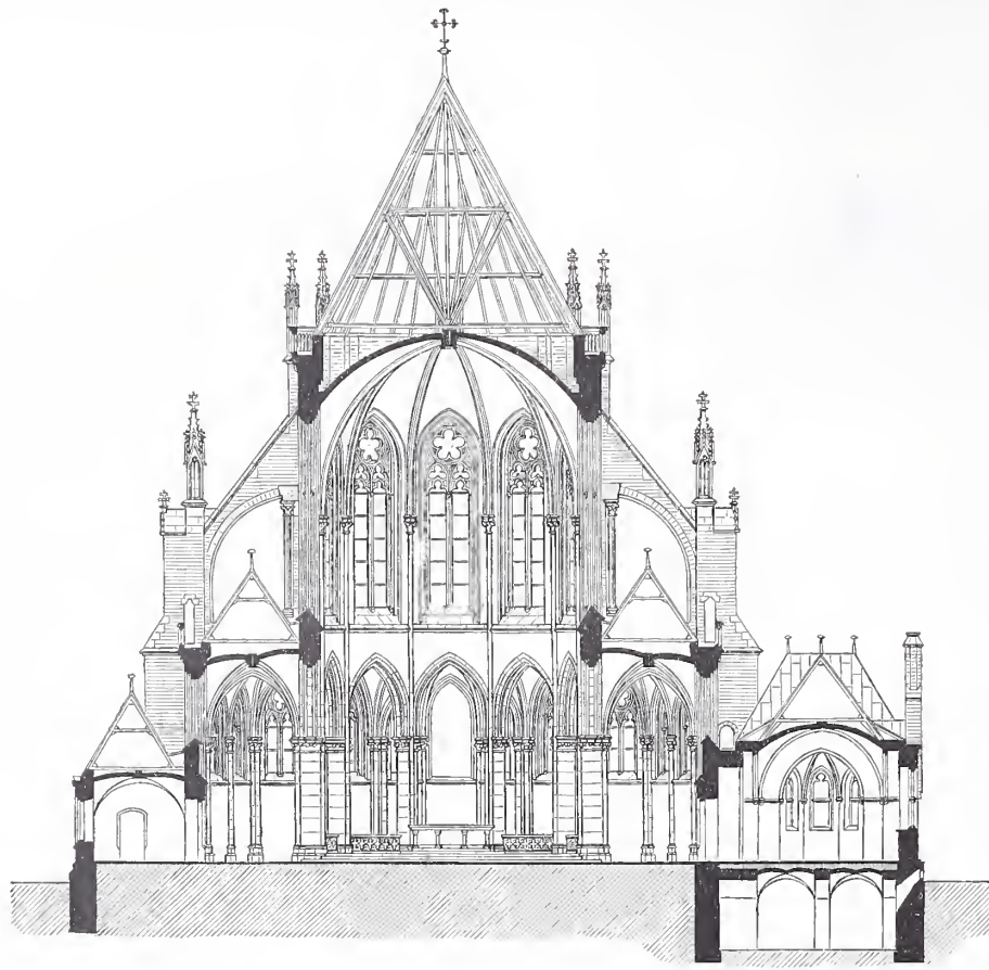
Schnitt AB.
