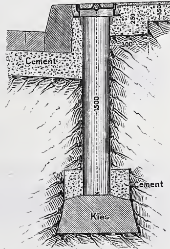
Querschnitt.
