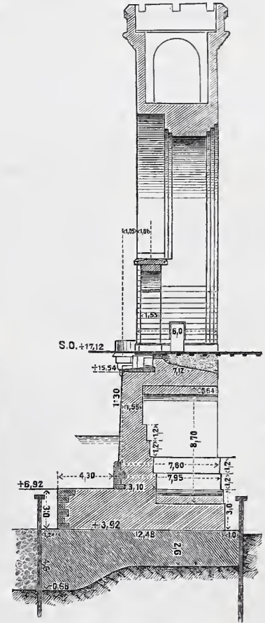
Abb. 9b. Schnitt durch einen Landpfeiler.
