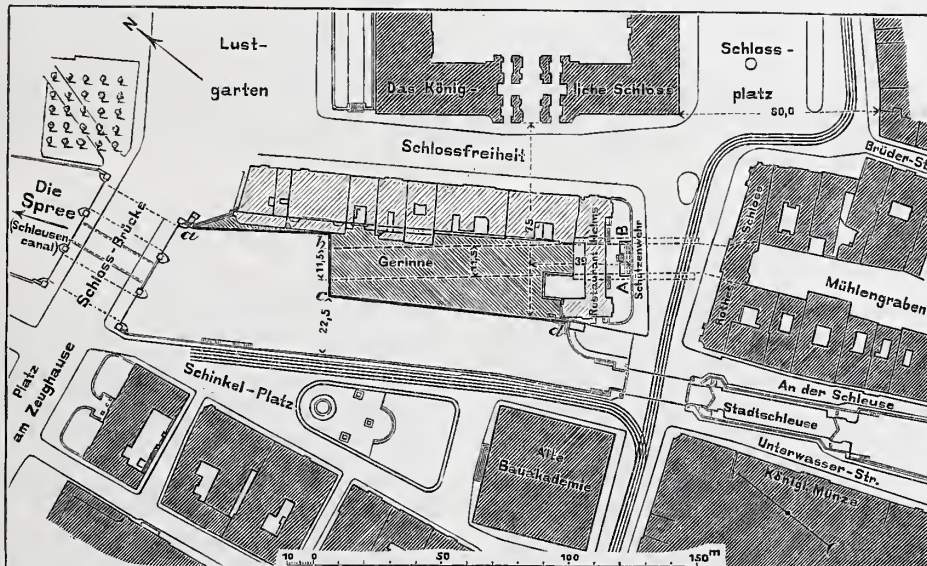
Lageplan. Nationaldenkmal für Kaiser Wilhelm I. in Berlin. (Zu der Mittheilung auf S. 242 der vorigen Nummer.)
