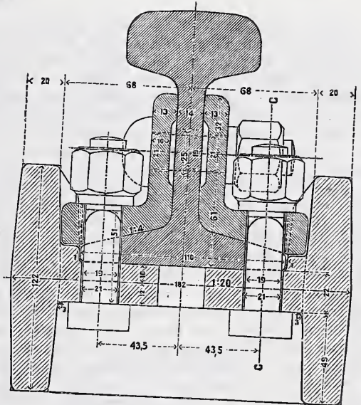
Abb. 4e. Querschnitt in der Mitte (a-a) (1/3 nat. Gröfse).
