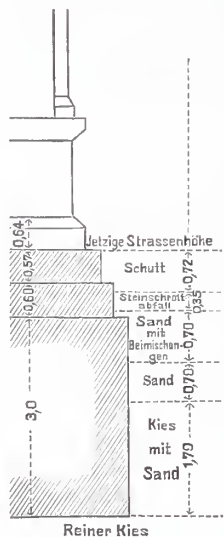
Abb. 1. Fundament des Römerthores.
