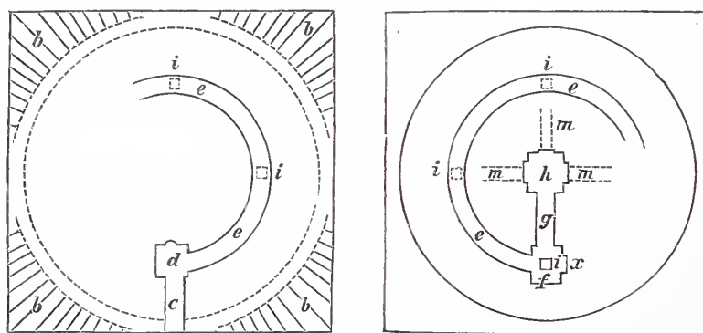
Abb. 1. Grabdenkmal des Kaisers Hadrian. Caninasche Wiederherstellung.
