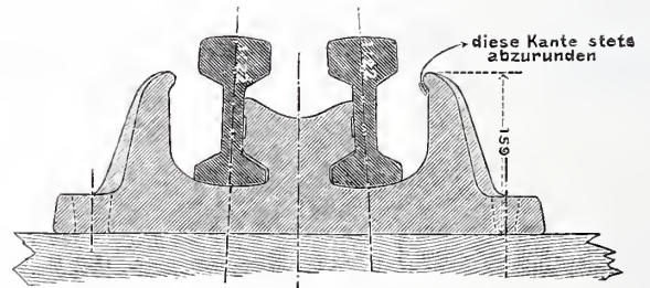
Abb. 9e. Schnitt durch Stuhl e.
