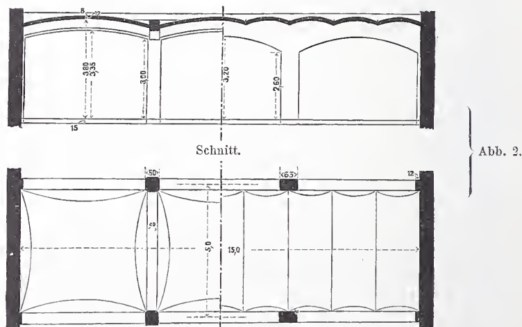
A. Pfeiler aus Klinkern in B. Gurtbogen, I-Träger Cement, Böhmisches Kappen. und preussische Kappen. Decke für eine Niederlage. Abb. 2.
