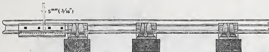
Abb. 3b. Längenschnitt des Geleises. Mafsstab 1:24.
