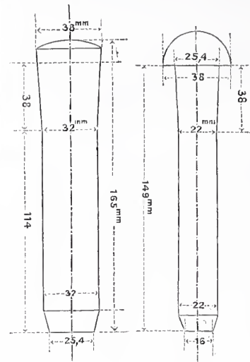
Abb. 4a. Holznagel. Abb. 4b. Eisennagel. Mafsstab 1:3.
