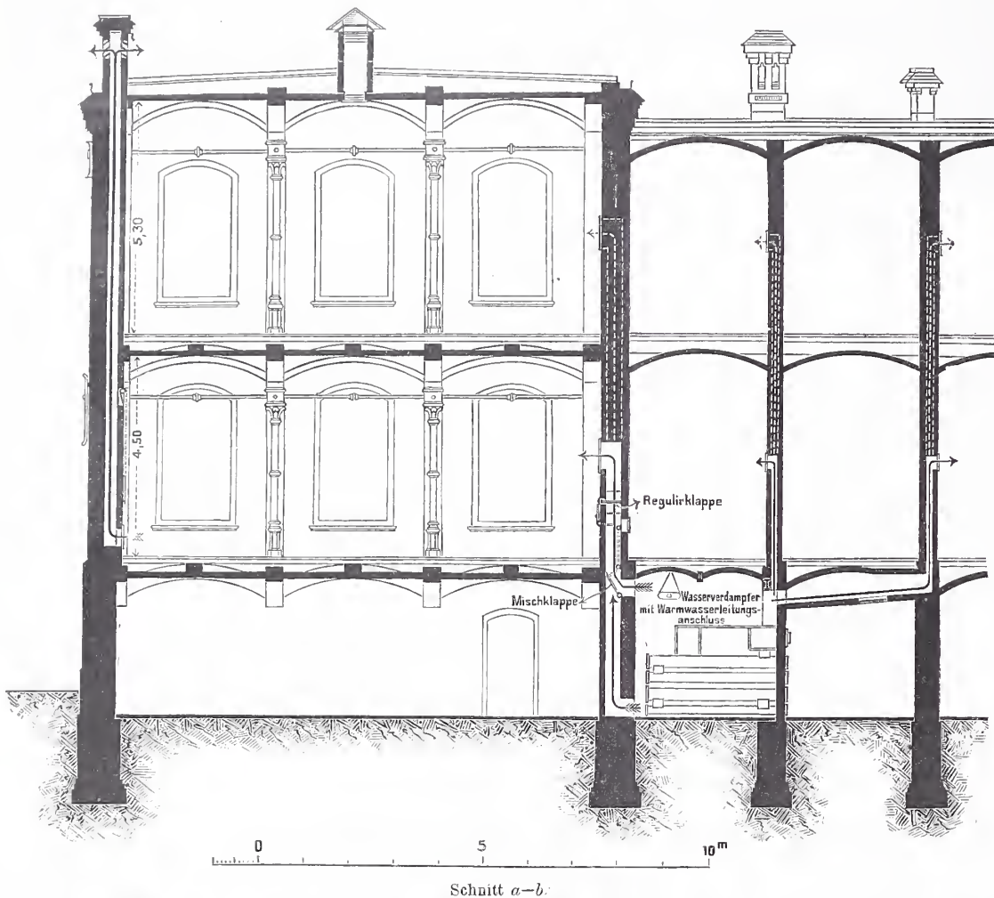
Schnitt a-b.
