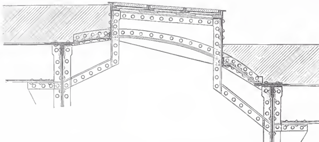
Abb. 18. Abdeckung mit Tonnenblech nebst Oberlicht. (Unterführung der Maybachstrafse).
