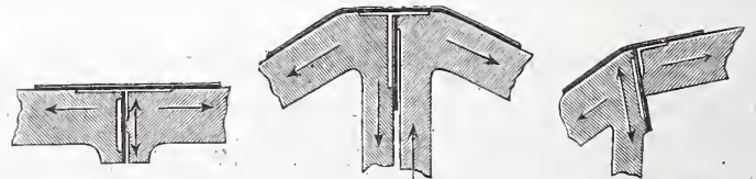
Abb. 13. Köpkes Federgelenke.
