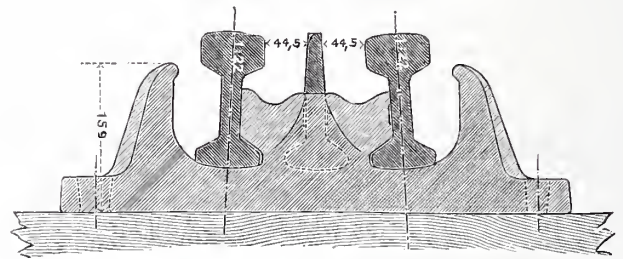
Abb. 9d. Schnitt durch Stuhl d.
