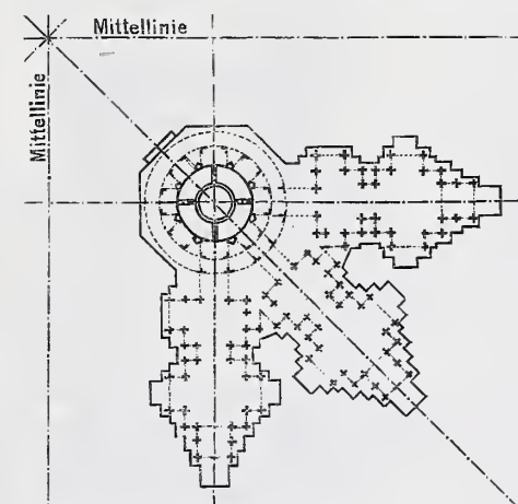
Abb. 4. Theil vom Grundrifs zu Abb. 3.
