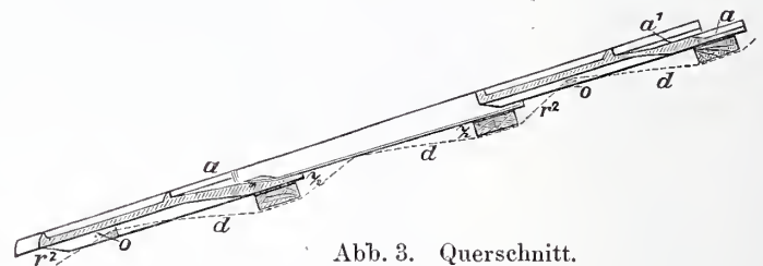
Abb. 3. Querschnitt.
