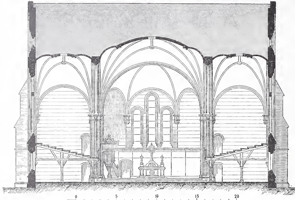
Querschnitt. Kirche in Eydtkuhnen.
