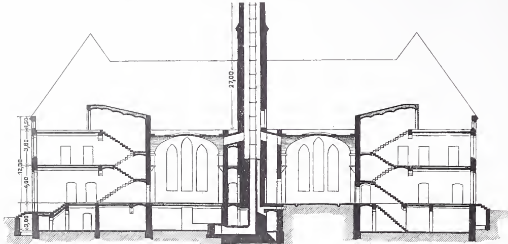
Längenschnitt.
