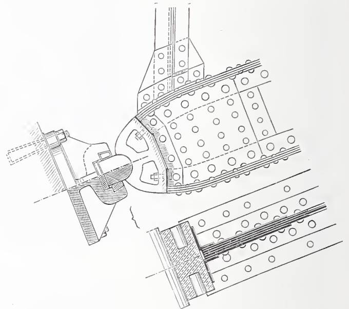
Abb. 13. Auflager des eisernen Ueberbaues der Venloer-Straßen-Unterführung.
