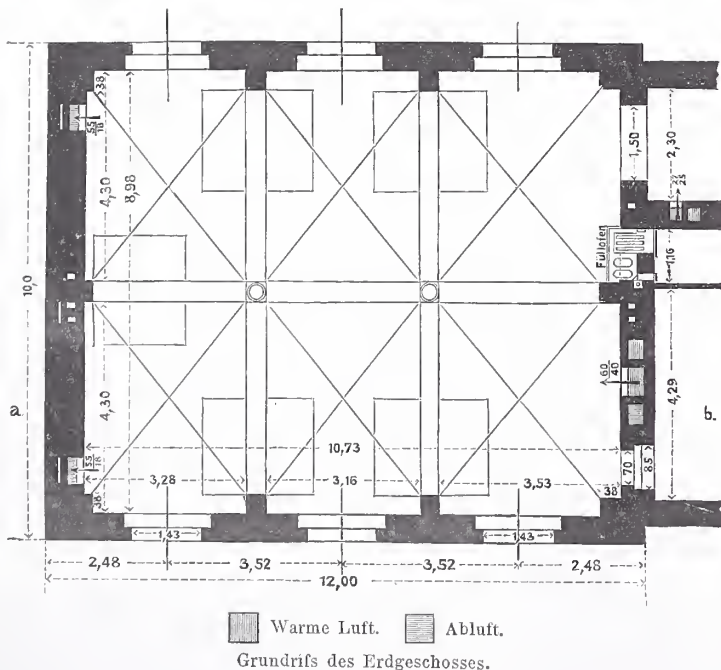
Abb. 12. Krankensaal der Frauenklinik in Breslau (Heizung u. Lüftung).
