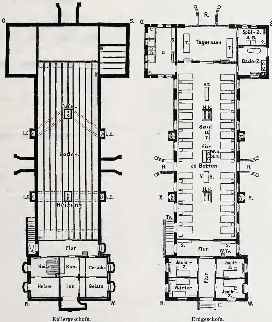
Abb. 14. Neues allgemeines Krankenhaus in Hamburg-Eppendorf. Grosser Krankenpavillon (Fußbodenheizung).
