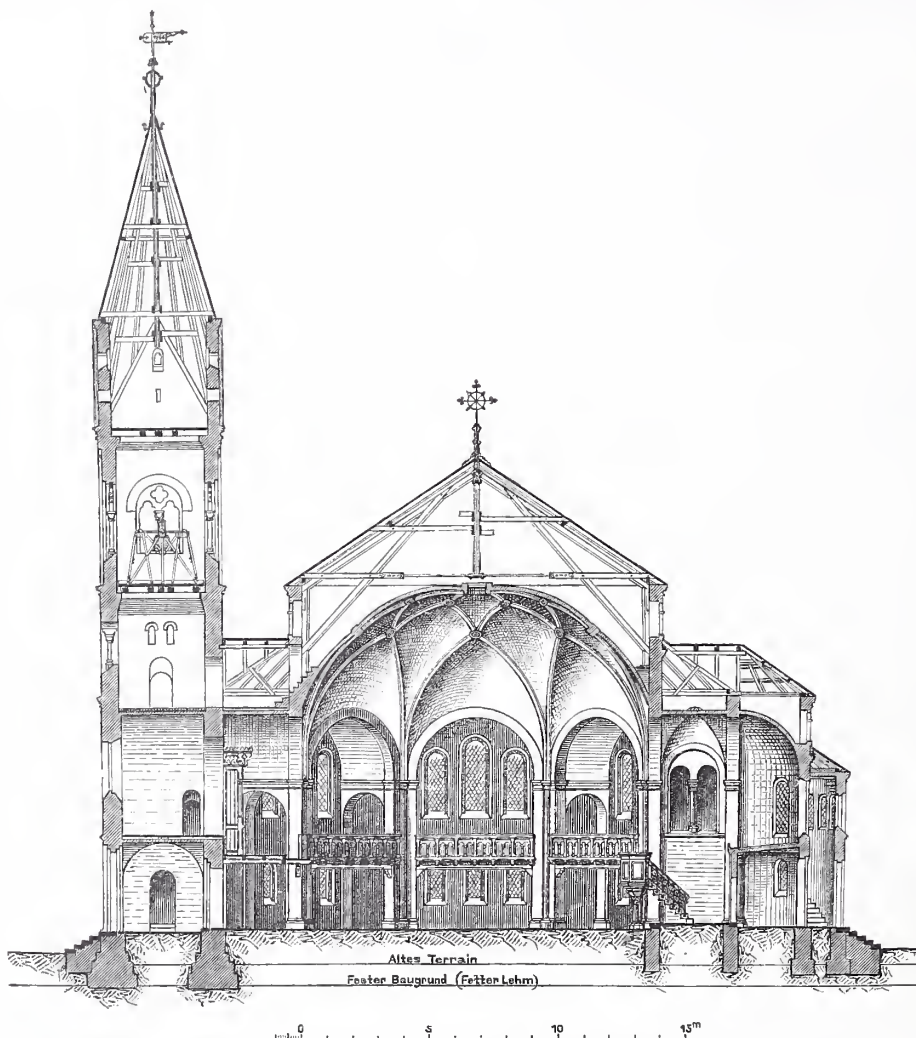
Längenschnitt.
