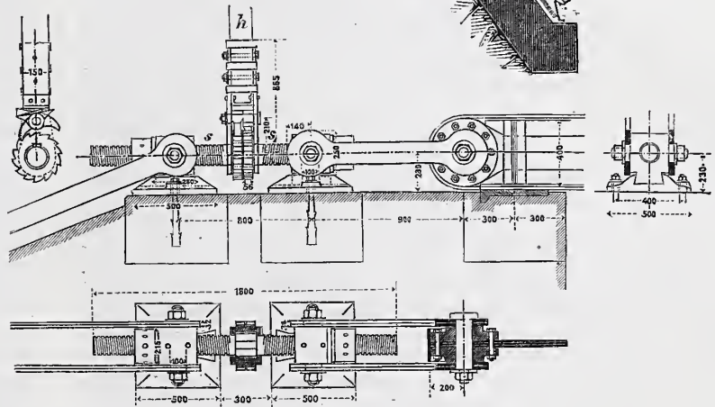
Abb. 4. Spannvorrichtung.
