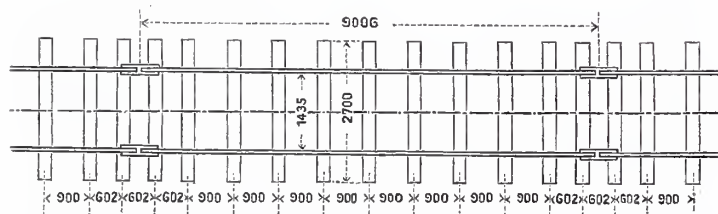
Abb. 2. Schwellentheilung.
