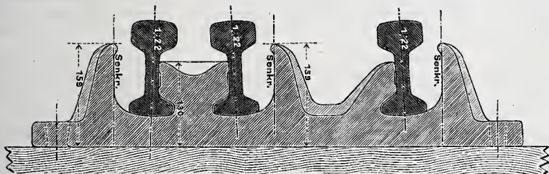
Abb. 10b. Querschnitt durch Stuhl A. Mafsstab 1:8.
