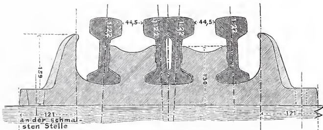
Abb. 9c. Schnitt durch Stuhl c.
