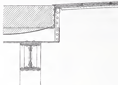
Abb. 19. Oberlicht-Anordnung bei der Unterführung der Mastrichter Strafse.
