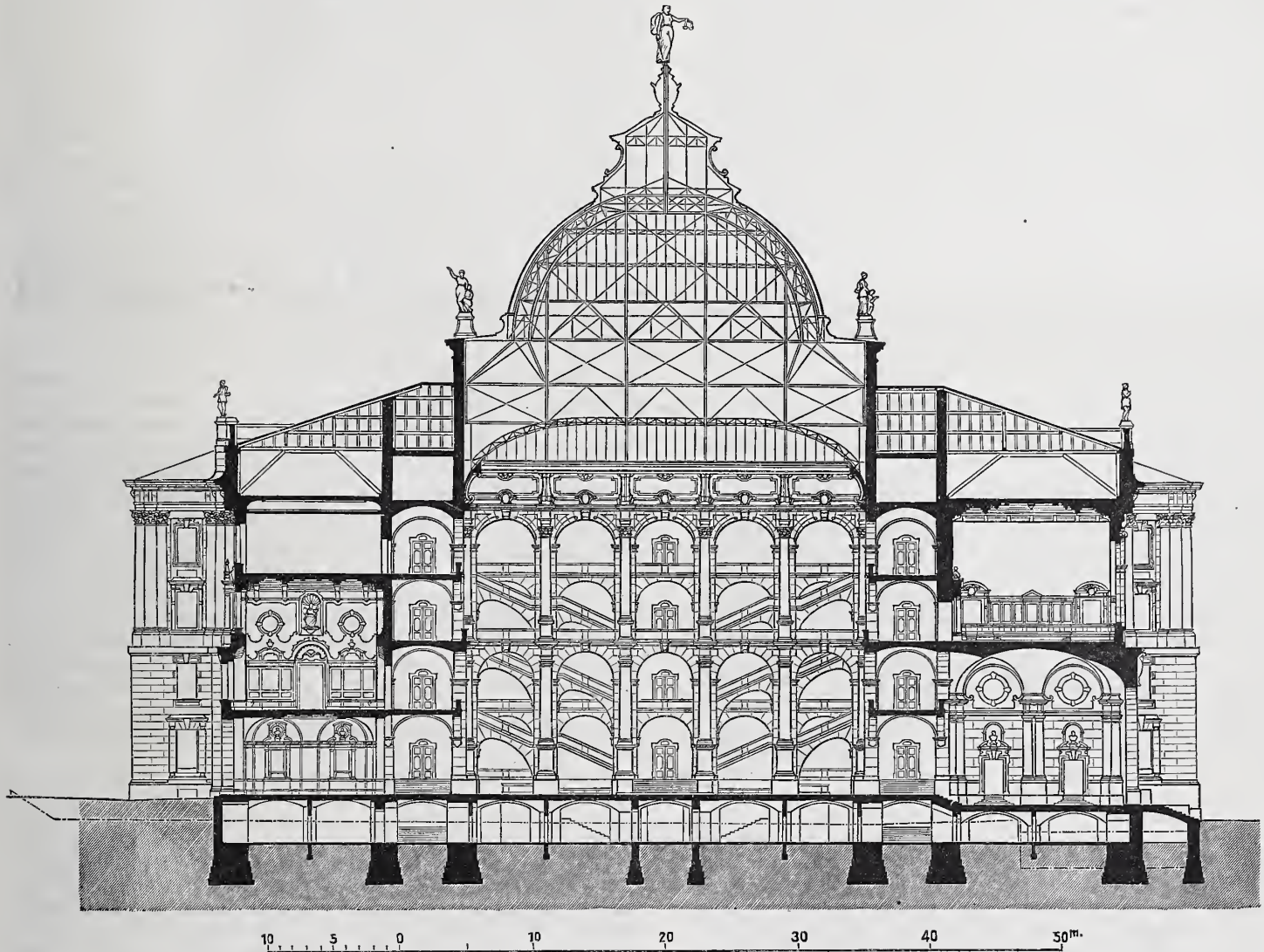
Abb. 3. Hauptquerschnitt.
