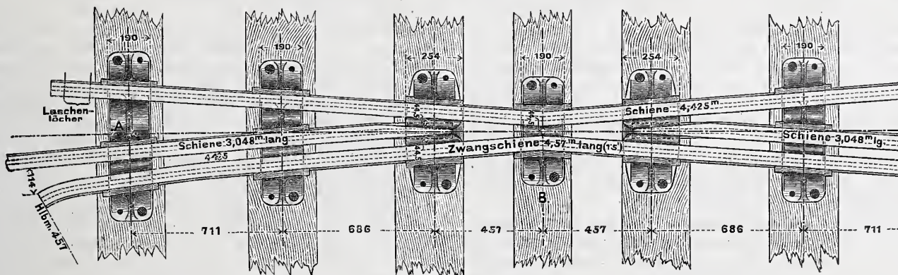
Abb. 10a. Grundrifs. Mafsstab 1:24.
