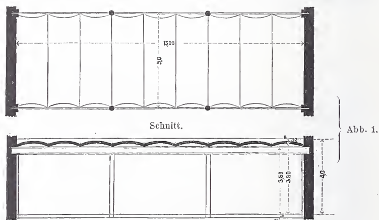
Gußeisernen Säulen, I-Träger und preussische Kappen. Abb. 1.
