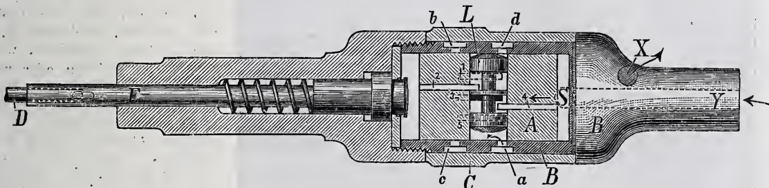
Abb. 1. Längenschnitt.
