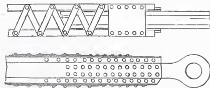
Abb. 6. Gurte und Glieder americanischer Brücken.
