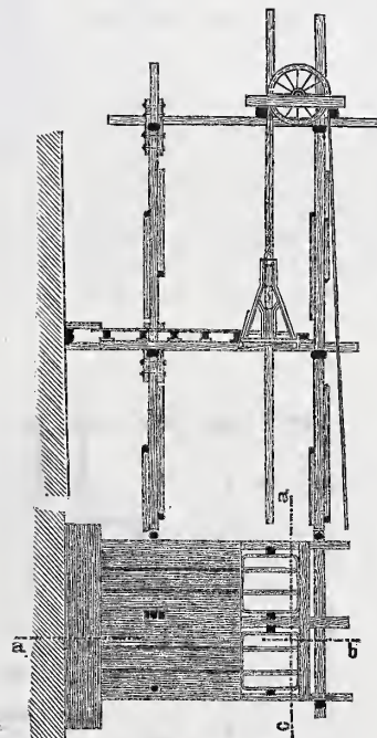
Abb. 14. Grundrifs und Schnitt a-b.
