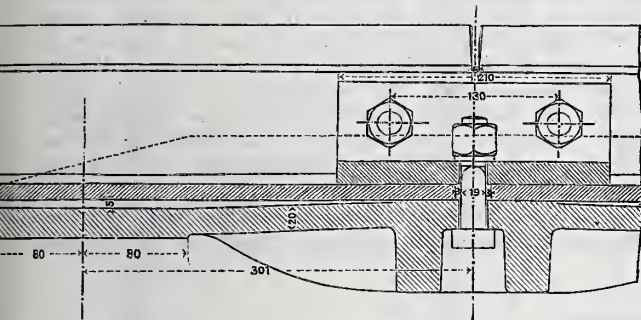
Abb. 4b. Längenschnitt durch die Brücke (c-c) (1/8 nat. Gröfse).
