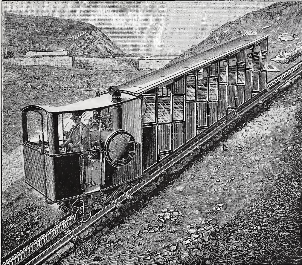
Abb. 1. Ansicht. Pilatusbahn.
