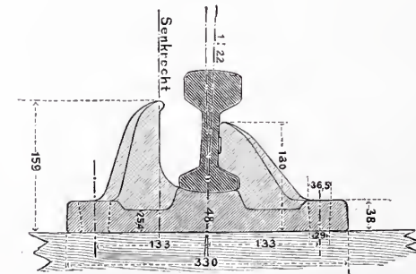
Abb. 9a. Schnitt durch Schiene und Stuhl. Mafsstab 1:8.
