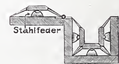
Abb. 6. Querschnitt.
