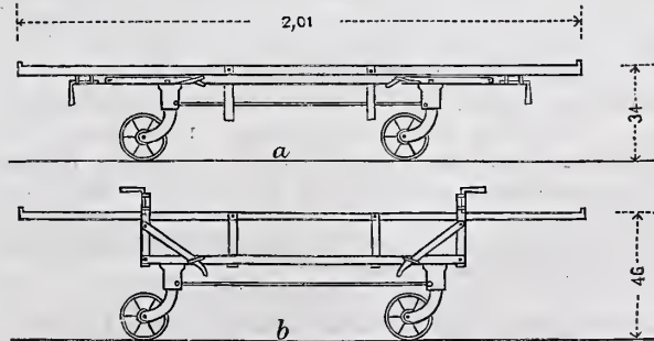
Abb. 36. Transportwagen für Krankenbetten.
