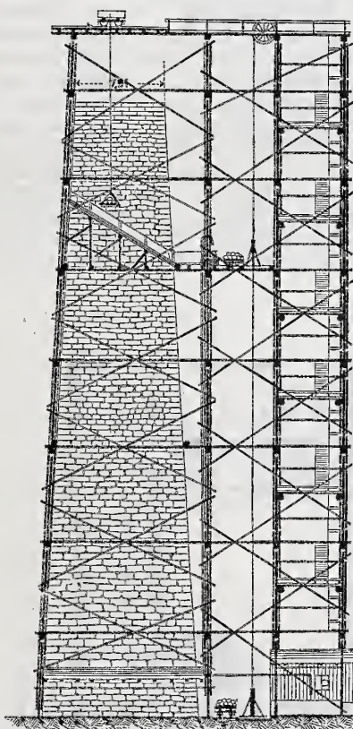
Abb. 13. Ansicht gegen die Moldau. Mauerungsgerüste.
