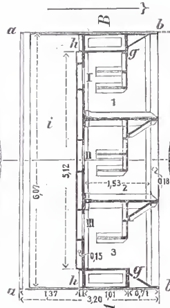
Abb. 4. Längenschnitt.
