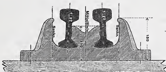
Abb. 10c. Querschnitt durch Stuhl B. Mafsstab 1:8.
