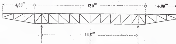
Abb. 2. Querträger.
