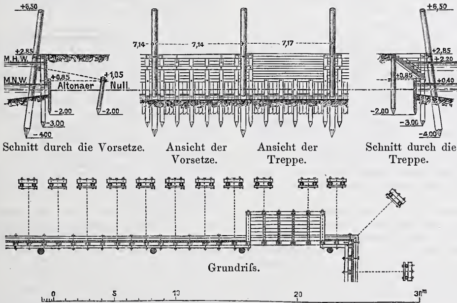
Abb. 5. Holz-Vorsetze des westlichen Hafens für Flussfahrzeuge. Hafenerweiterungsbauten der Stadt Altona.
