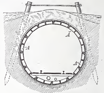
Querschnitt yy .
