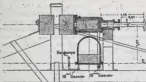
Abb. 4. Längenschnitt.
