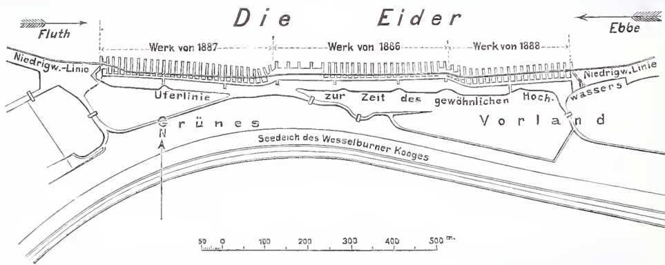
Abb. 2. Lageplan der Uferschutzwerke vor dem Wesselburener Kooge.
