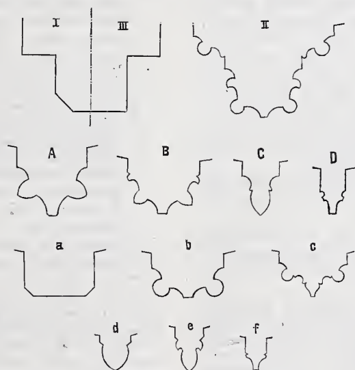
Abb. 2. Gurtbögen und Rippen der Gewölbe.
