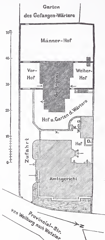
Abb. 1. Lageplan. Amtsgericht in Braunfels.
