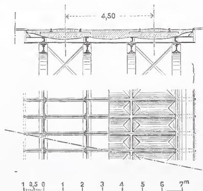
Abb. 14. Fahrbahn-Anordnung bei der Unterführung der Venloer Straße.
