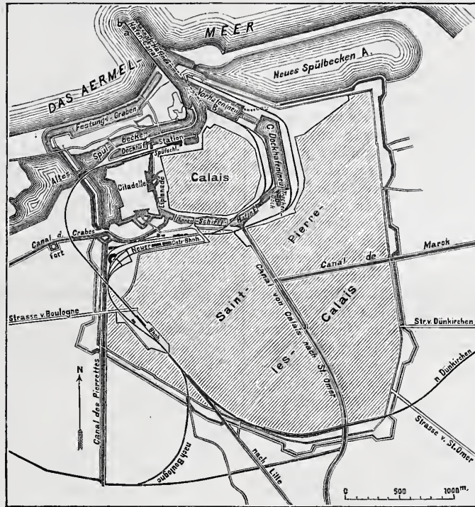
Abb. 1. Lageplan von Calais und Saint-Pierre-les-Calais.
