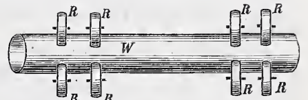
Abb. 5. Grundriss der Welle mit den Rollen.
