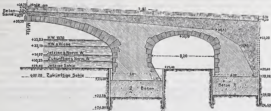
Längenschnitt.
