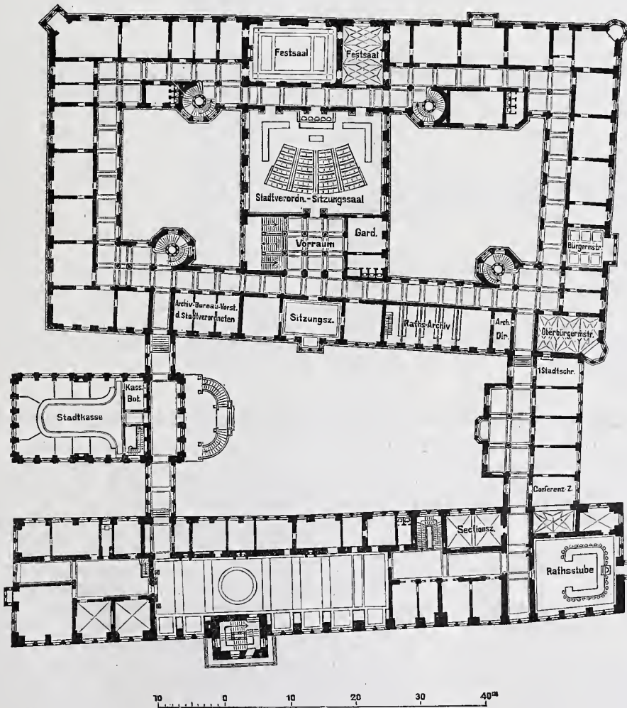
I. Stockwerk. Neubau des Rathhauses in Leipzig.
