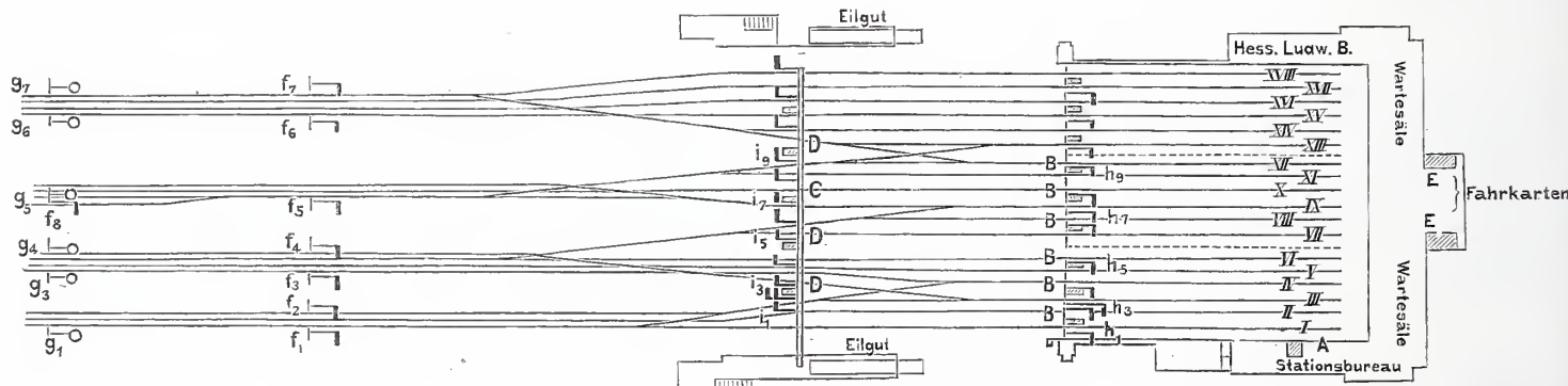
g = 6 Vorsignale. f = 7 Abschlussignale. fs = Abschlussignal für das Verbindungsgeleis. i = 11 einflügelige und 1 zweiflügeliges Ausfahrtsignal. h = 12 Wegesignale. C = Assistentenbude. D D D = Stellwerke. — (Die Nebengeleise sind weggelassen.)
