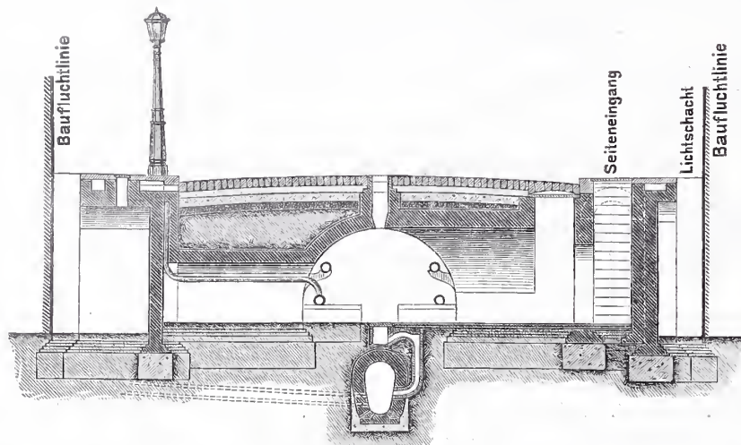
Querschnitt A-B.
