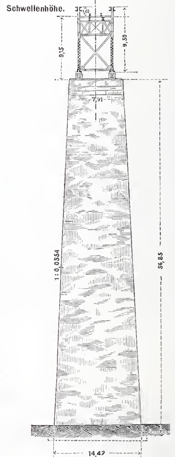
Abb. 10. Schnitt A-B.
