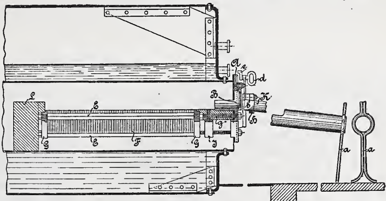
Abb. 2. Senkrechter Längenschnitt.
