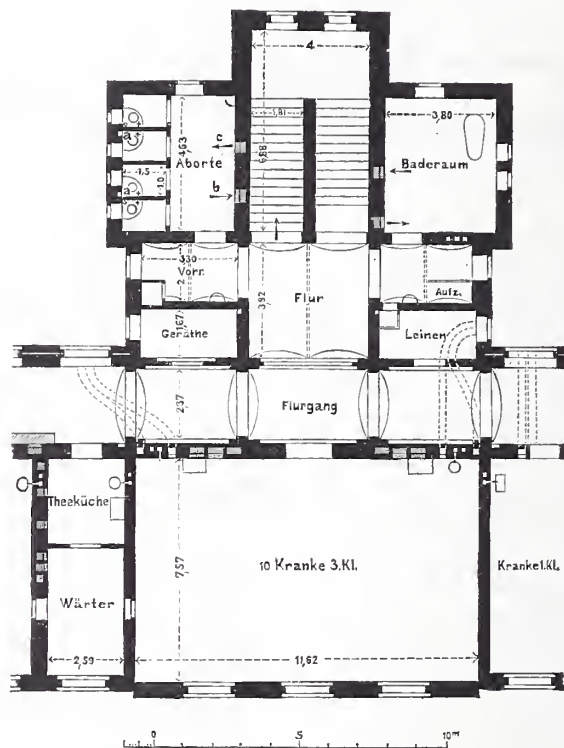
aa Entlüftung der Abortsitze. b Entlüftung des Abortraumes. c Zuführung warmer Luft.
