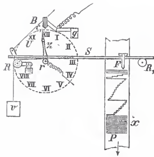
Abb. 2. Aufzeichnungswerk.
