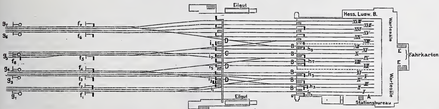
g = 6 Vorsignale. f = 7 Abschlufssignale. f 3 = Abschlufssignal für das Verbindungsgeleis. i = 11 einflüglige und 1 zweiflüglige Ausfahrtssignale. h = 12 Wegesignale. C = Assistentenbude. DDD = Stellwerke. — (Die Nebengeleise sind weggelassen.)
