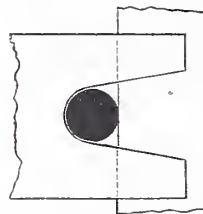
Abb. 6. Schnitt e-f.
