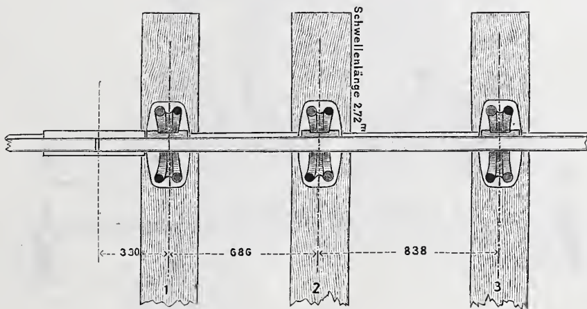
Abb. 3a. Grundriß des Geleises.
