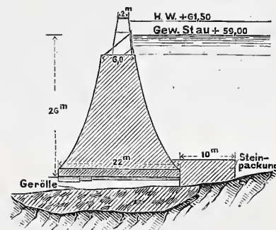
Abb. 5. Schnitt a—b.
