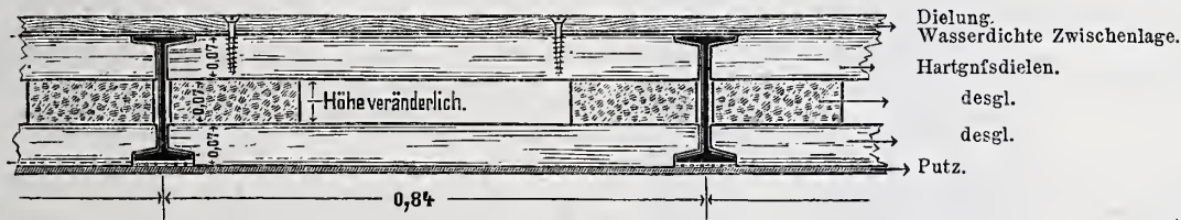
Abb. 1. I-Träger für 6 m Spannweite bei 300 kg/qm Nutzlast.
