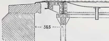
Abb. 16. Unterstützung des Schleppblechs durch Consolen am Endquerträger (Mastrichte Strafe).
