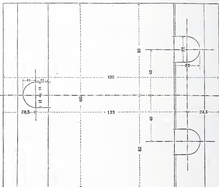
Abb. 3. Unterlagsplatte (1/2 nat. Gröfse).
