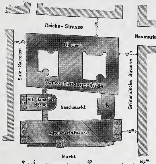
a. Lauben für die Bürgersteige. b. Säulenhallen, darüber Verbindungsgänge. c. Läden (Gewölbe). d. Thurm. Lageplan.
