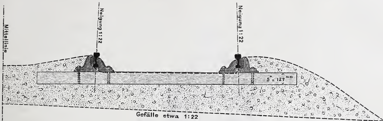
Abb. 2. Querschnitt des Geleises. Mafsstab 1:24.
