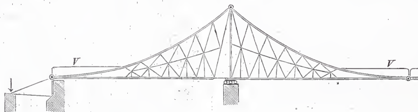
Abb. 12. Köpkes versteifte Hängebrücke.
