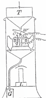
Abb. 1. Regenmesser.
