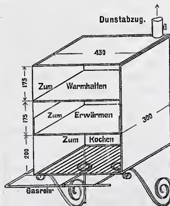
Abb. 28. Wärmeschrank mit Gaskocher.
