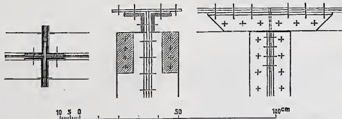
Wagerechter Schnitt. Querschnitt. Abb. 4. Abb. 5.
