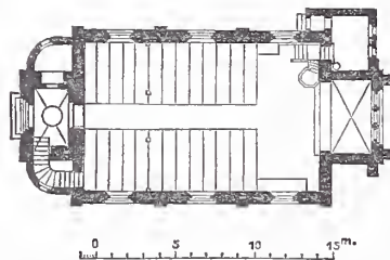
Grundriß.
