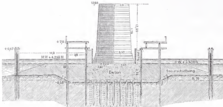
Abb. 9b. Schnitt.
