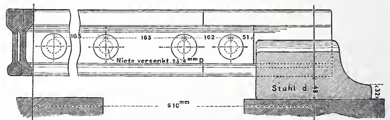
Abb. 9f. Längenschnitt und Ansicht der Herzstückspitze.
