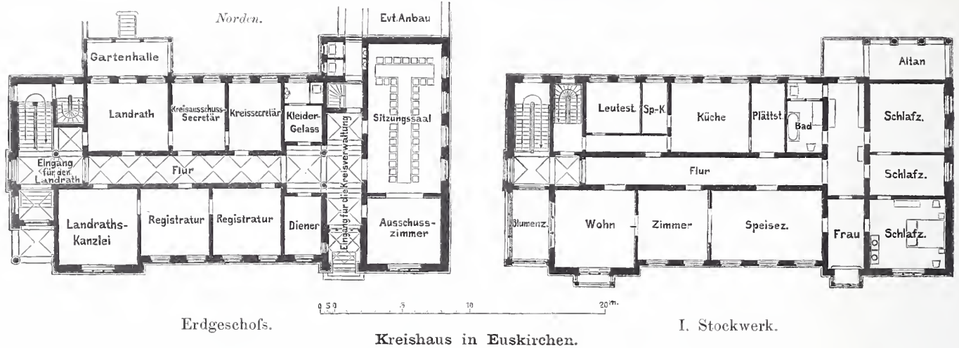
Kreishaus in Euskirchen.
