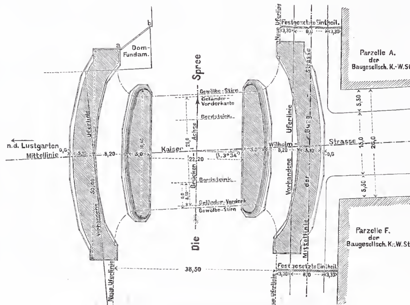
Grundriß der Kaiser Wilhelmbrücke in Berlin.
