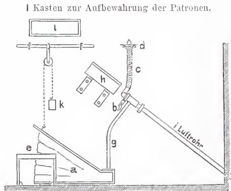
Abb. 3. Ansicht.
