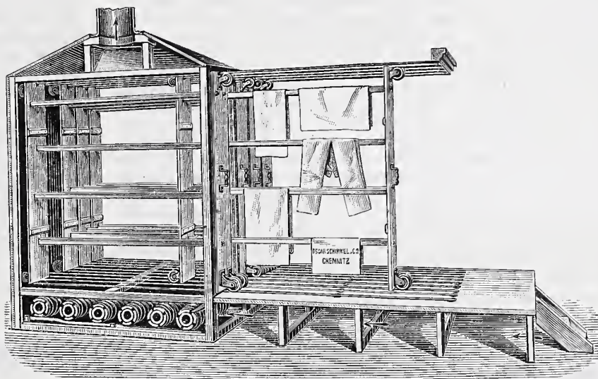
Abb. 26. Wäschetrocknenapparat mit Ausziehschiebern (Coulissen).
