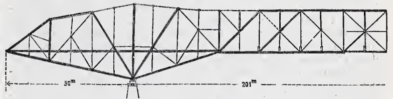
Abb. 14. Colorado-Brücke.
