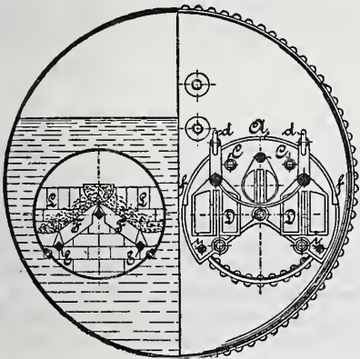
Querschnitt mit eingeschobener Kohlschaufel. Vorderansicht. Abb. 1.
