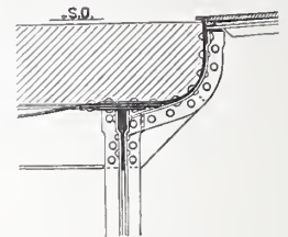
Abb. 20. Anordnung des Oberlichts bei der Unterführung der Gladbacher Strafse.
