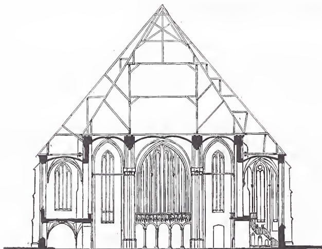
Abb. 1. Querschnitt.
