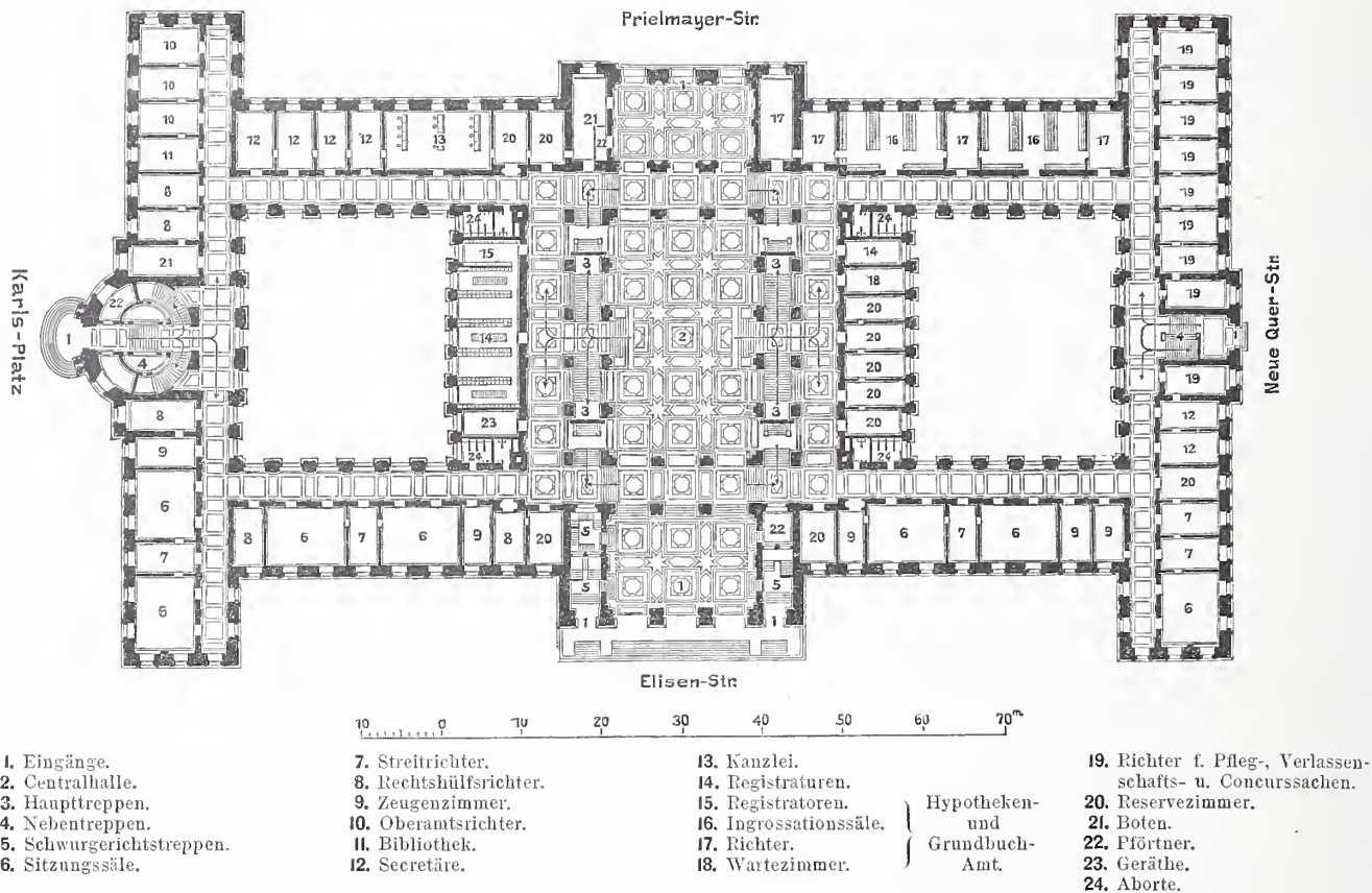
Abb. 2. Erdgeschoss. (K. Amtsgericht München I., Abth. A. f. Civilsachen.) II. Bauentwurf für das neue Justizgebäude in München.
