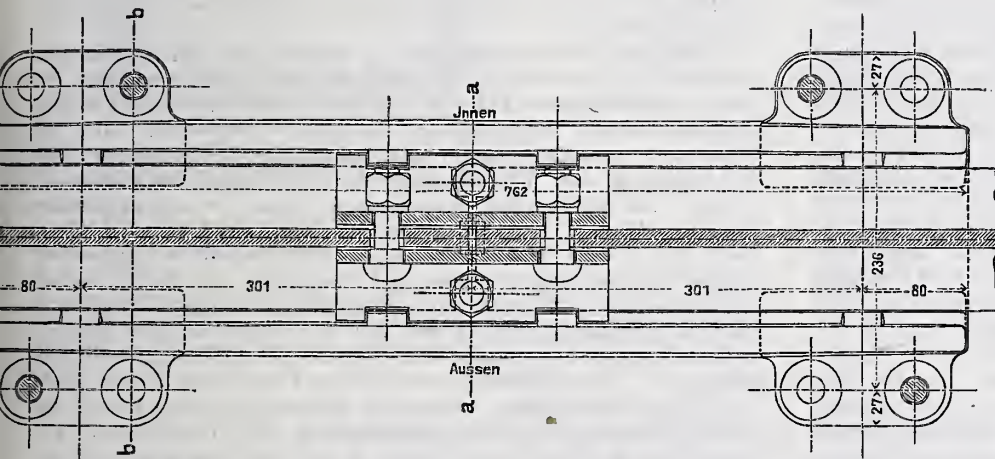
Abb. 4c. Grundriß der Brücke (1/8 nat. Gröfse).
