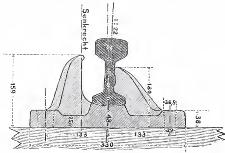
Abb. 9a. Schnitt durch Stuhl a.
