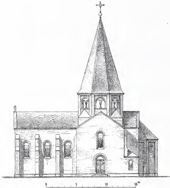
Stüdfrent der Kirche.
