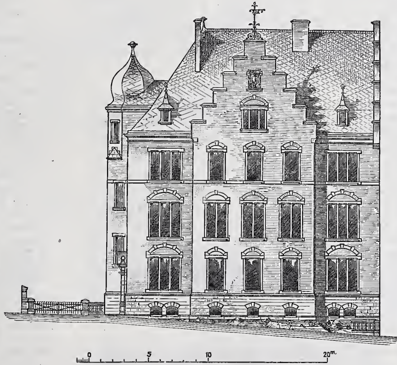
Abb 2. Ost-Ansicht.
