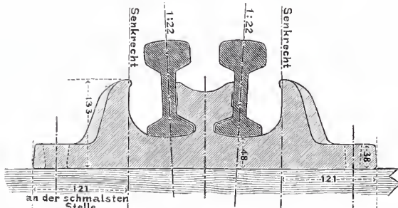
Abb. 9b. Schnitt durch Stuhl b.
