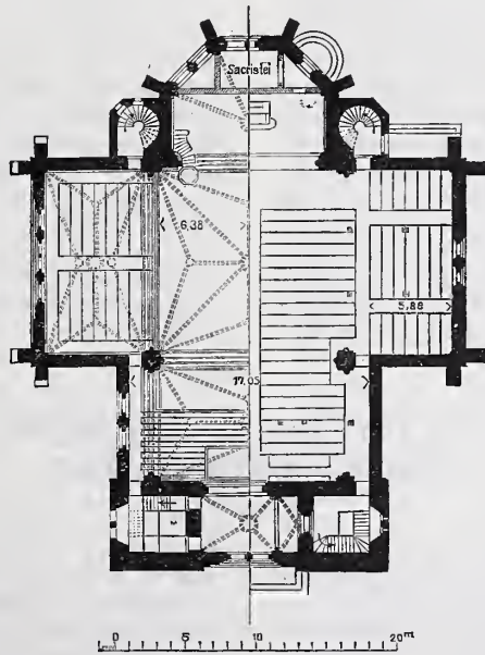
Grundriss
