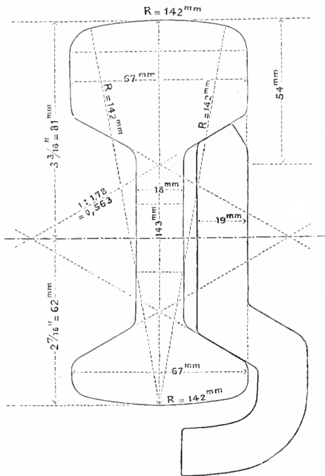
Abb. 1. Querschnitt der Schiene mit Lasche. Mafsstab 1:2.
