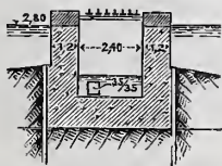
Abb. 3. Querschnitt.
