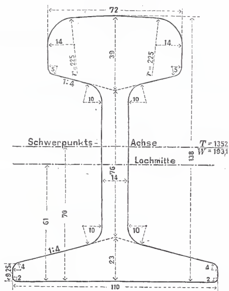
Abb. 1. Schienen-Querschnitt (1/2 nat. Gröfse).
