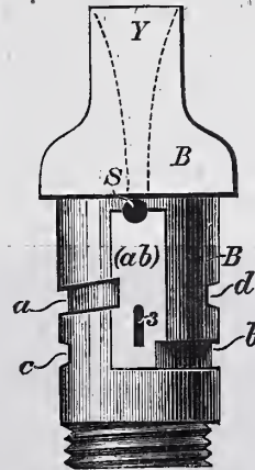
Abb. 4. Ansicht der Einströmungsseite des Cylinders B .
