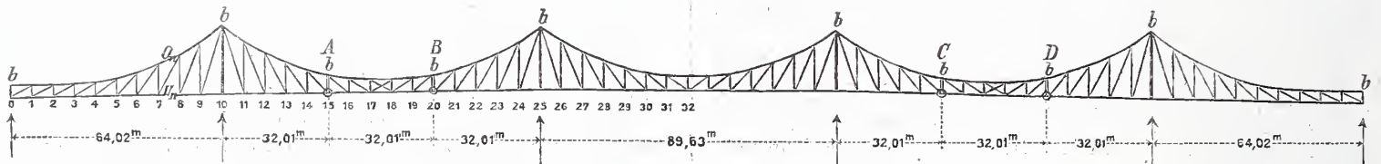
Abb. 3. Hauptträger.
