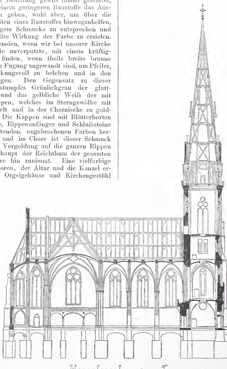
Abb. 2. Längenschnitt.
