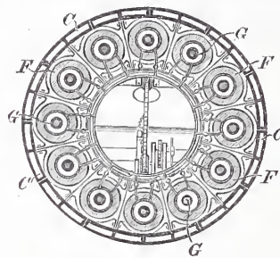
Querschnitt xx .
