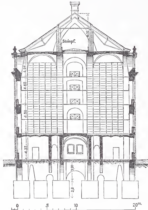
Querschnitt.
