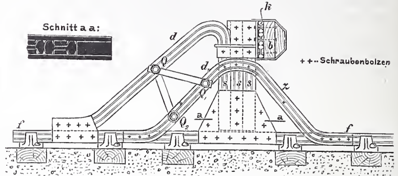
Englischer Prellbock.
