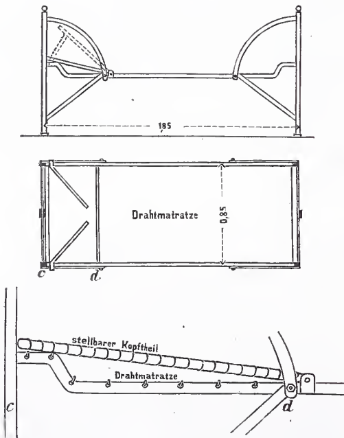
Abb. 29. Bettstelle mit Drahtgeflecht und beweglichem Kopftheile.
