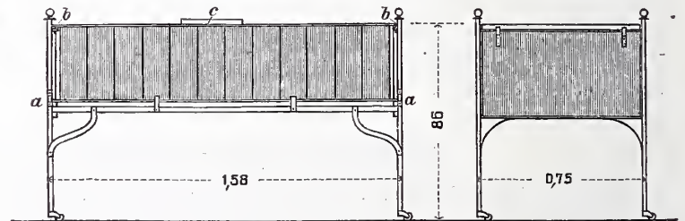
Abb. 31. Kinderbettstelle.
