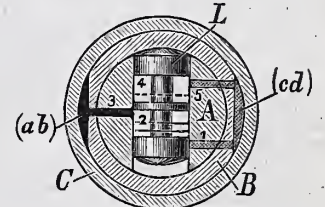
Abb. 3. Querschnitt.
