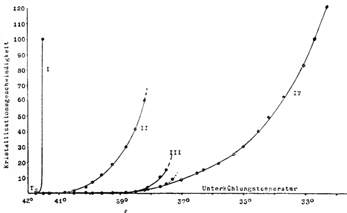
Fig. 5. Abhängigkeit der Kristallisationsgeschwindigkeit (in Teilstrichen = 0,017 mm/min) von der Unterkühlungstemperatur für verschiedene Flächenarten eines Salokristalls.
