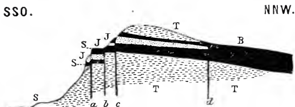
Fig. 2. Profil durch die Schichten von Gröf. B = Basalt; T = vulkanischer Tuff; J = Jökullhlaupsediment (Vulkanoglazial); S = Schifflflächen; a, b, c, d Verwerfungsspalten.
