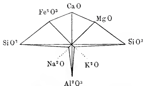
Fig. 6. Melaphyr von Palle rabbiose (DOELTER analys.) 1 .
