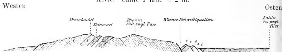
Fig. 1. Querprofil durch die Dharan-Antiklinale am Nordende der Lakki-Kette. Skale 1 mile = 2 m.
