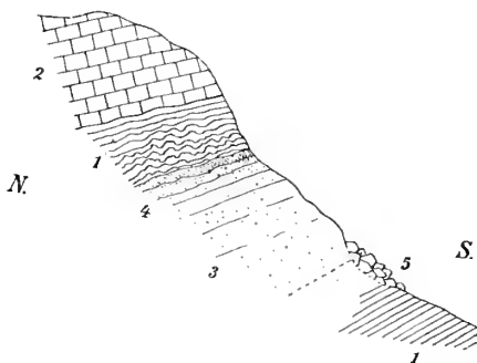
Fig. 1. Profil durch den Quarzporphyr- und Phyllitkontakt im Stojičevac dol auf der Südseite des Vratnica-Gebirges. 1 Karbonischer Phyllit. 2 Permian-karbonischer Kalkstein. 3 Quarzporphyr. 4 Derselbe in felsitischer Ausbildung. 5 Quarzporphyrschutt.
