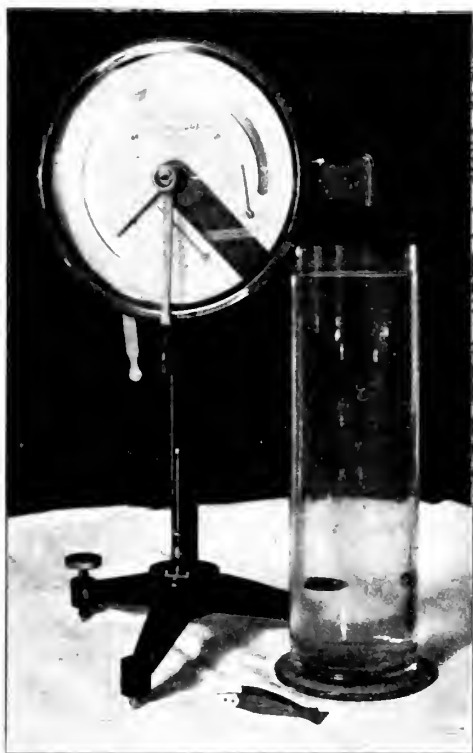
Fig. 6. Torsionswage für 150 Milligramm.
