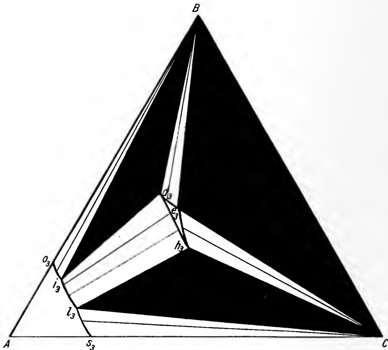
Fig. 7. Isothermendigramm für das ternäre Raummodell (konstanter Druck P) für die konstante Temperatur T_3 .
