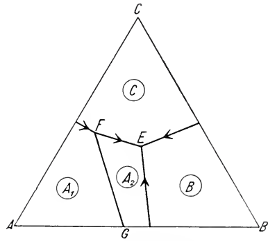
Fig. 5. Zu Modell 2.
