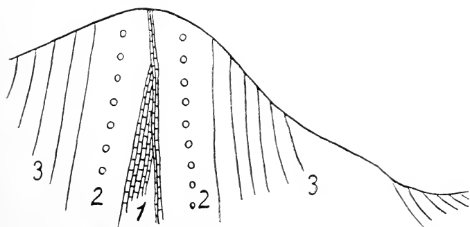
Fig. 1. Das Mittelmiocän bei Görgény-Sóakna. (Skizze.) 1. Schotteriger, fester Mergel. 2. (A-Horizont). 3. Grauer Tegel. (Mezősége-Schichten?) B-Horizont.
