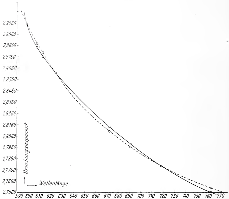
Fig. 2. Dispersion des ordentlichen Strahles des Zinnobers.
