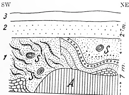
Fig. 5. Abgleitung (?) im Obermiocän bei Lövér.
