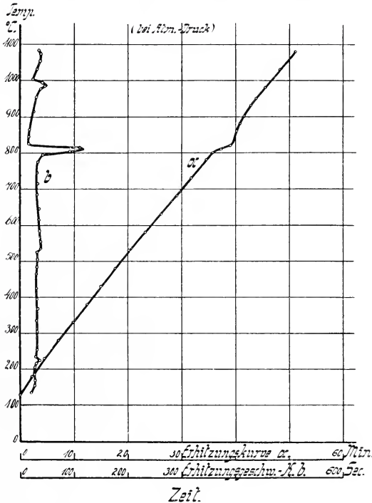
Fig. 13. Witherit, Fundort unbekannt.
