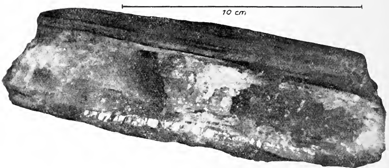
Fig. 4. Derselbe Block im Querbruch. Man beachte die Auswalzung der Steinsalzkrystalle.
