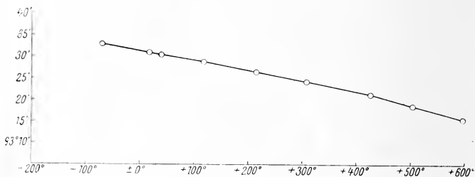
Fig. 9. Änderung des Winkels (001):(0\bar{1}0) bei Labradorit.
