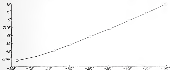
Fig. 2. Winkeländerung des Dolomitrhomboeders {1011} im Temperaturintervall von -170^{\circ} C bis 590^{\circ} C.
