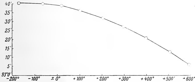
Fig. 5. Änderung des Winkels (001):(010) bei Albit. Kristall 1.
