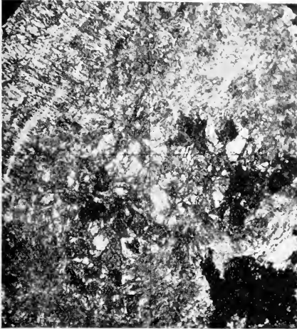
Fig. 7. Salit, Nephrit, Serpentin. Vergr. 61:1. +N.
