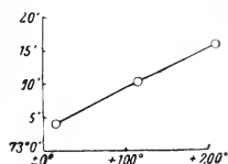
Fig. 4. Winkeländerung des Manganspatrhomboeders {1011} im Temperaturintervall von 16° C bis 212° C.
