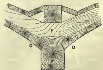
G, G, garboard-strakes; F, frame; K, keel.
