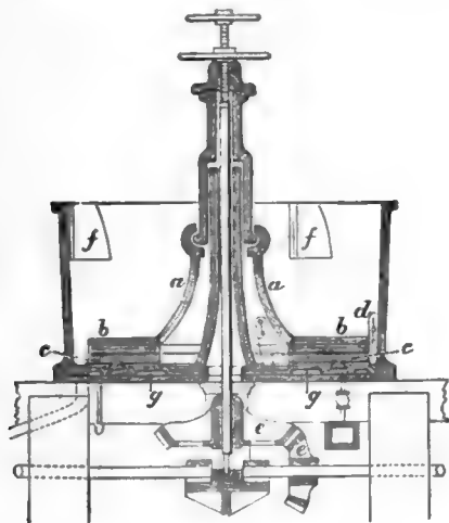
Fig. 1.—Amalgamating Pan :
