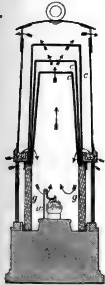
Fig. 2.—Marsaut Lamp.
