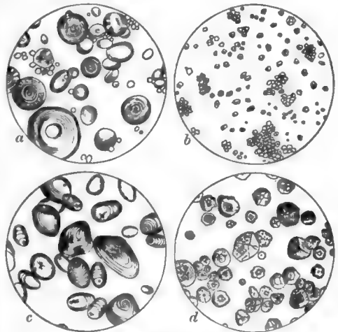
Starch Granules :
