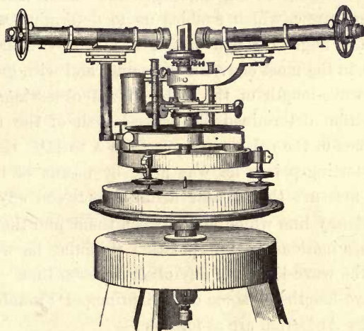
FIG. 34.—Ångström's spectrometer.
