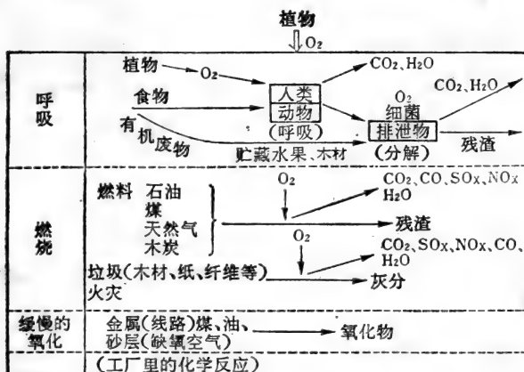
图 3.2 氧气的消耗
