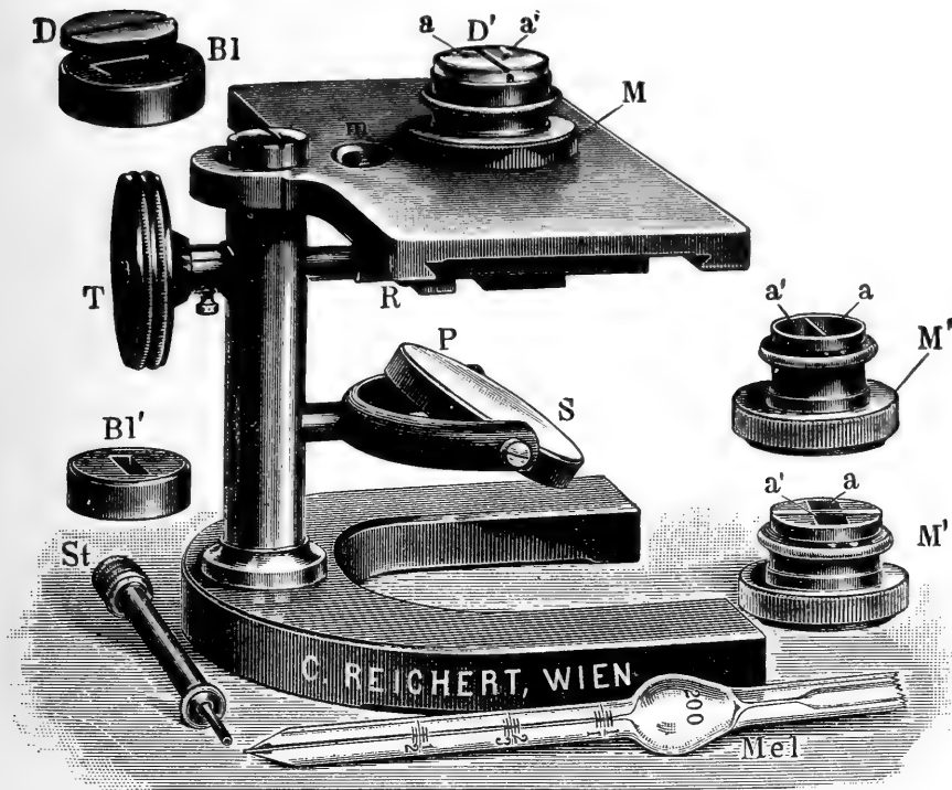
FIG. 9. Fleischl-Miescher hemometer.
