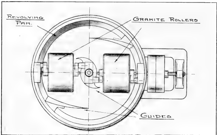
PLAN OF CHOCOLATE MELANGEUR.
