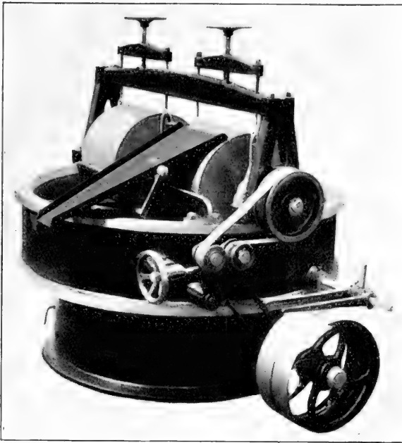
CHOCOLATE MELANGEUR.
