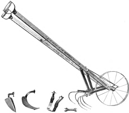
Fig. 1—Hawkeye Jr. Garden Raiser (PATENTED)
