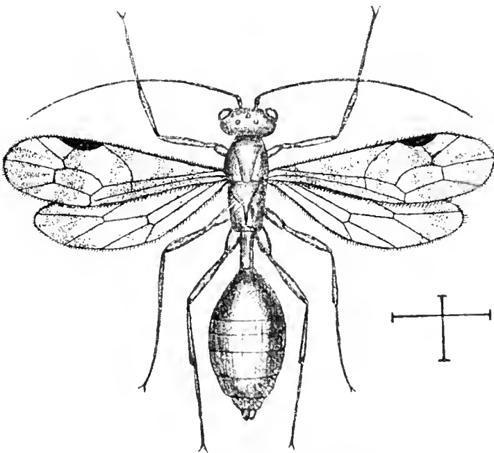
Fig. 47. Agriotypus armatus ♂.
