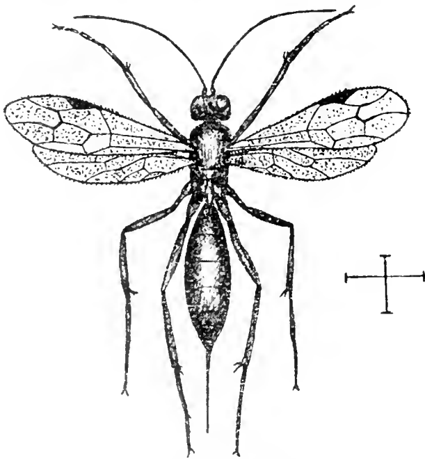
Fig. 49. Hemiteles biannulatus ♀.
