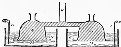
FIG. 27. Bell apparatus. (H. Bechhold.)
