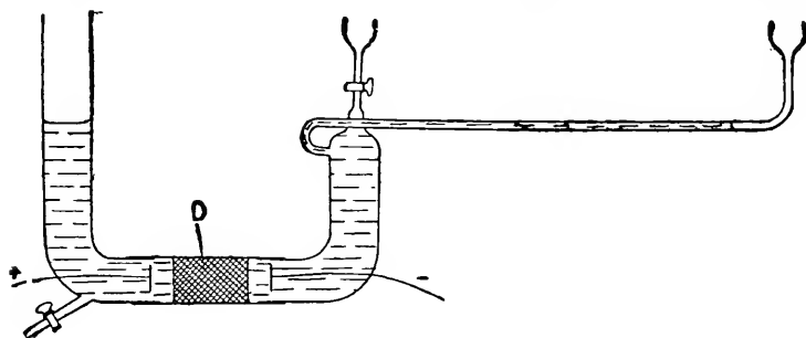
FIG. 8. Apparatus for electro-endosmosis. (H. Freundlich.)
