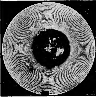
FIG. 50. Liesegang's rings. (From R. Liesegang.)
