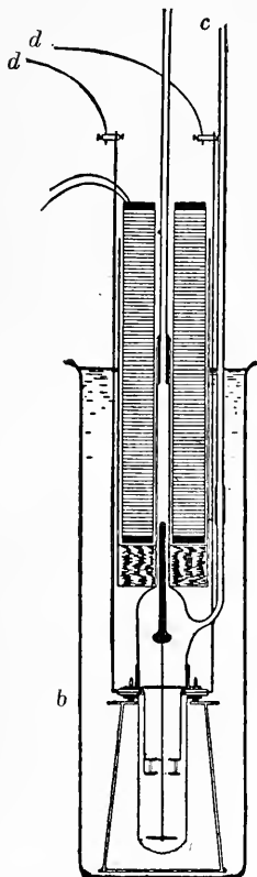
FIG. 22. Osmometer of Biltz and Von Vegesack.
