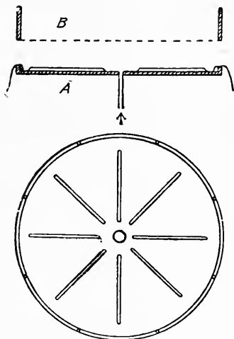
FIG. 13. Star dialyzer. (R. Zsigmondy.)
