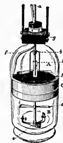
FIG. 21a. Dabrowski's diffusion apparatus.
