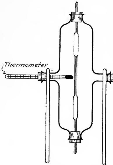
FIG. 24. Viscosimeter. (H. A. Determan.)
