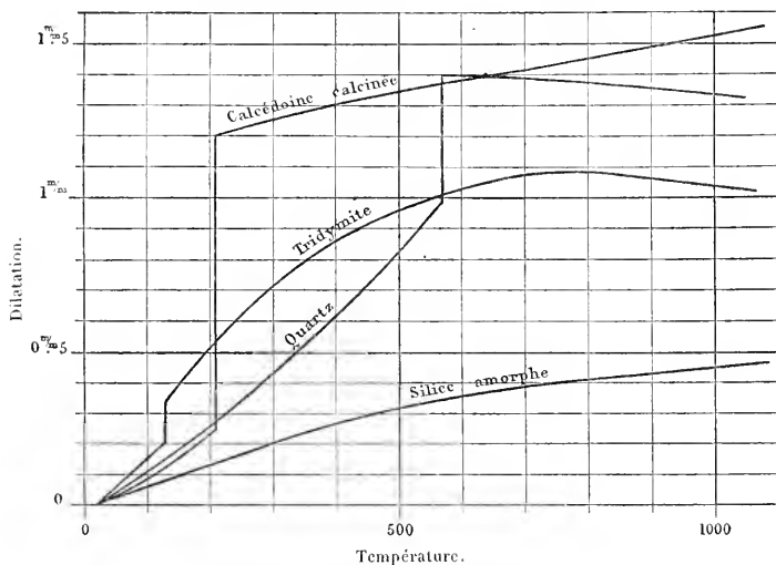
Dilatation des différentes variétés de silice.
