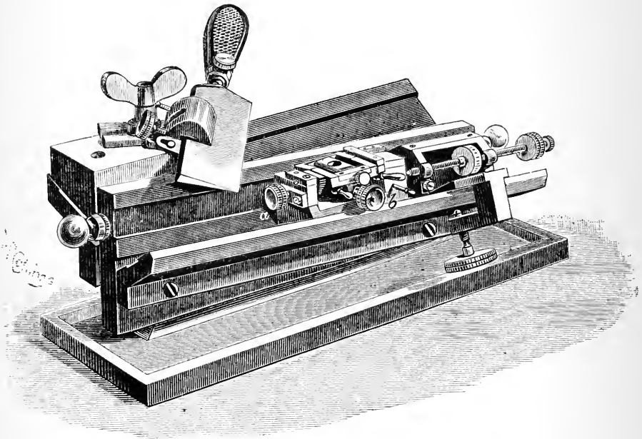
FIG. 45.—Thoma's microtome.
