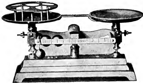
Fig. 37.—Cream scales.
