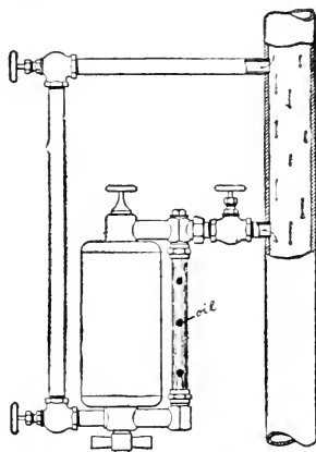
Fig. 84.—Lubricator.
