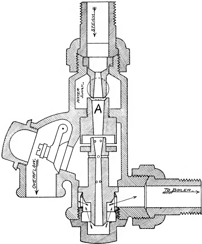
Fig. 78.—Injector.
