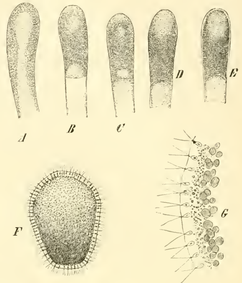
Fig. 251. Vaucheria sessilis . A , B Anlage der Sporangien. C , D , E Ausbildung der Schwärmersporen. Vergr. 95. F Schwärmerspore. Vergr. 25. G ein Stück der äusseren farblosen Plasmaschicht, dem vorderen Ende der Schwärmerspore entnommen. Vergr. 950.
