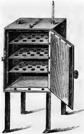
FIG. 9.—HOT-AIR STERILISER.
