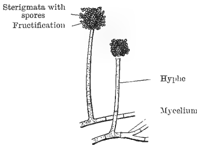
FIG. 3.— ASPERGILLUS GLAUCUS .
