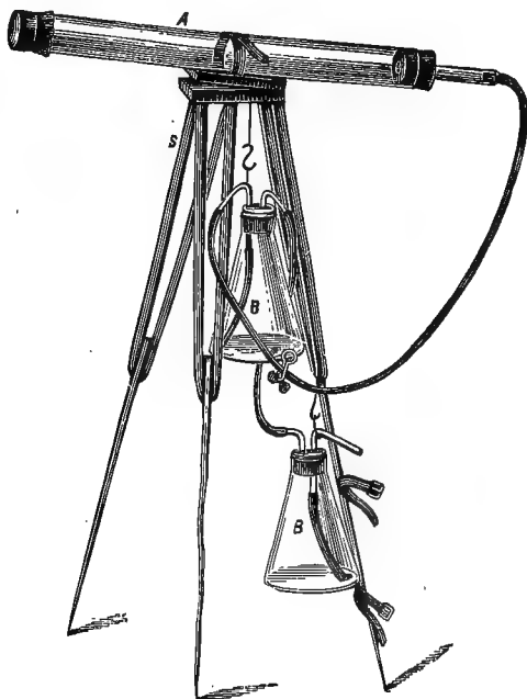
FIG. 38.—HESSE'S APPARATUS.
