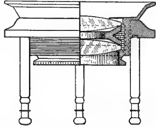
FIG. 201. TRIPOD MAGNIFIER.
