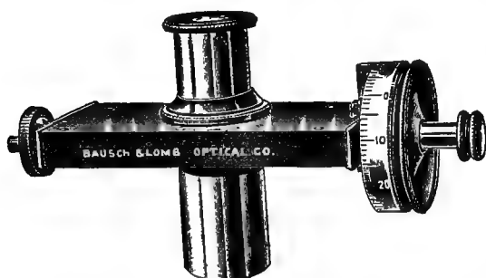
FIG. 93. FILAR MICROMETER OCULAR.
