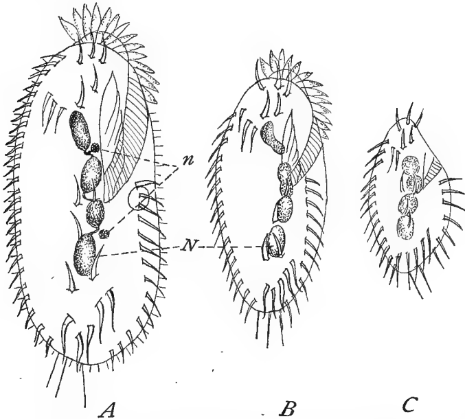
Fig. 29. — Onychodromus grandis Stein. [MAUPAS.]
