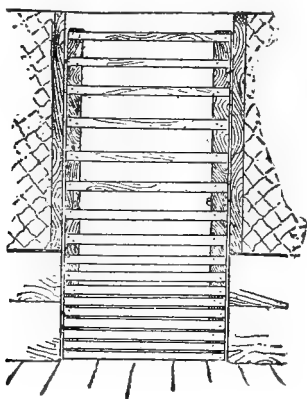
FIG 55: COMBINATION DOOR
