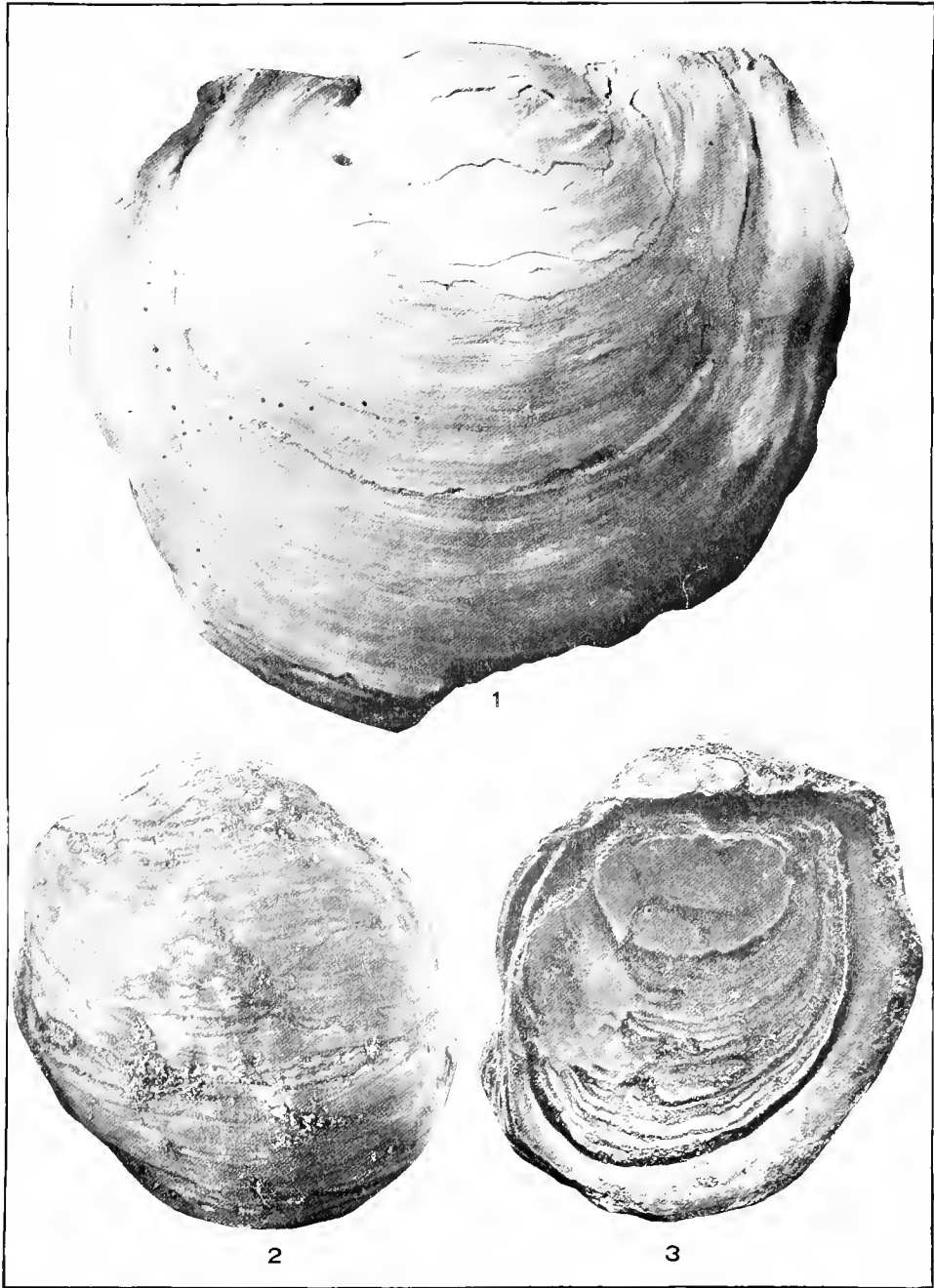
PELECYPODA.
