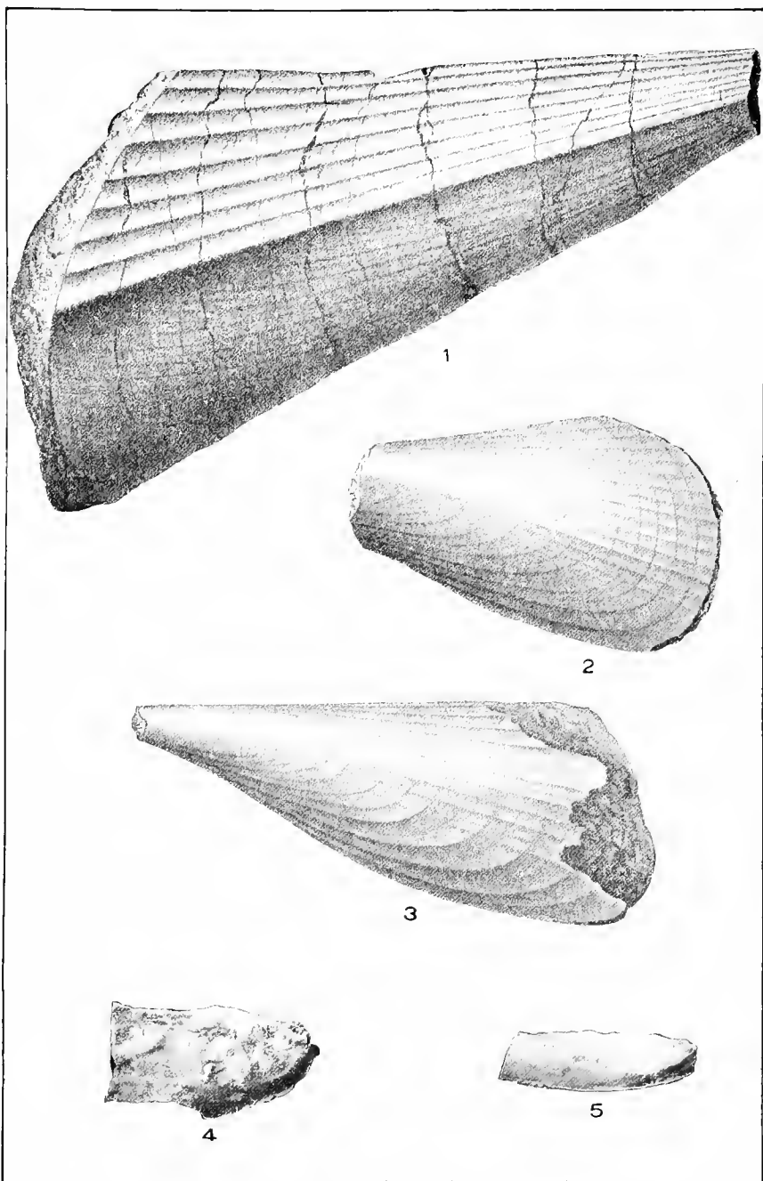
PELECYPODA.
