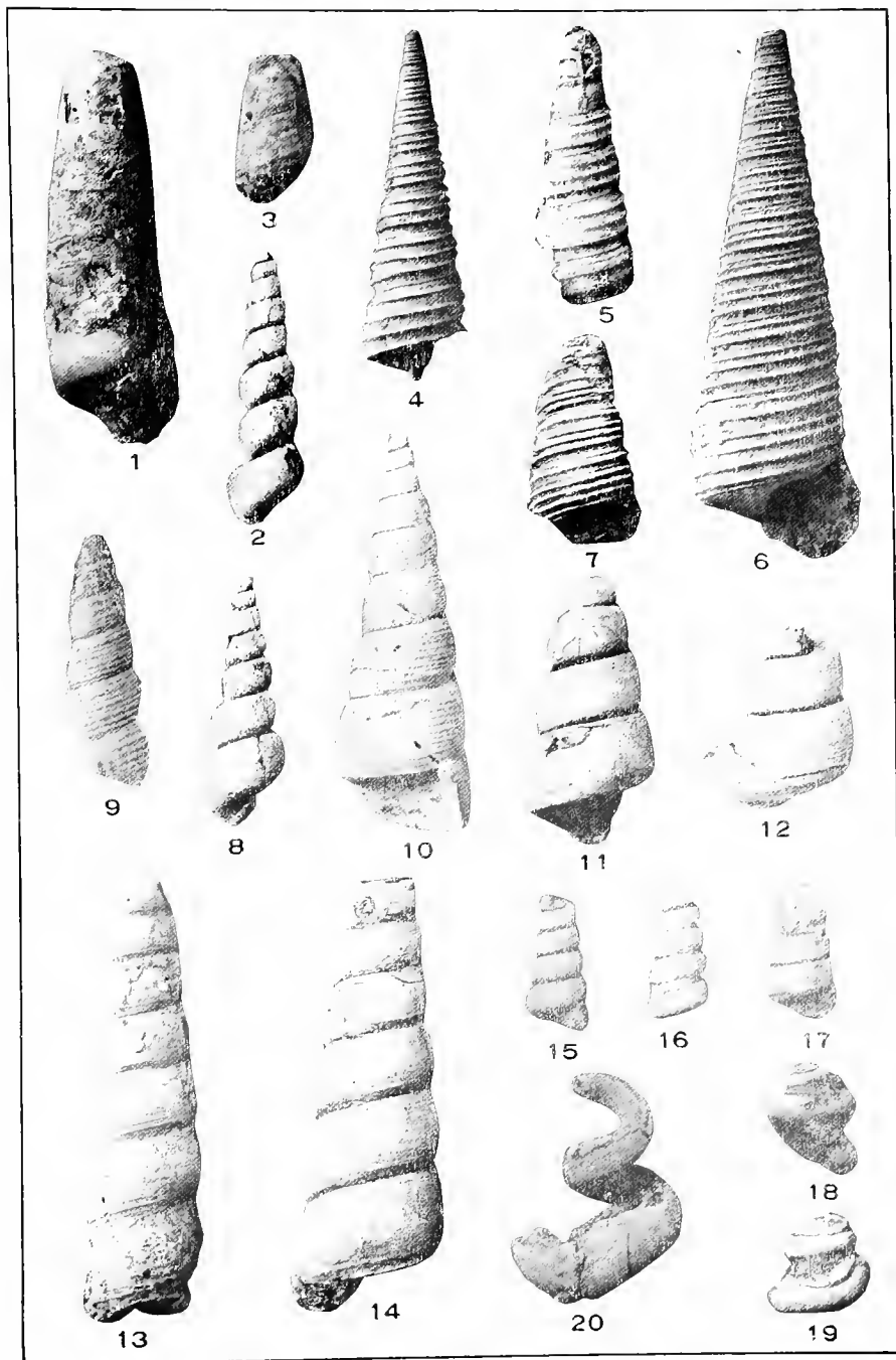
GASTROPODA.
