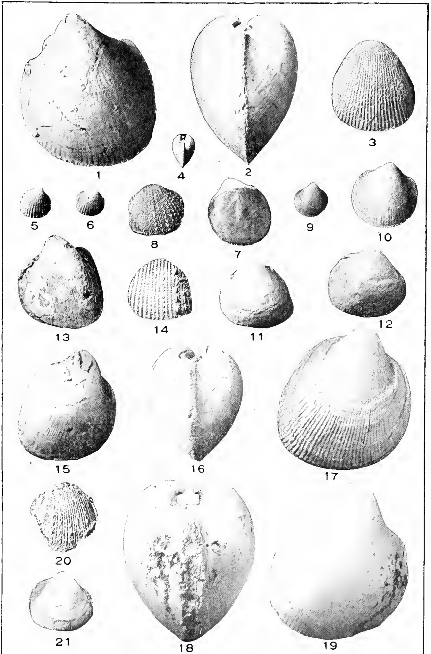
PELECYPODA.
