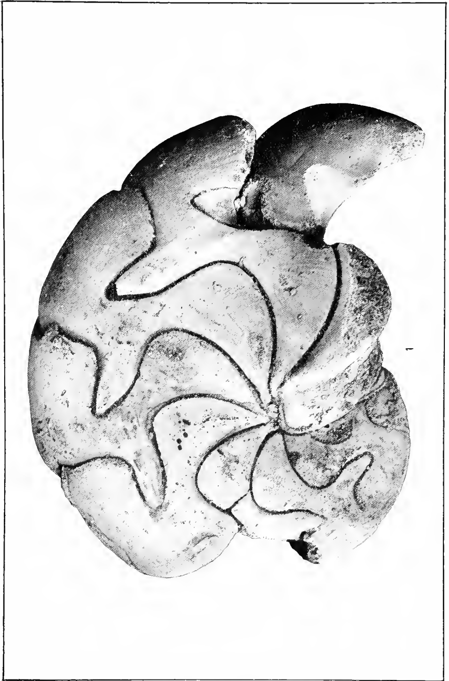
CEPHALOPODA.
