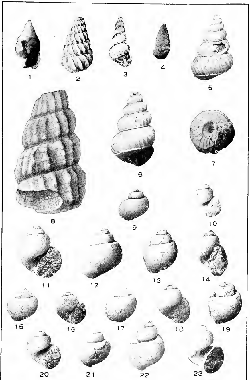
GASTROPODA.
