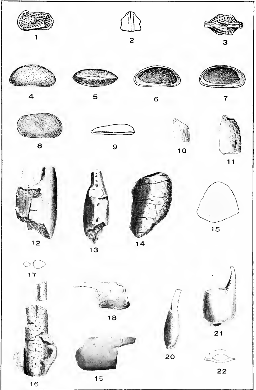
CRUSTACEA.
