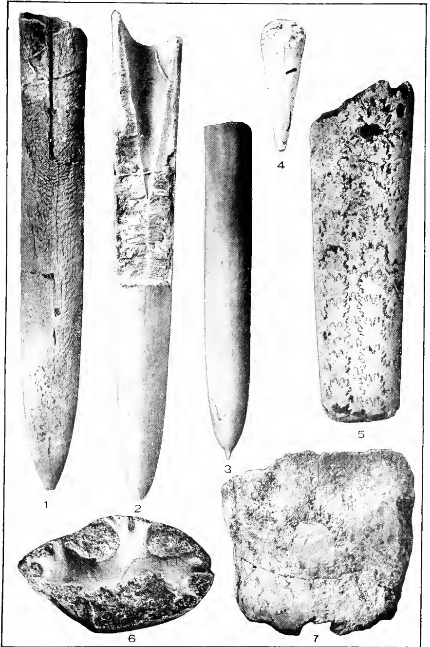
CEPHALOPODA.
