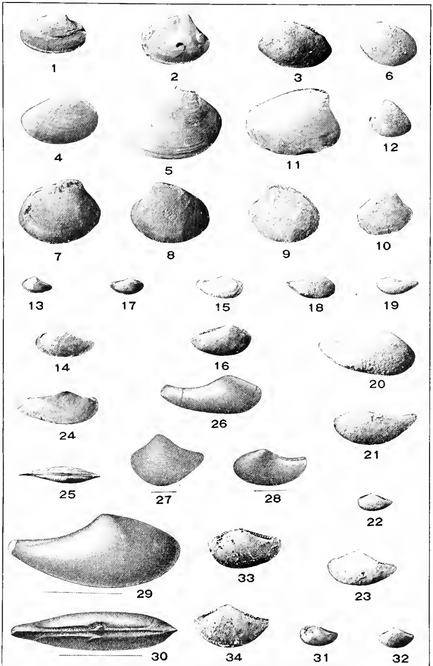
PELECYPODA.
