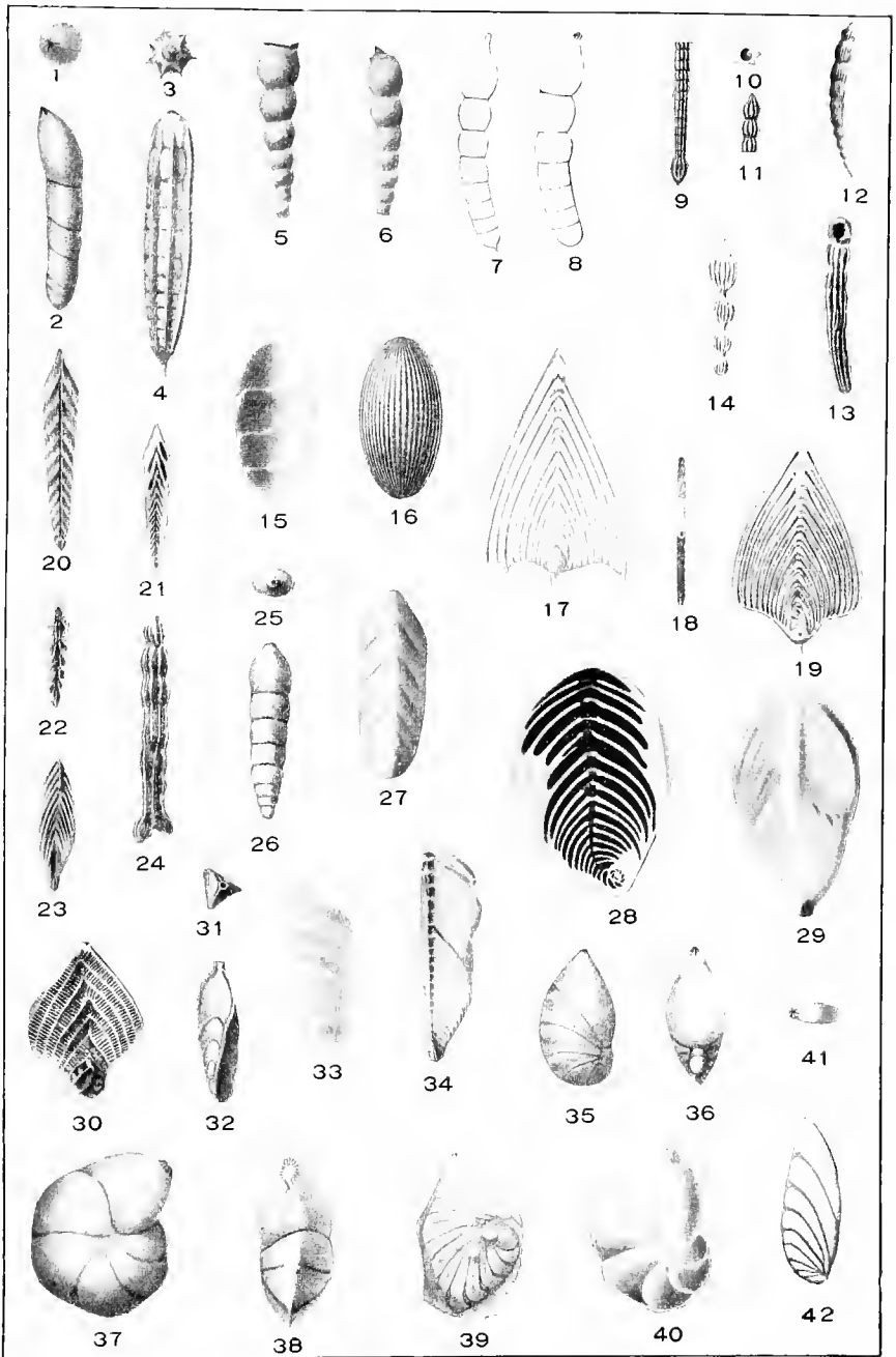
FORAMINIFERA.
