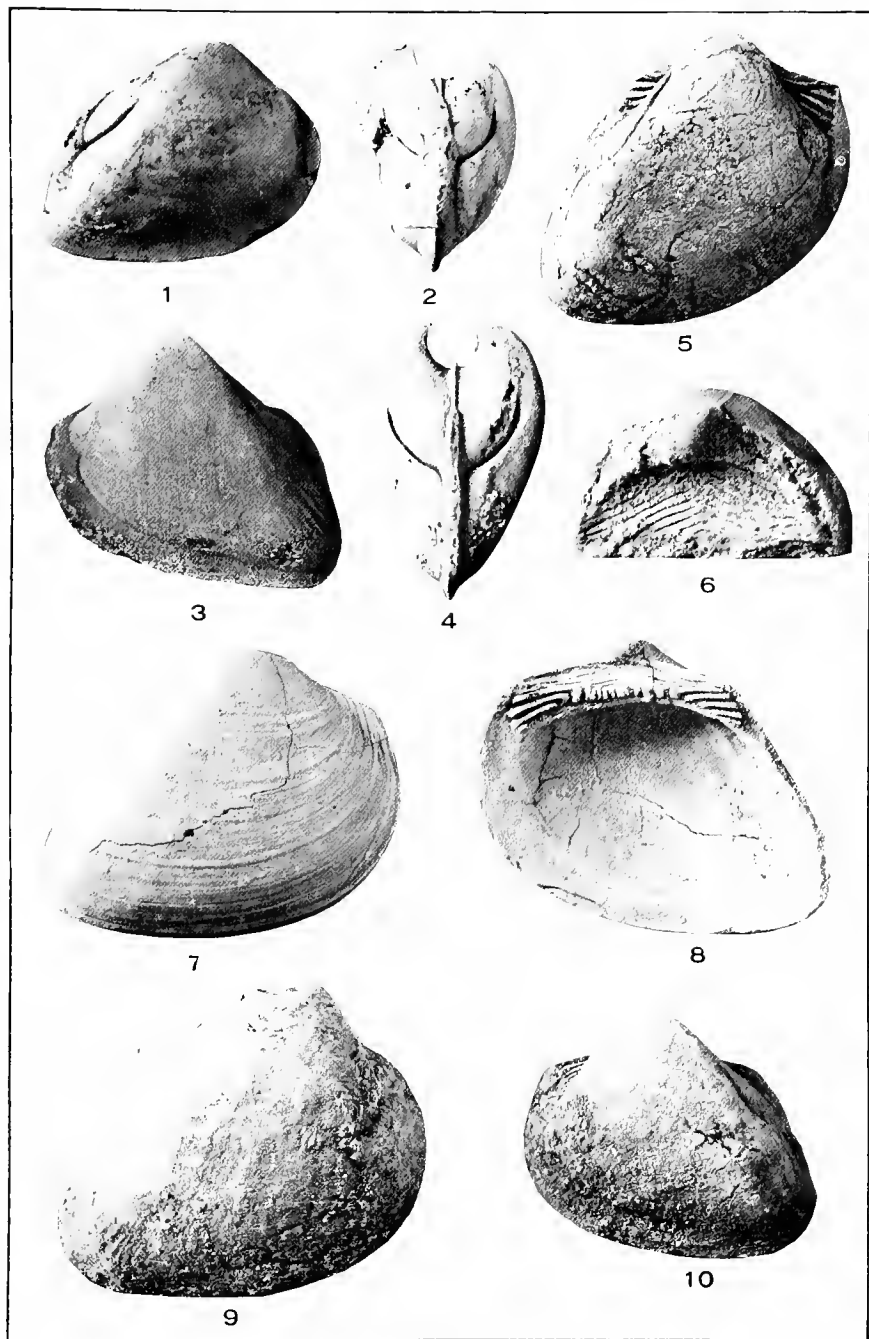
PELECYPODA.
