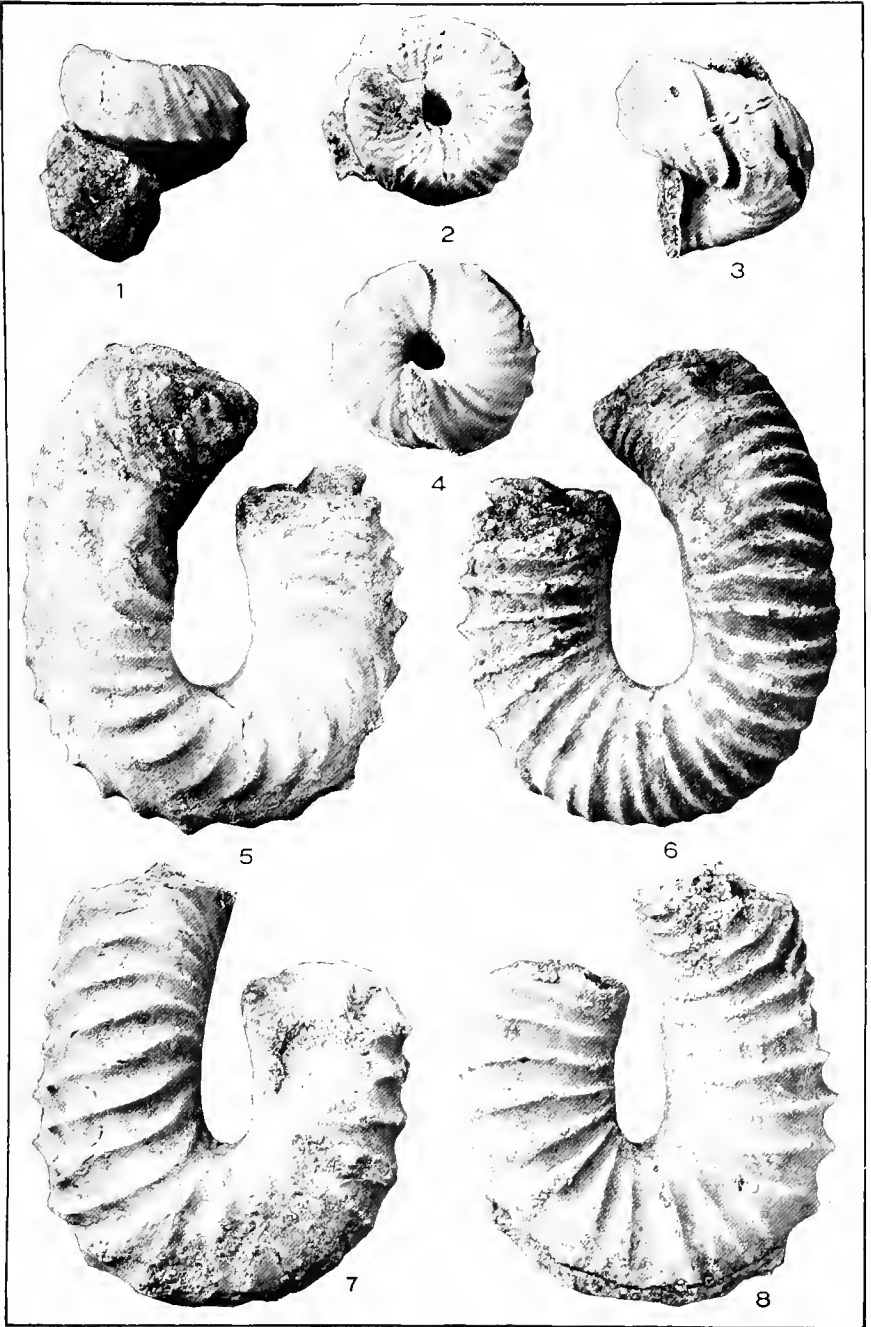
CEPHALOPODA.
