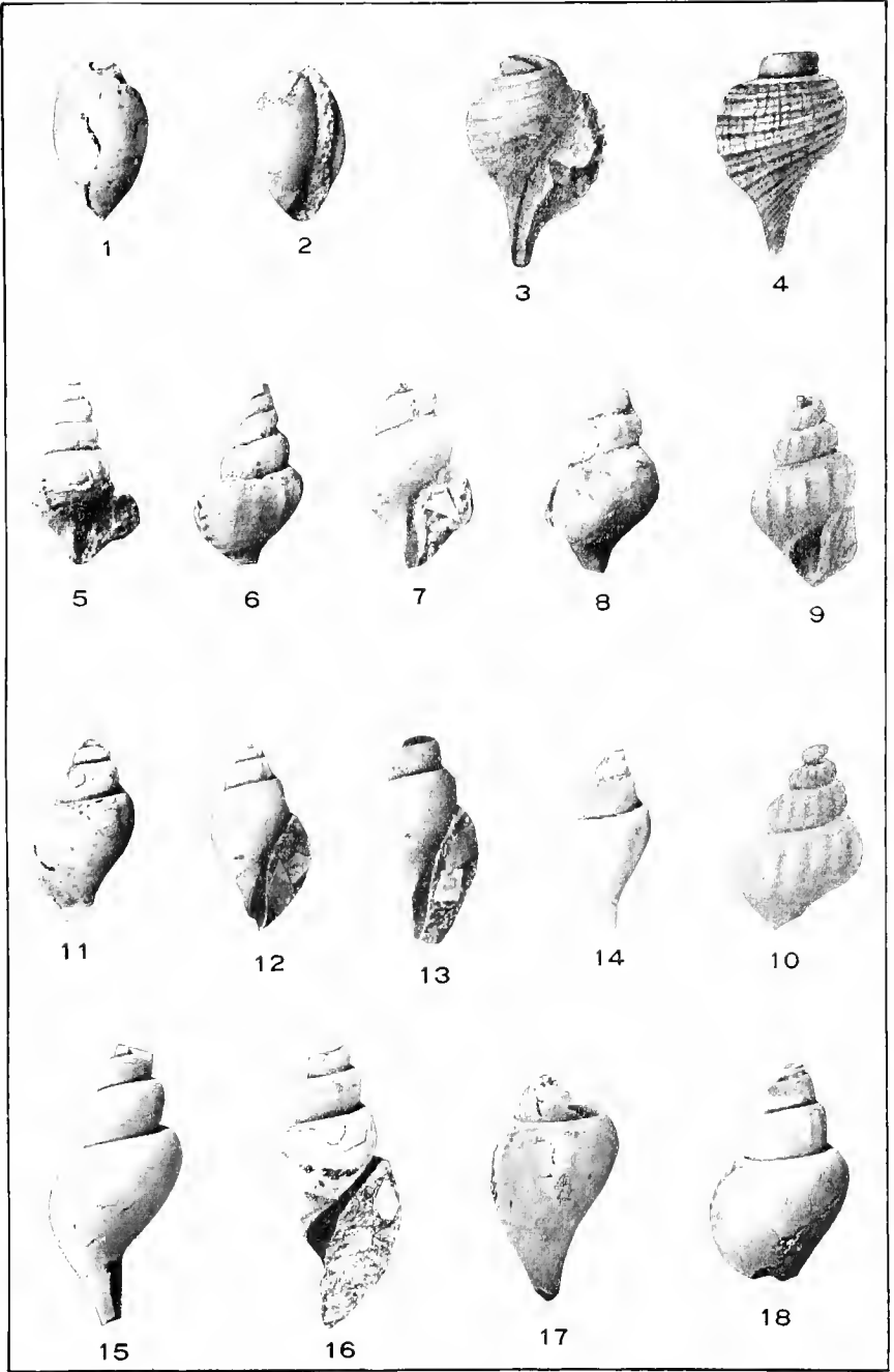
GASTROPODA.
