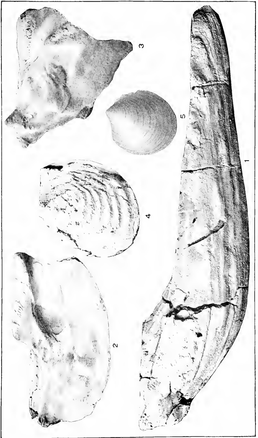
PELECYPODA.
