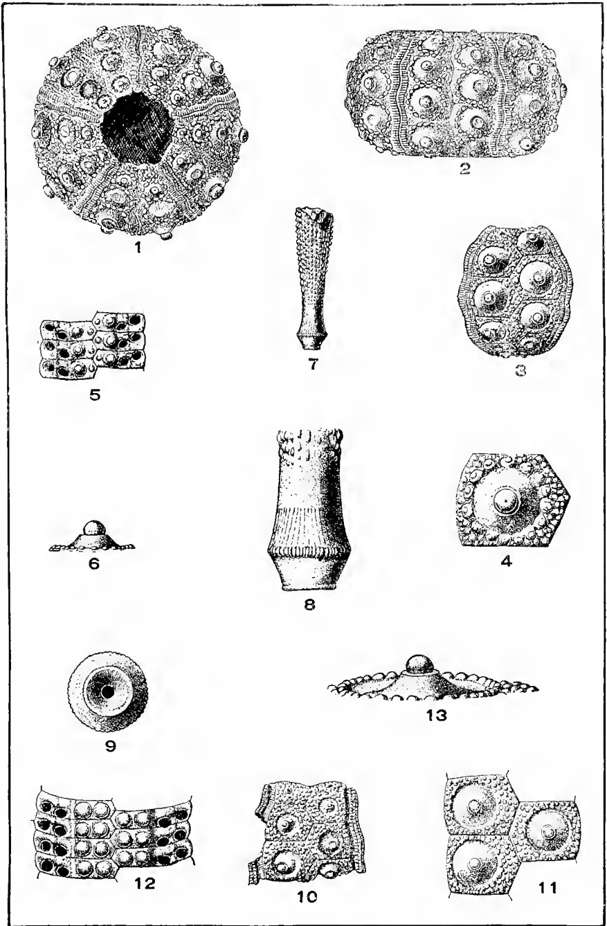
ECHINODERMATA.
