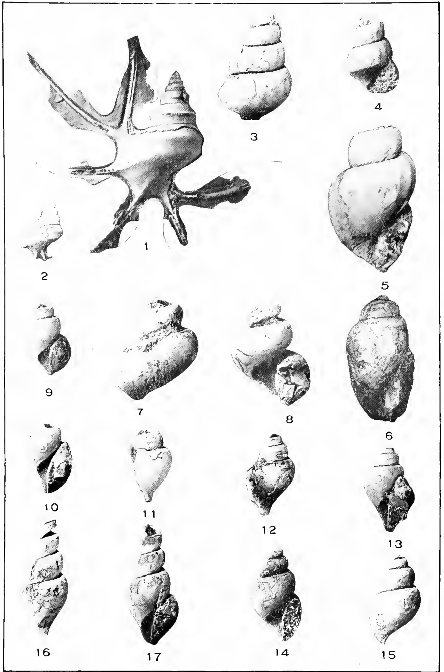
GASTROPODA.
