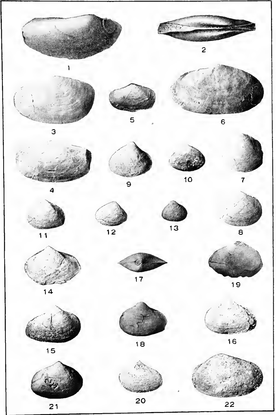
PELECYPODA.
