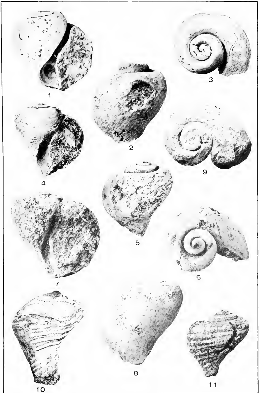
GASTROPODA.
