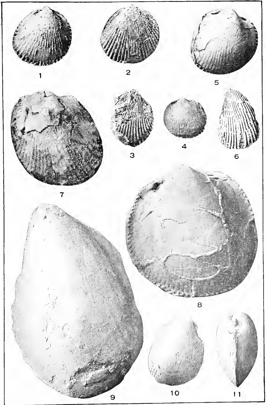
PELECYPODA.
