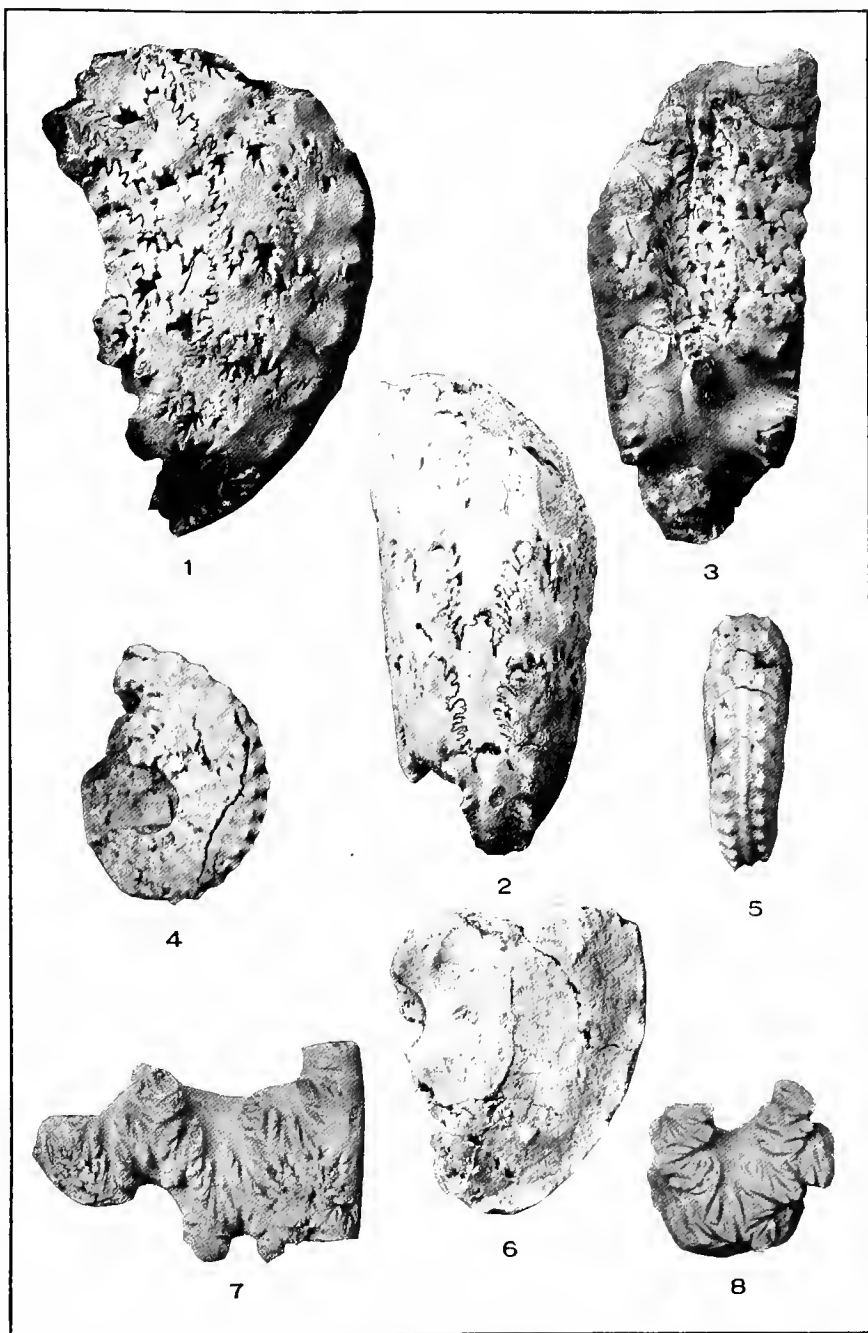
CEPHALOPODA.
