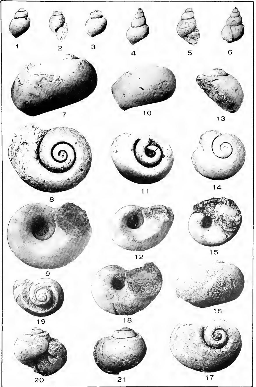
GASTROPODA.
