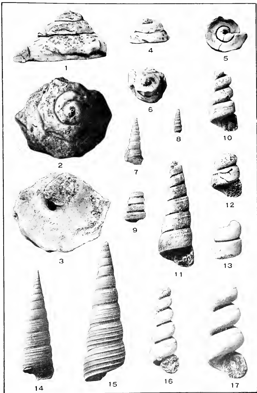
GASTROPODA.
