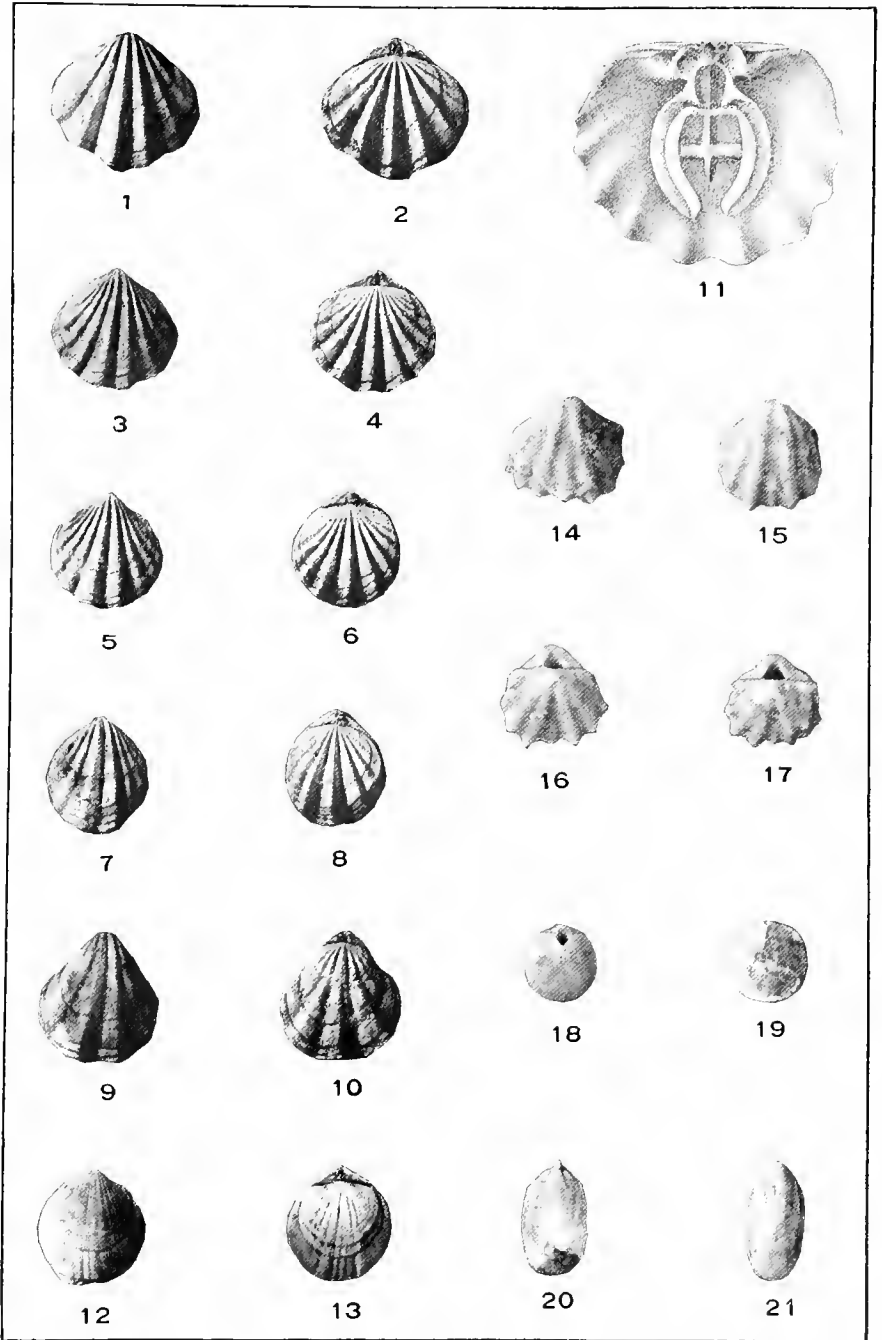
BRACHIOPODA.
