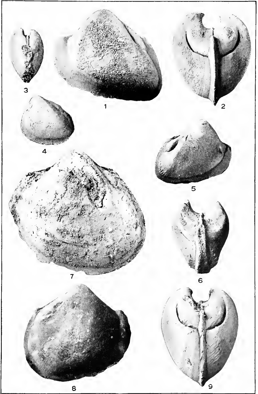
PELECYPODA.
