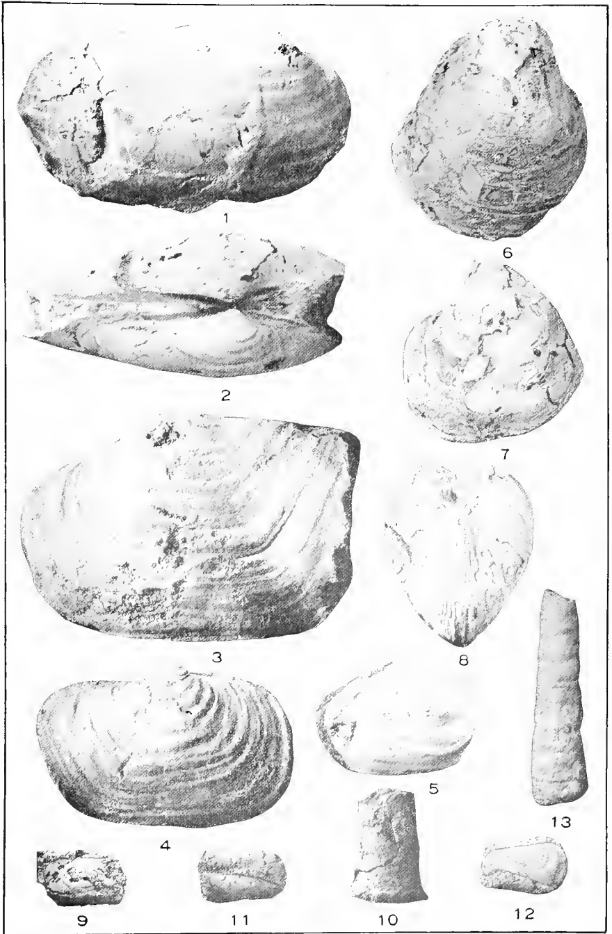
PELECYPODA.
