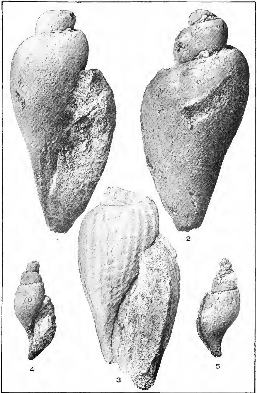
GASTROPODA.
