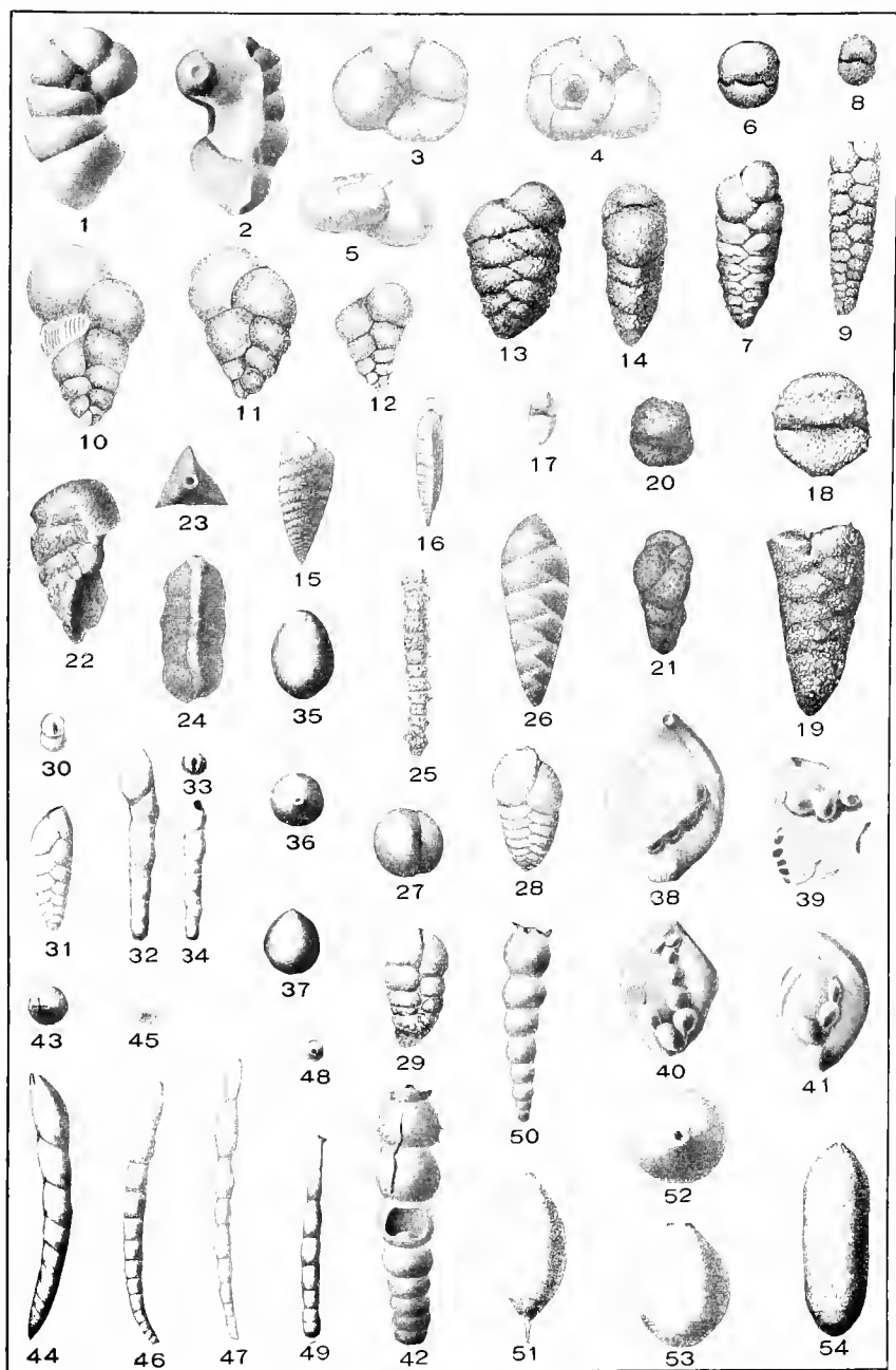
FORAMINIFERA.
