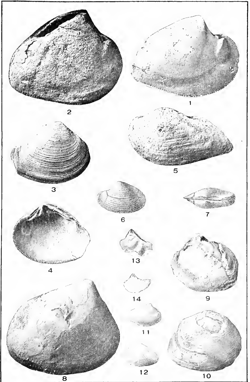
PELECYPODA.
