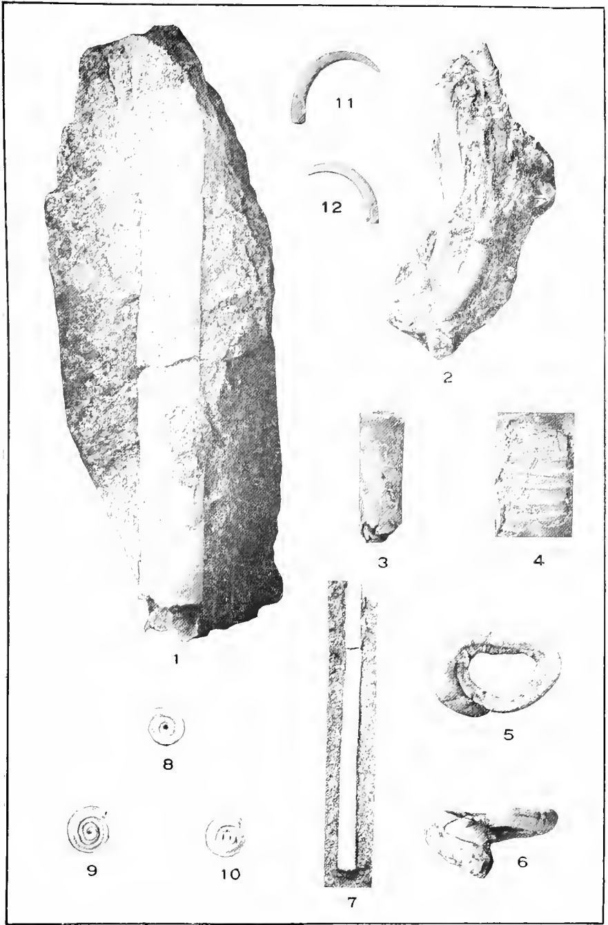
VERMES.
