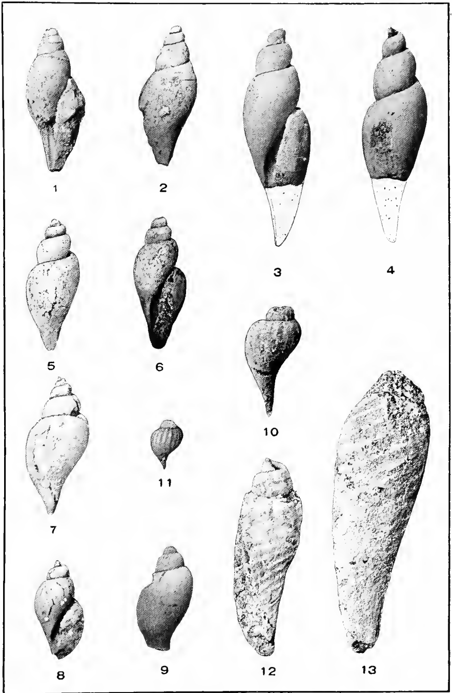
GASTROPODA.
