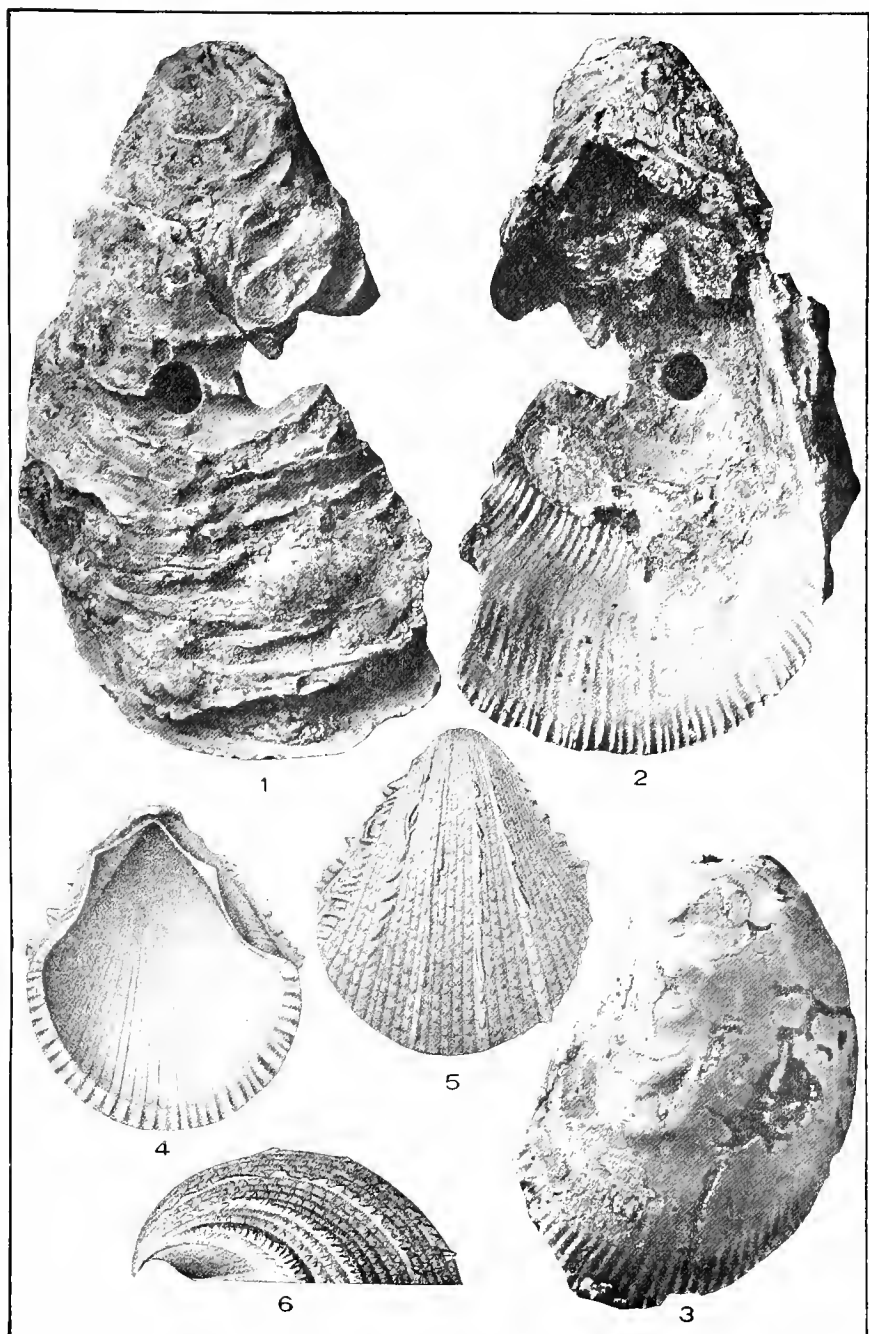
PELECYPODA.
