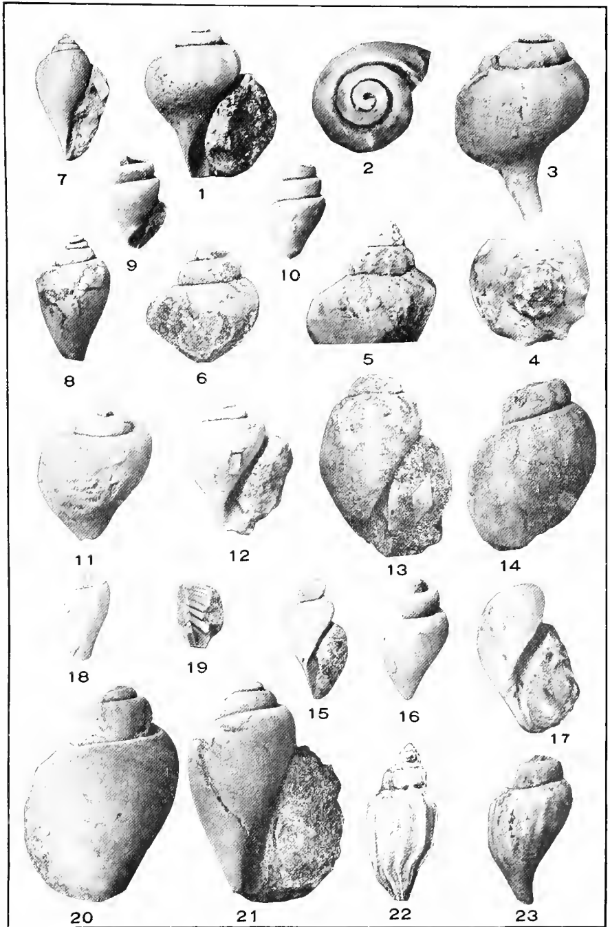
GASTROPODA.
