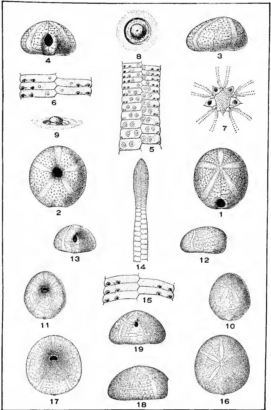
ECHINODERMATA.
