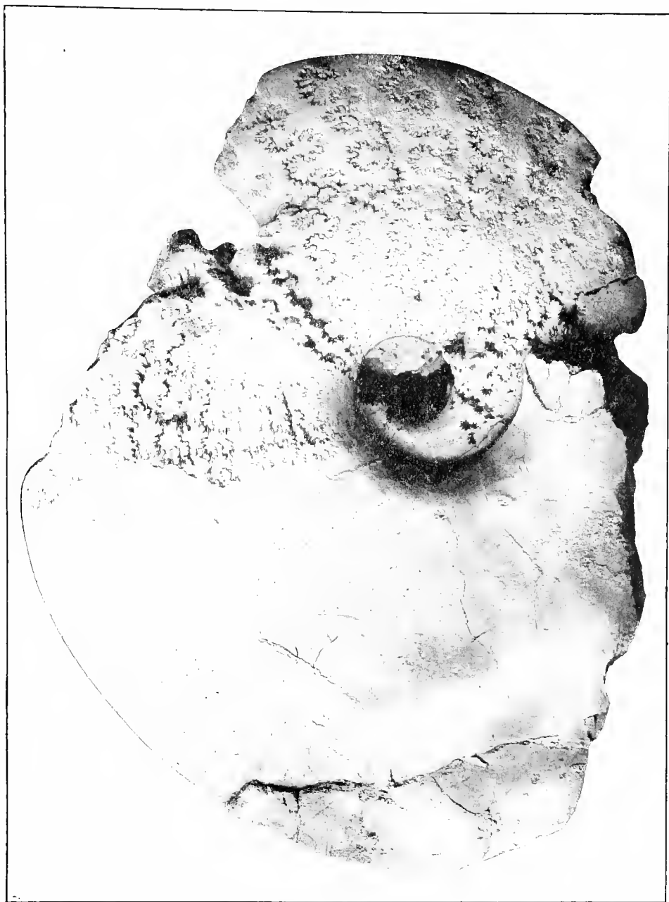
CEPHALOPODA.
