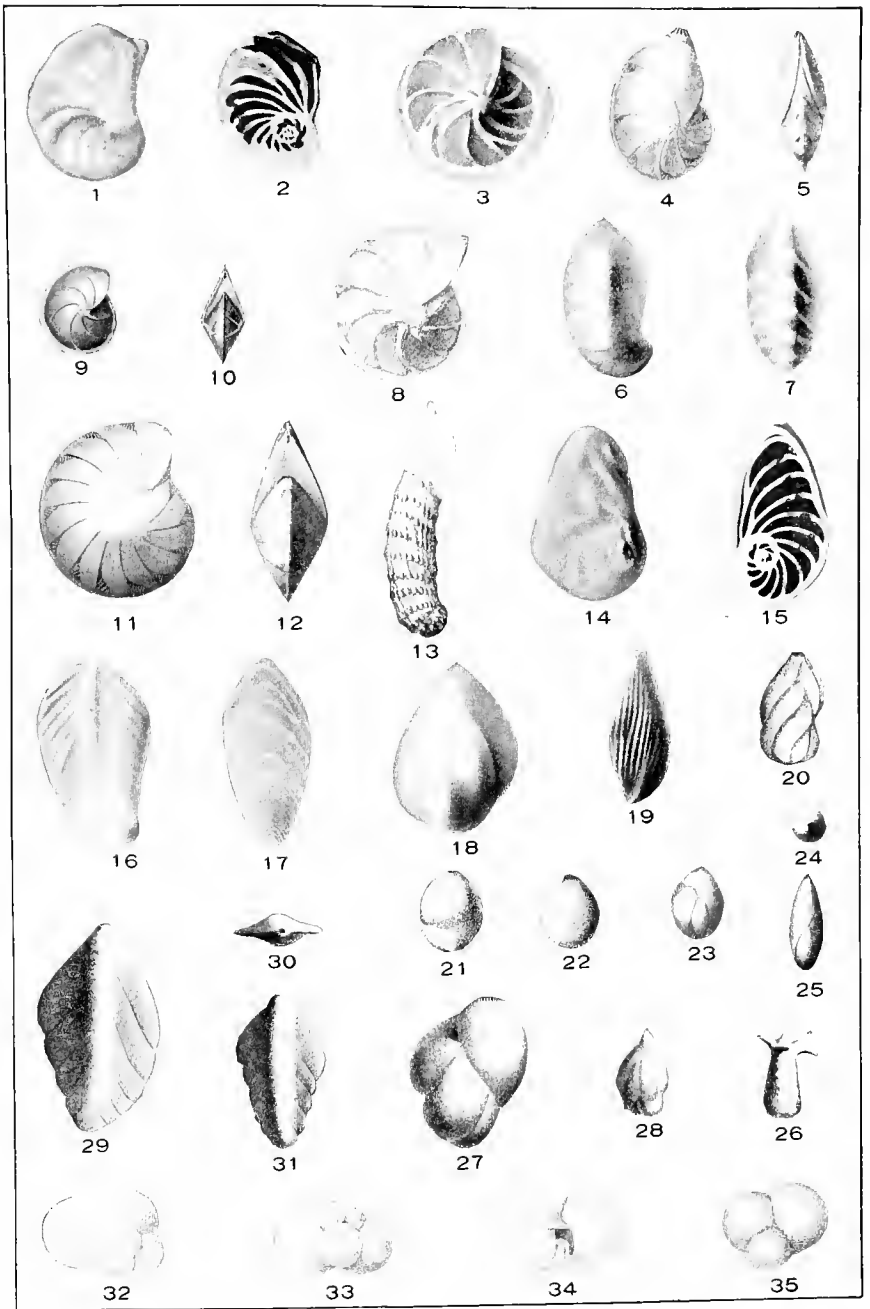
FORAMINIFERA.
