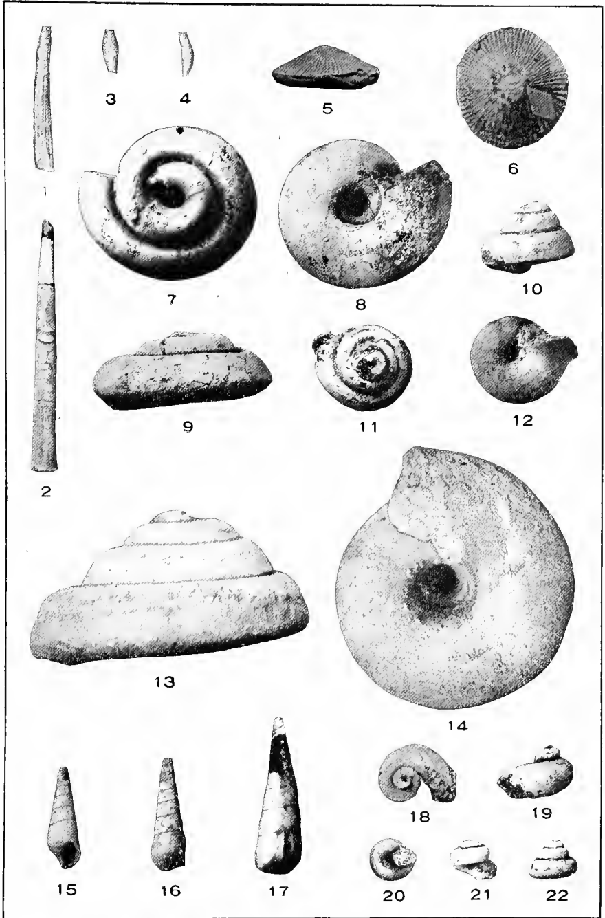
GASTROPODA.
