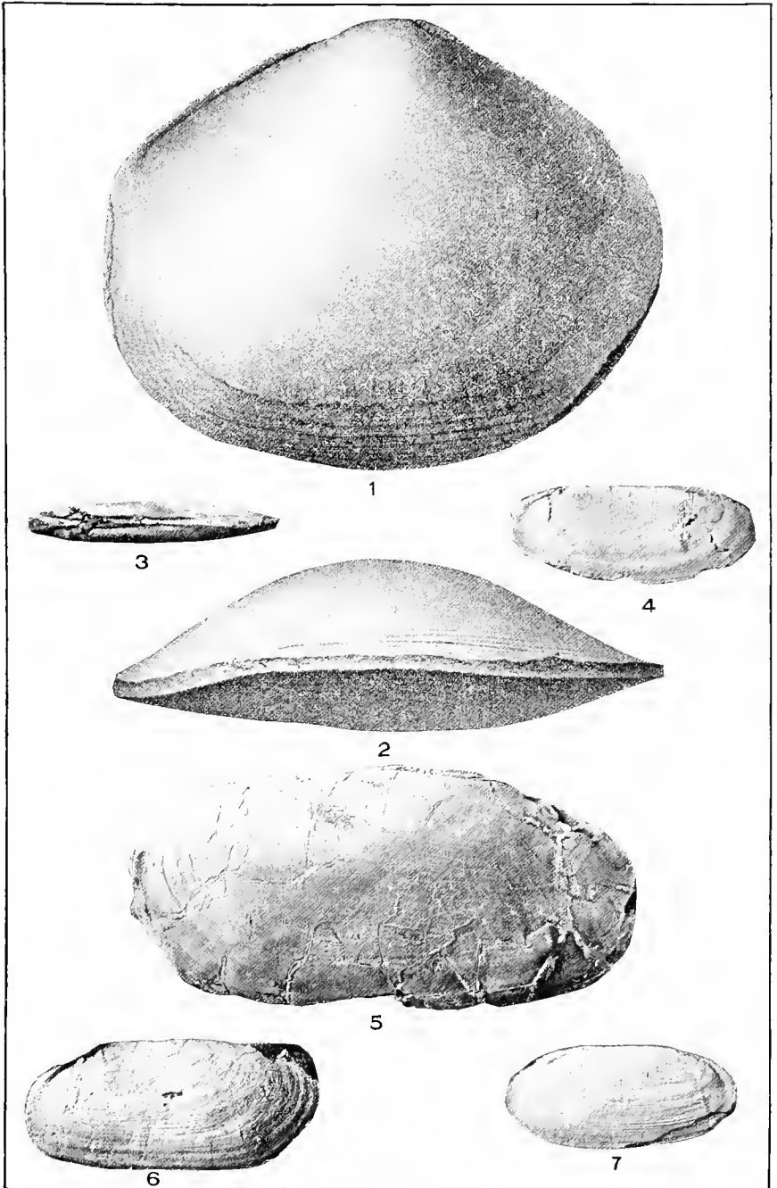
PELECYPODA.
