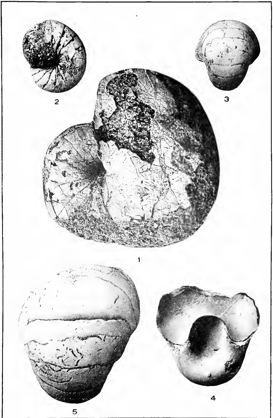
GASTROPODA.
