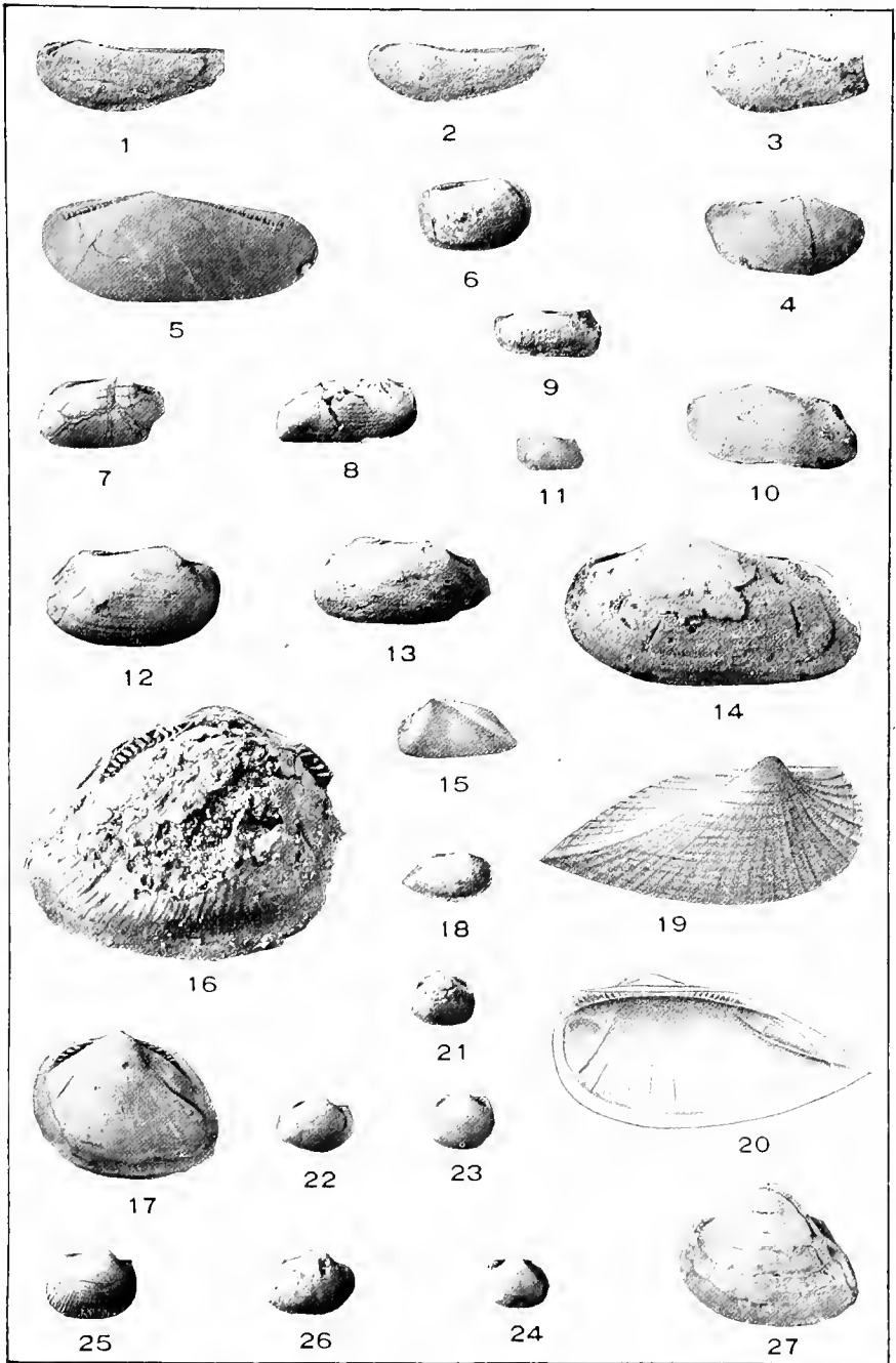
PELECYPODA.
