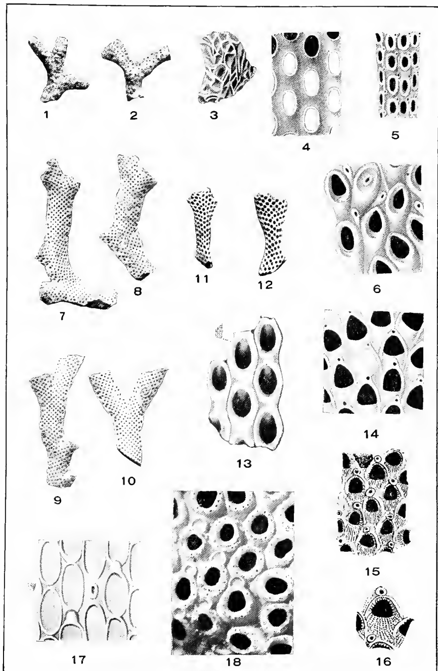
BRYOZOA.
