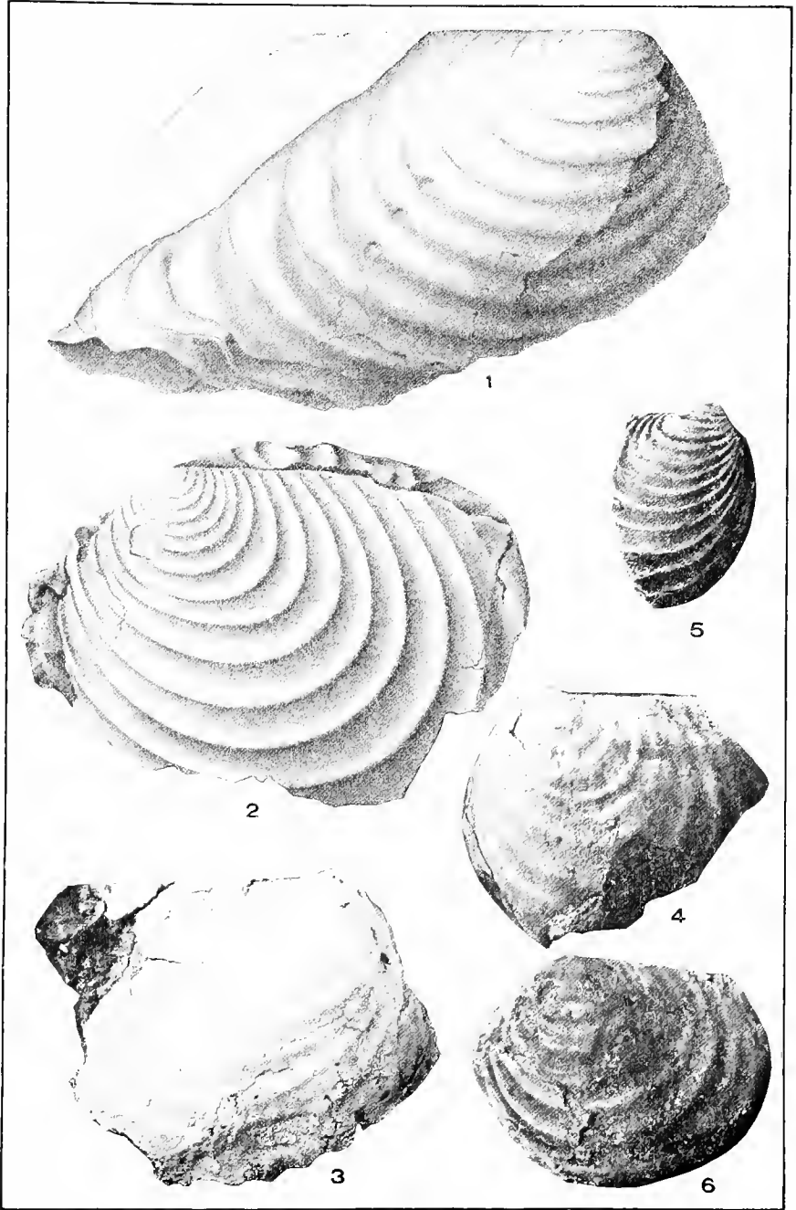
PELECYPODA.
