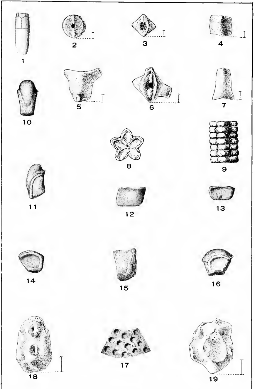
ECHINODERMATA.
