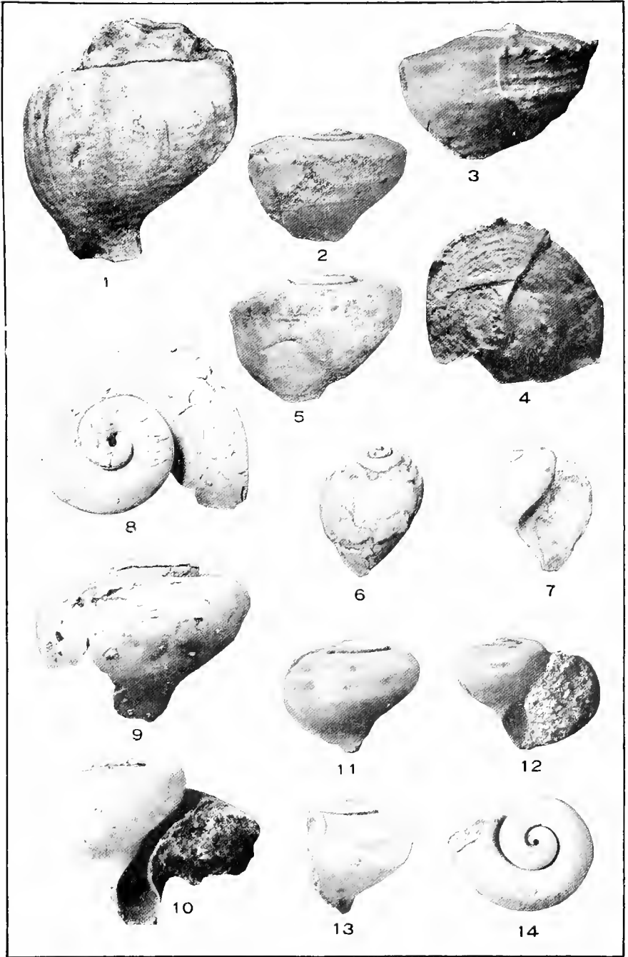
GASTROPODA.
