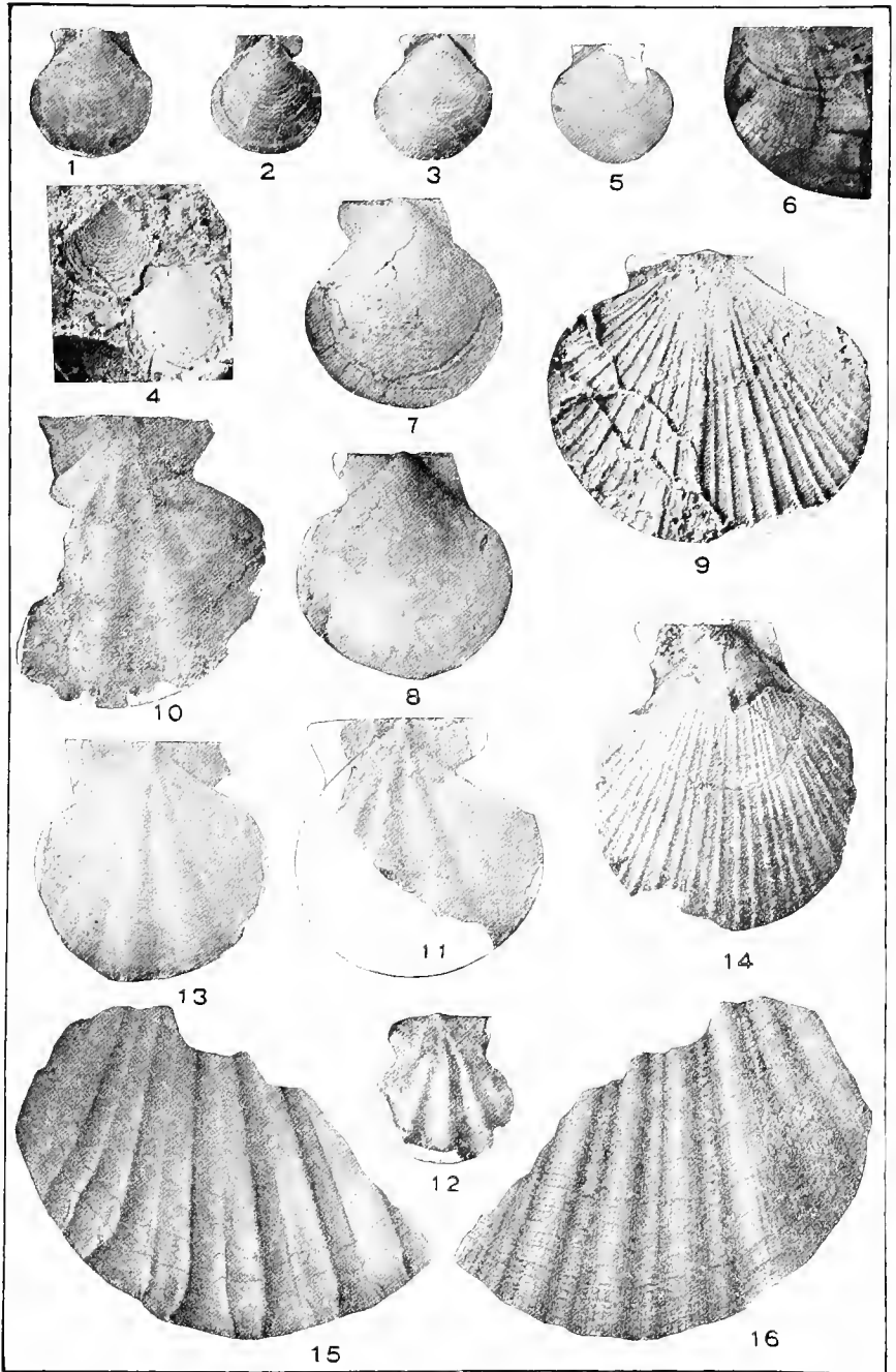
PELECYPODA.
