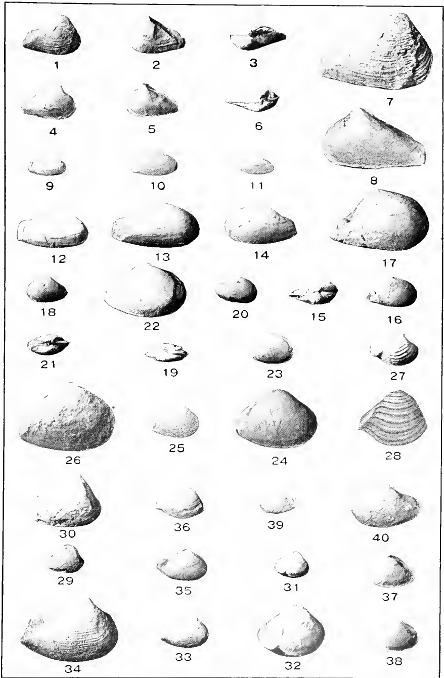
PELECYPODA.
