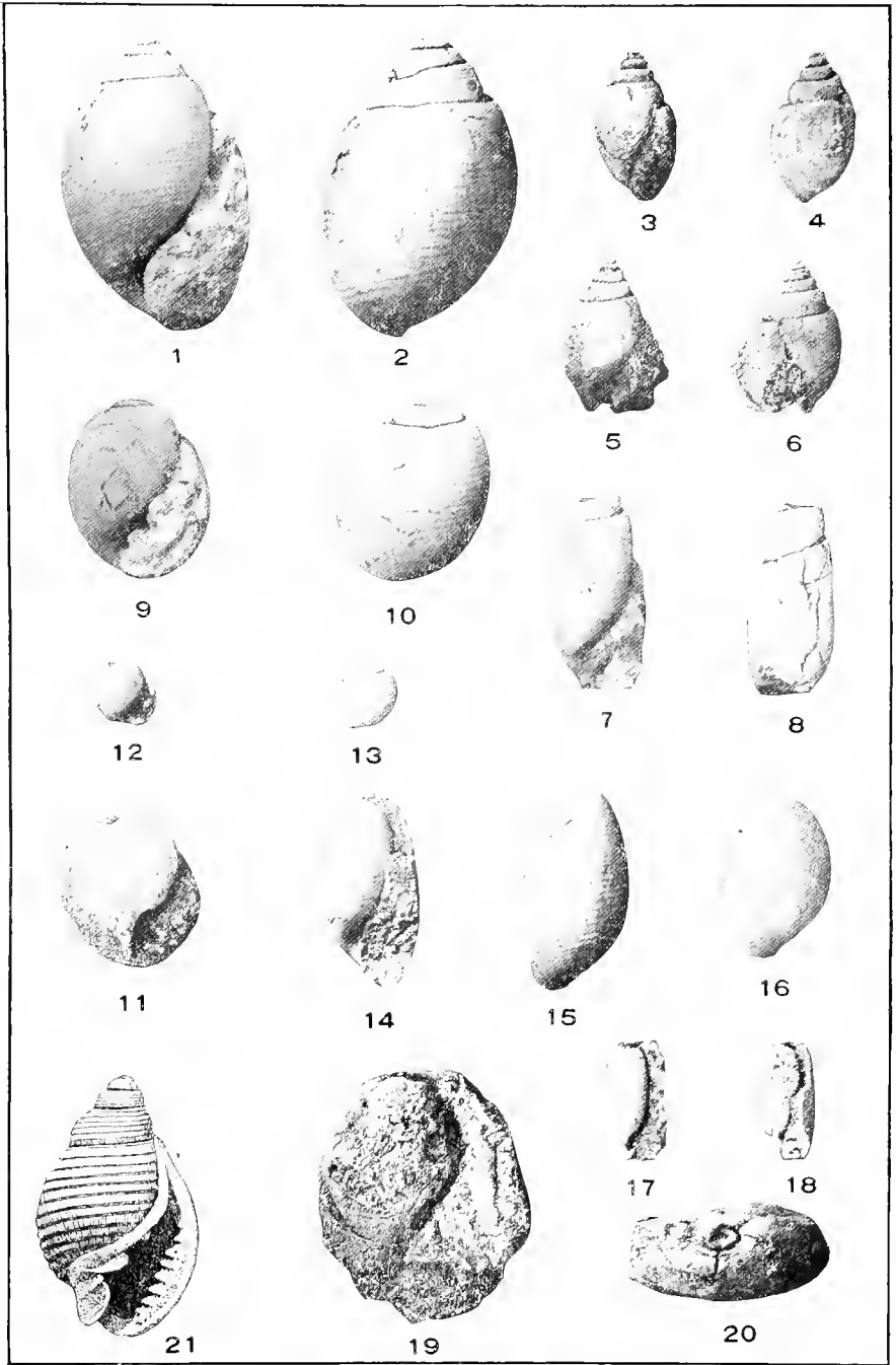
GASTROPODA.
