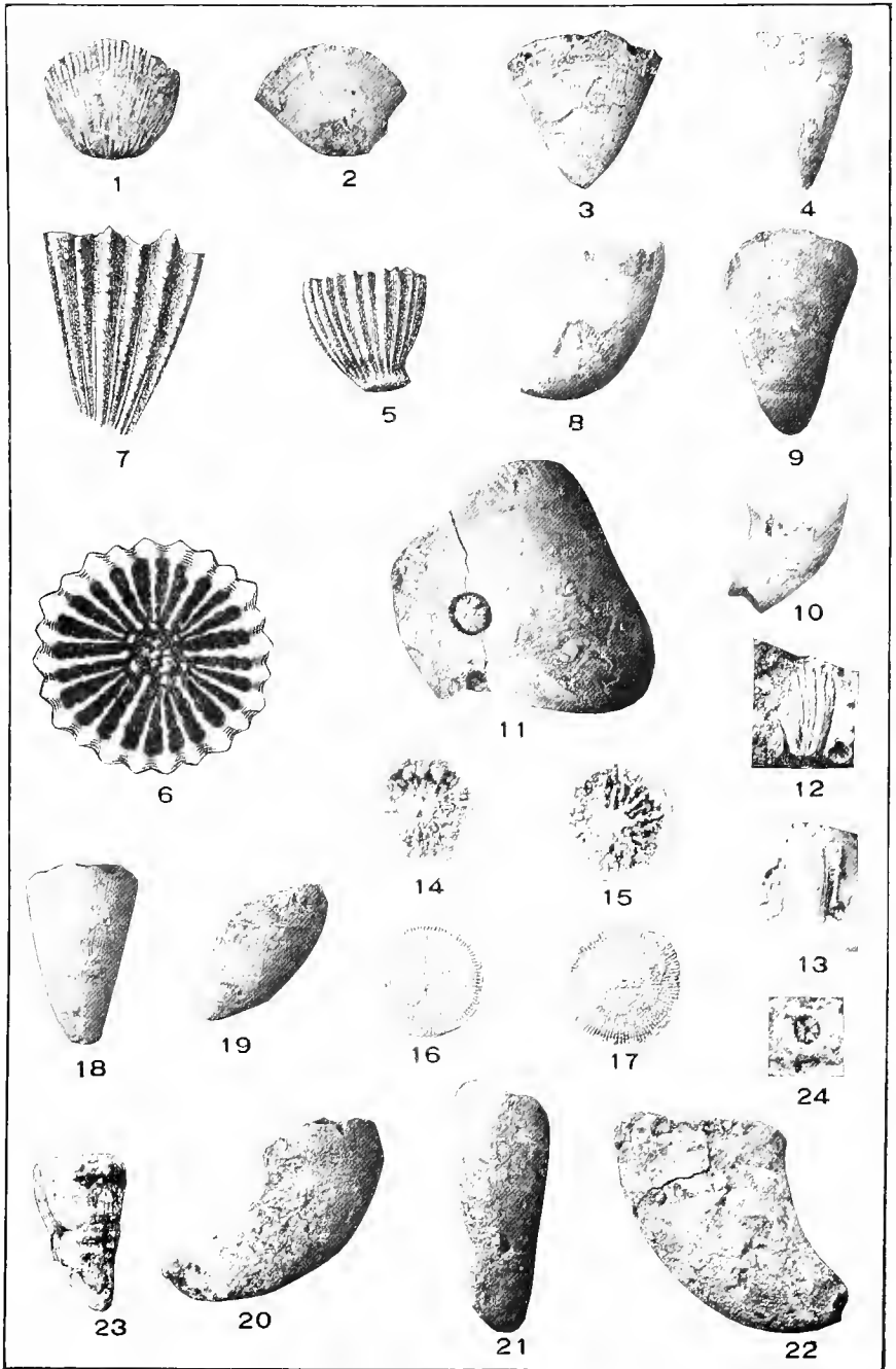
ANTHOZOA.
