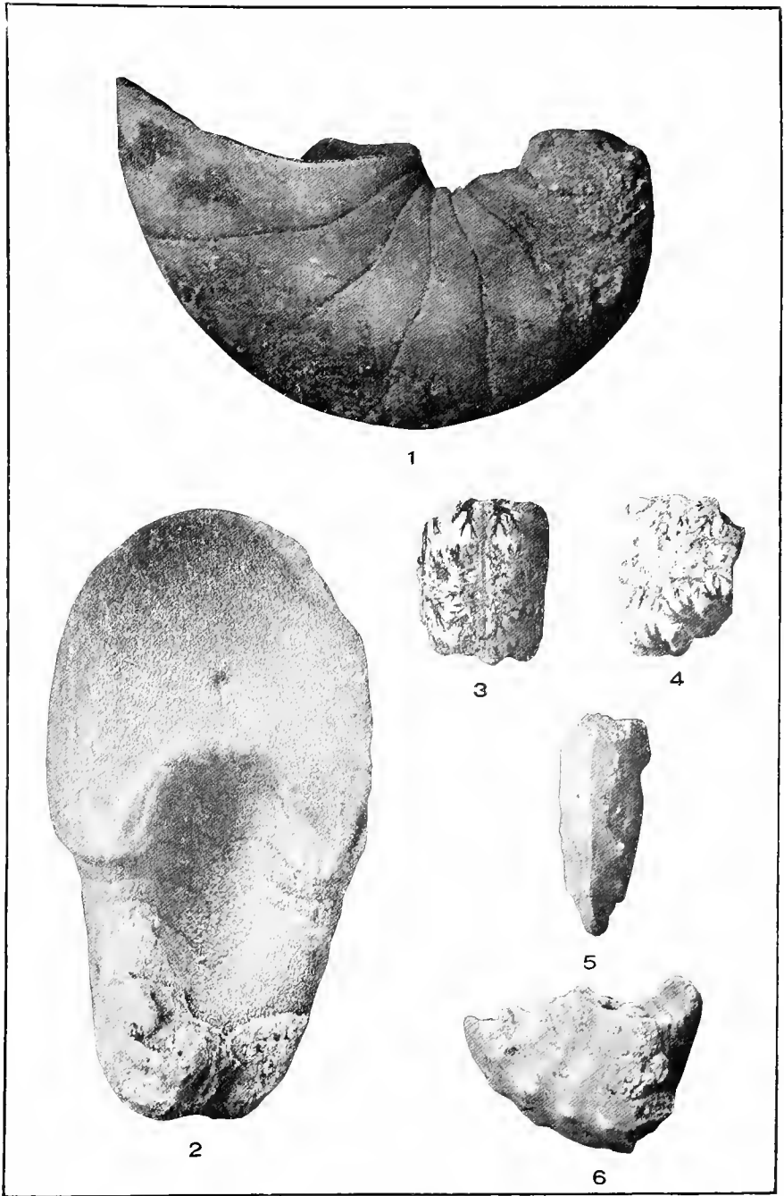
CEPHALOPODA.
