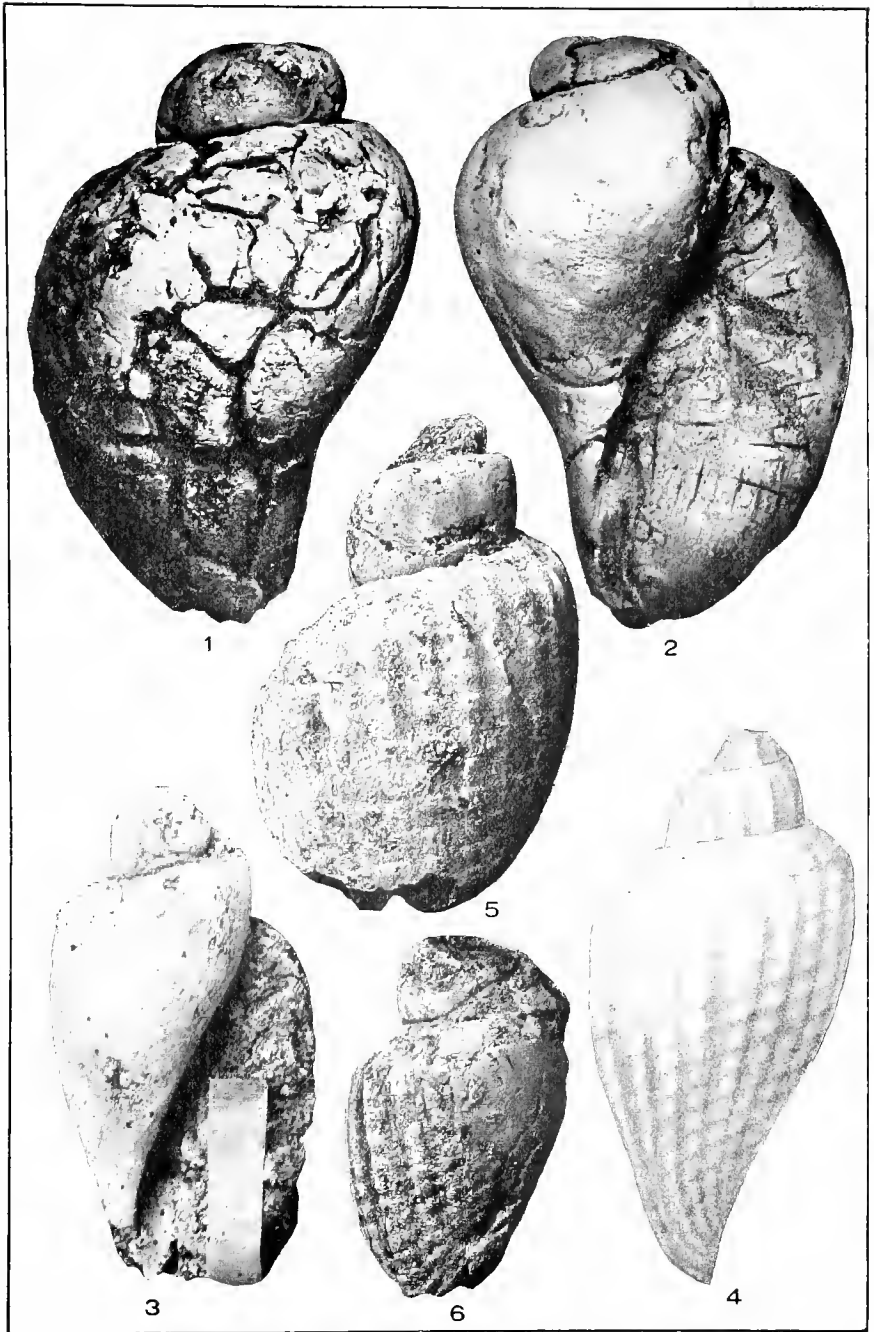
GASTROPODA.
