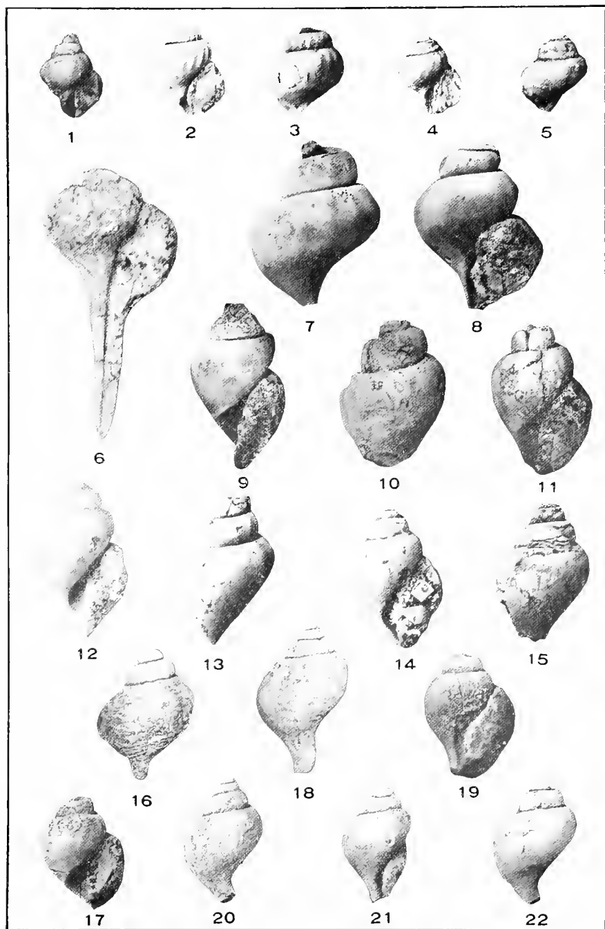
GASTROPODA.
