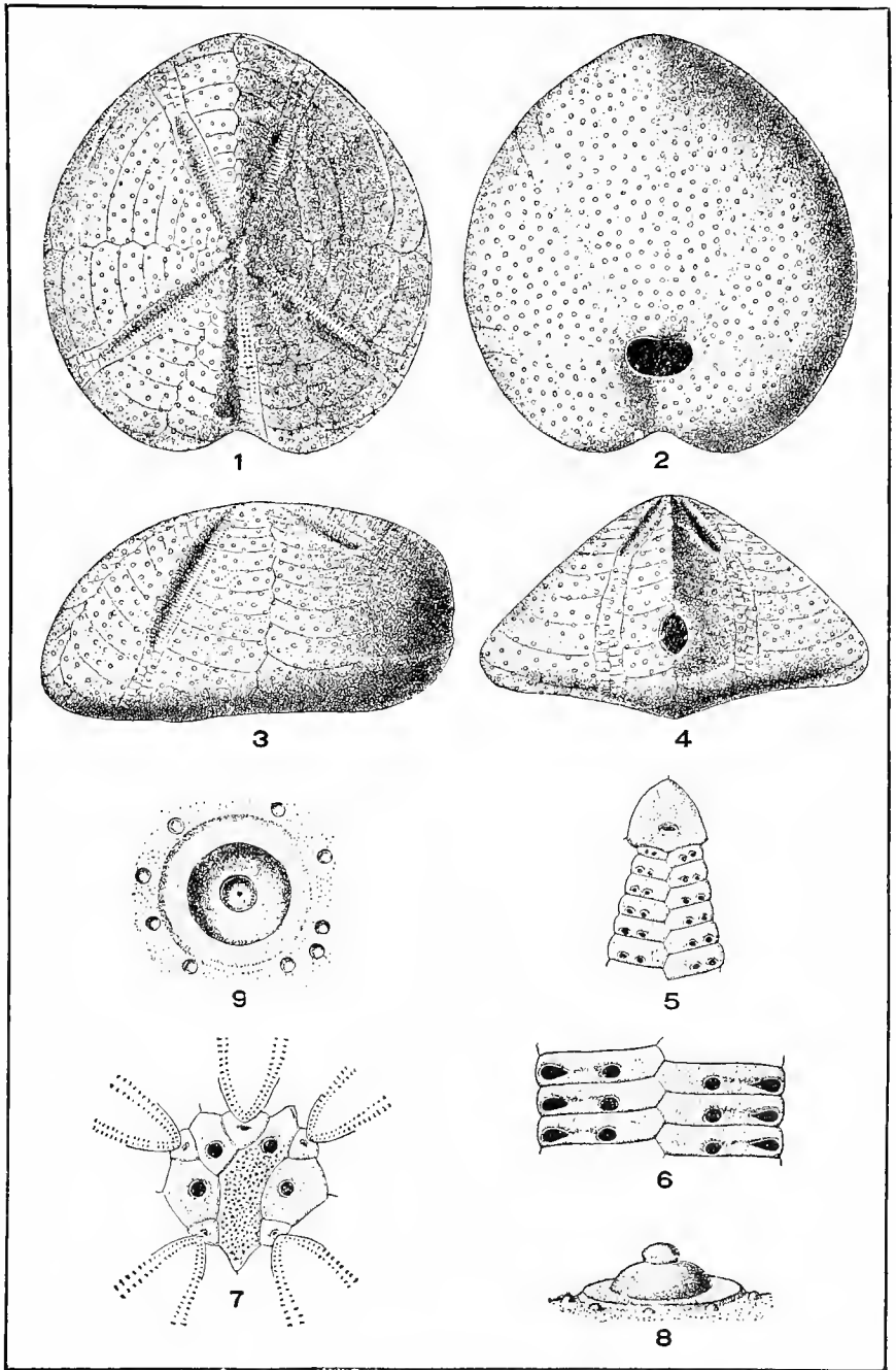
ECHINODERMATA.
