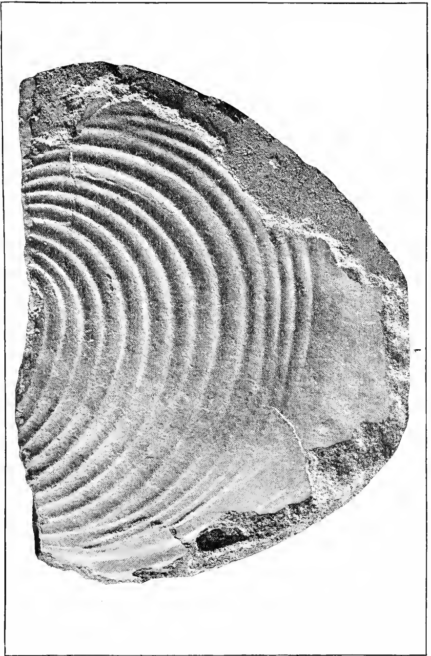
PELECYPODA.
