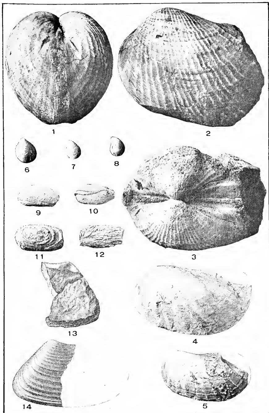
PELECYPODA.
