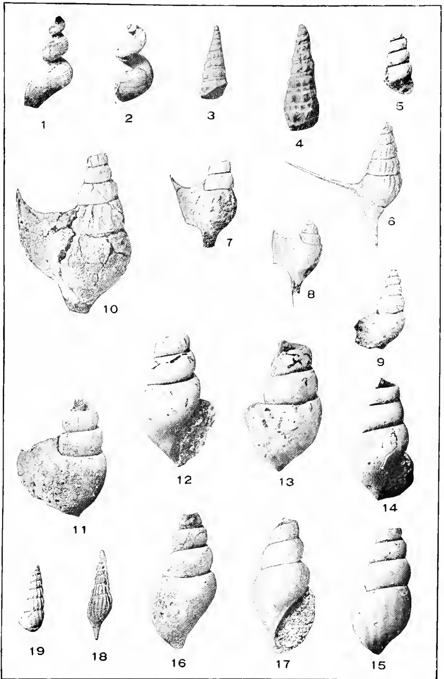
GASTROPODA.
