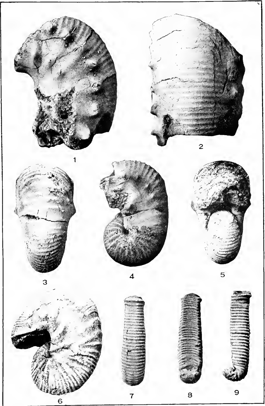
CEPHALOPODA.
