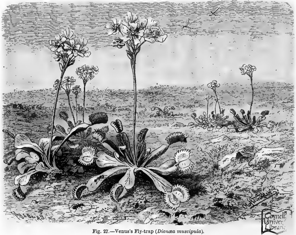
Fig. 27.—Venus's Fly-trap ( Dionaea muscipula ).
