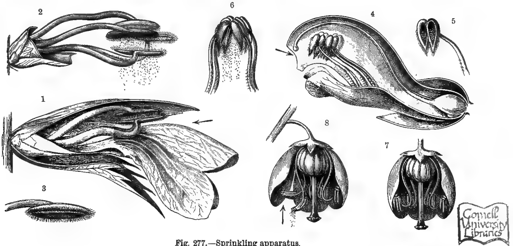
Fig. 277.—Sprinkling apparatus.
