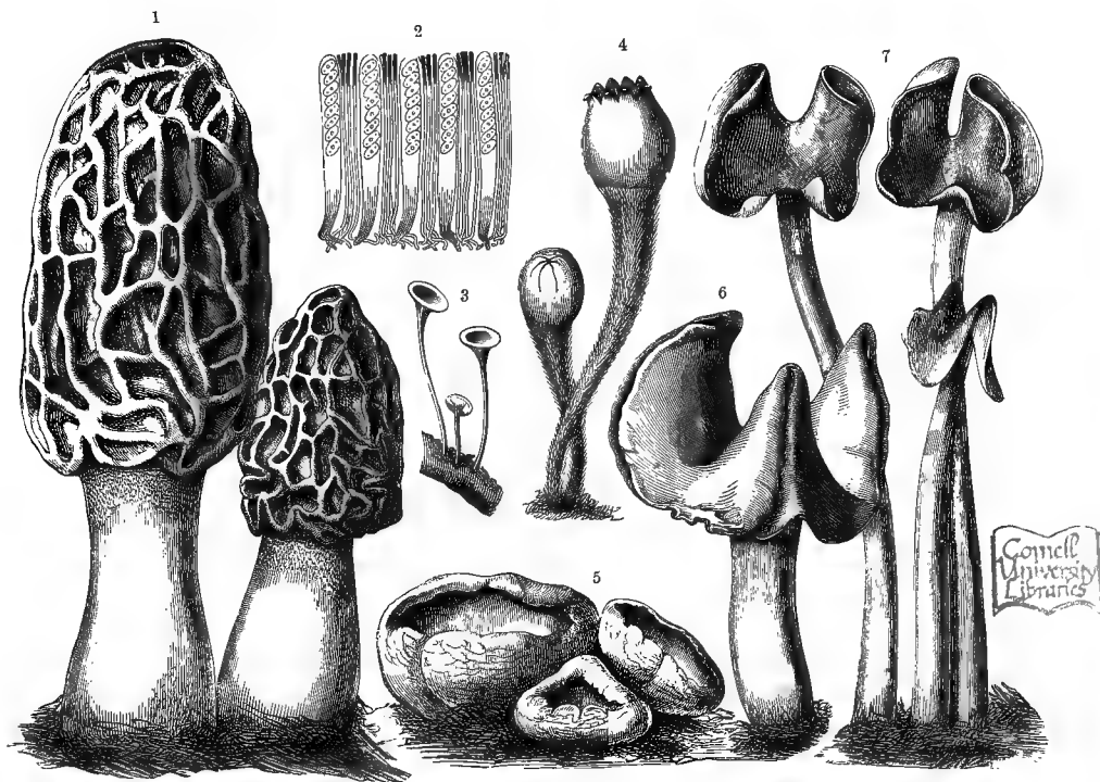
Fig. 194.—Discomycetes.
