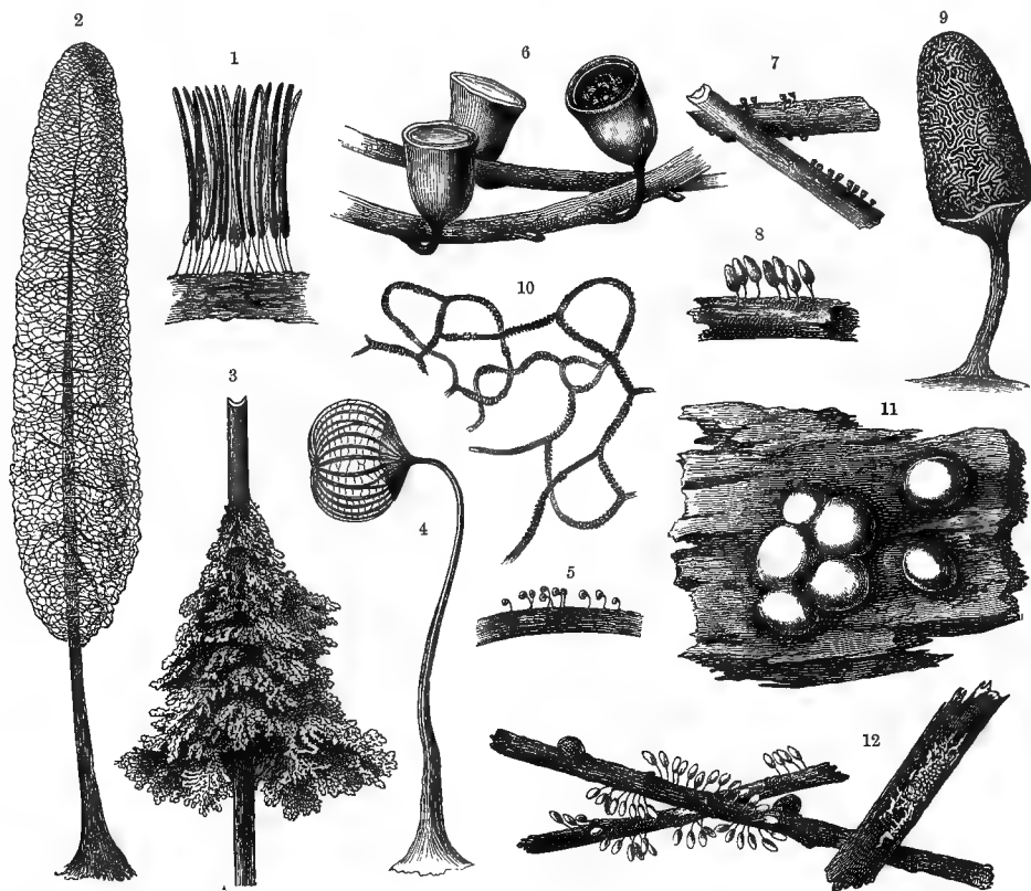
Fig. 355.—Myxomycetes.
