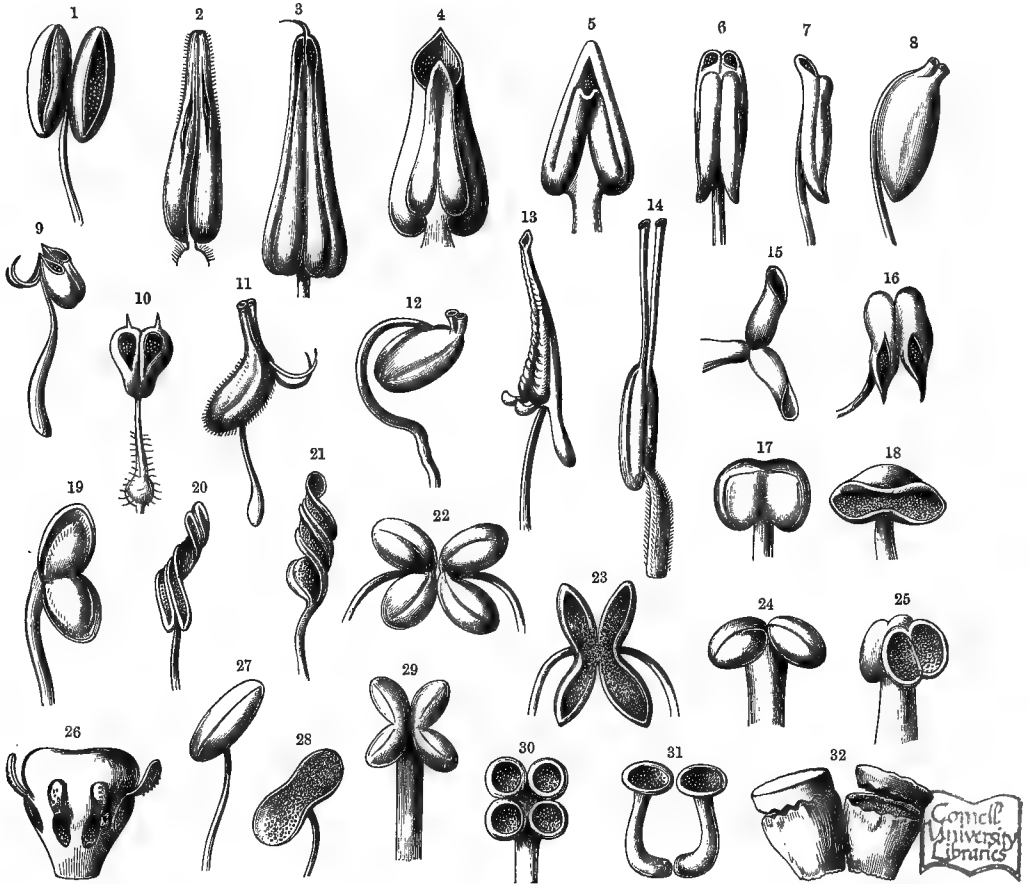
Fig. 216.—Stamens.
