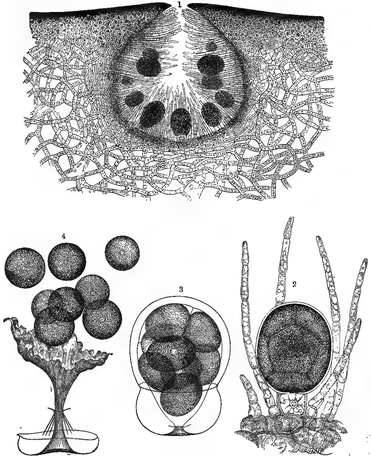
Fig. 202.— Fucus vesiculosus .
