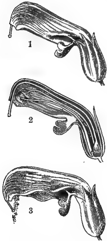
Fig. 276.— Pedicularis recutita .
