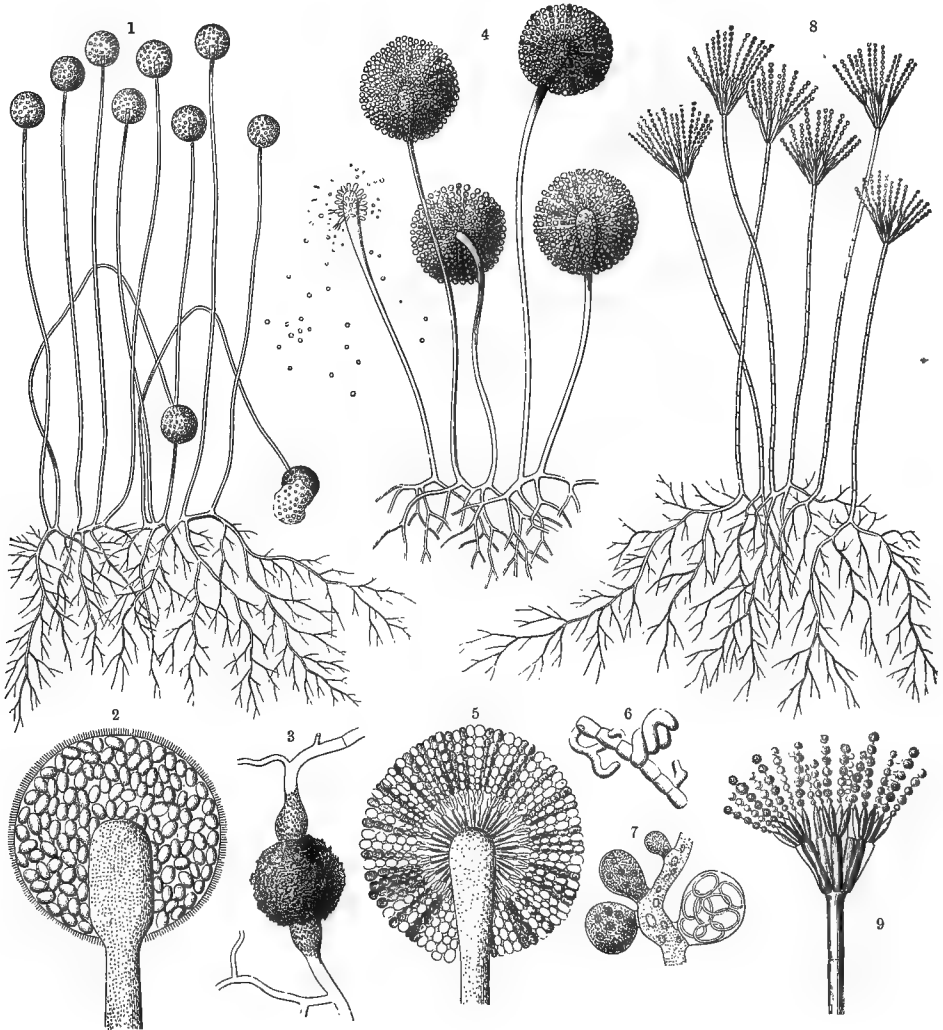
Fig. 193.—Moulds.
