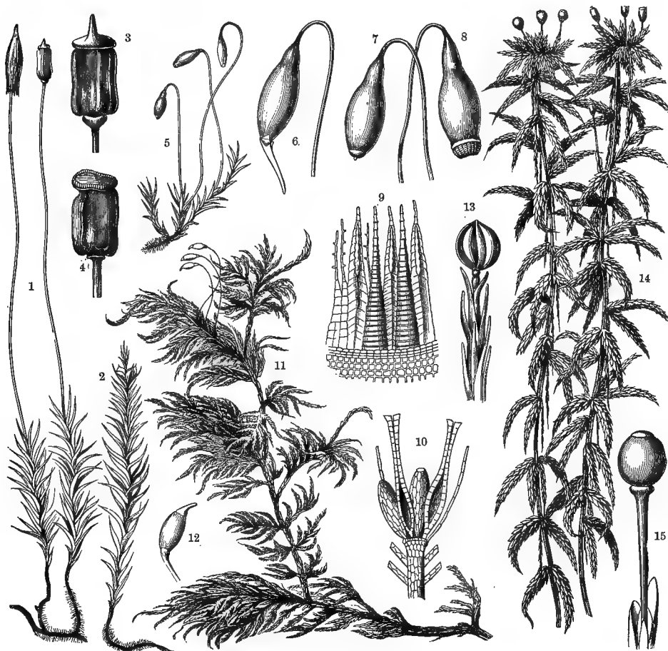
Fig. 191.—Mosses.
