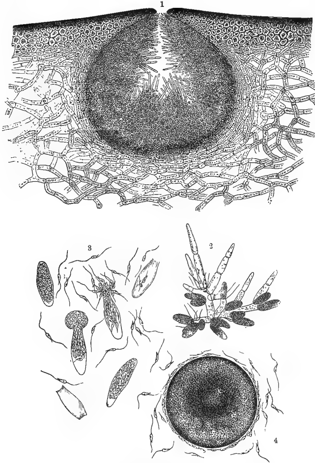
Fig. 203.— Fucus vesiculosus .
