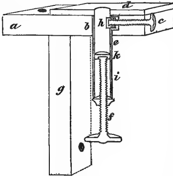
fig. 214. Cutting Machine.
