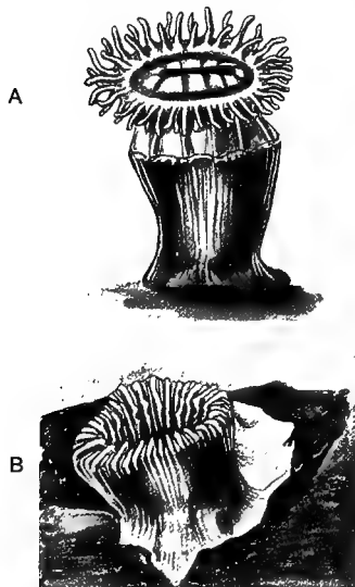
FIG. 22.—The Devon Cup Coral ( Caryophyllia smithii ).
