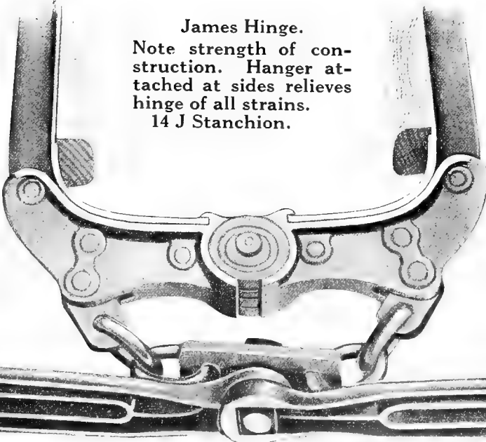
Actual size of rivet in hinge.
