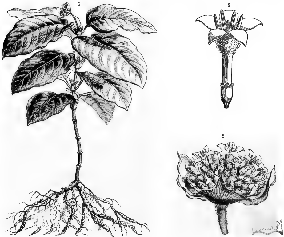
Fig. 432.—Caprifoliales: Cephaelis Ipecacuanna (Family Rubiaceæ).
