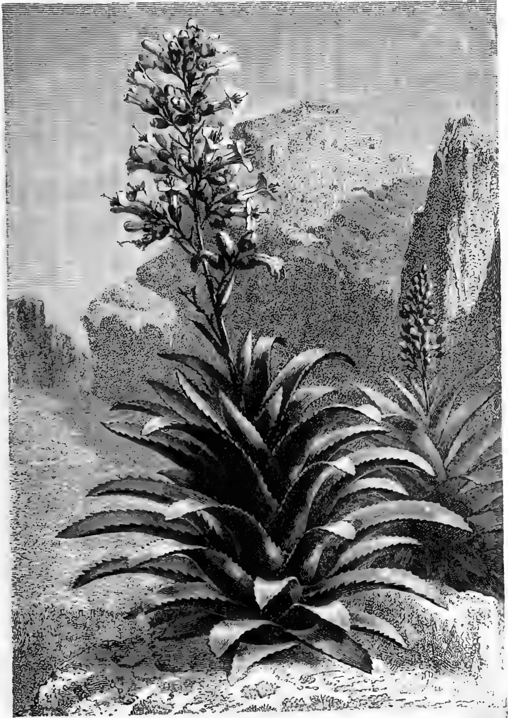
Fig. 410.— Echmea paniculata (after Baillon).
