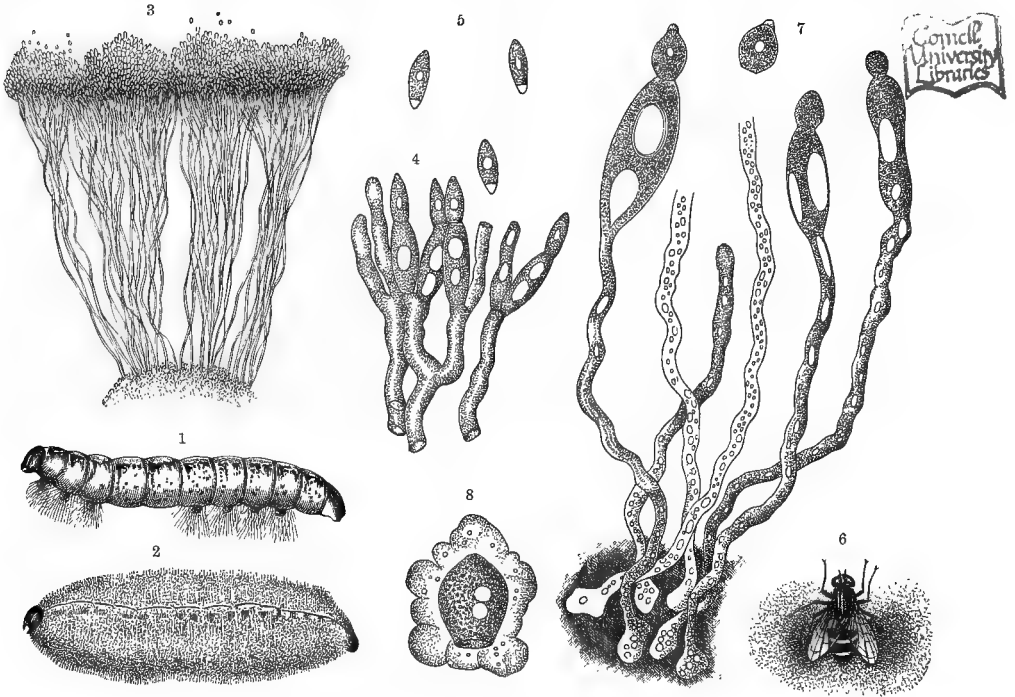
Fig. 383.—Entomophthoræ: Entomophthora and Empusa .
