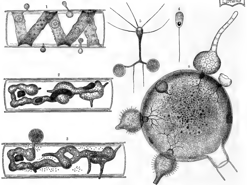
Fig. 379.—Chytridiaceae and Ancylistaceae.
