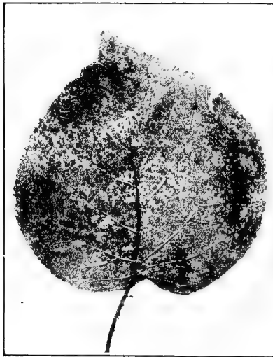
FIG. 43. — Apricot-rust.
