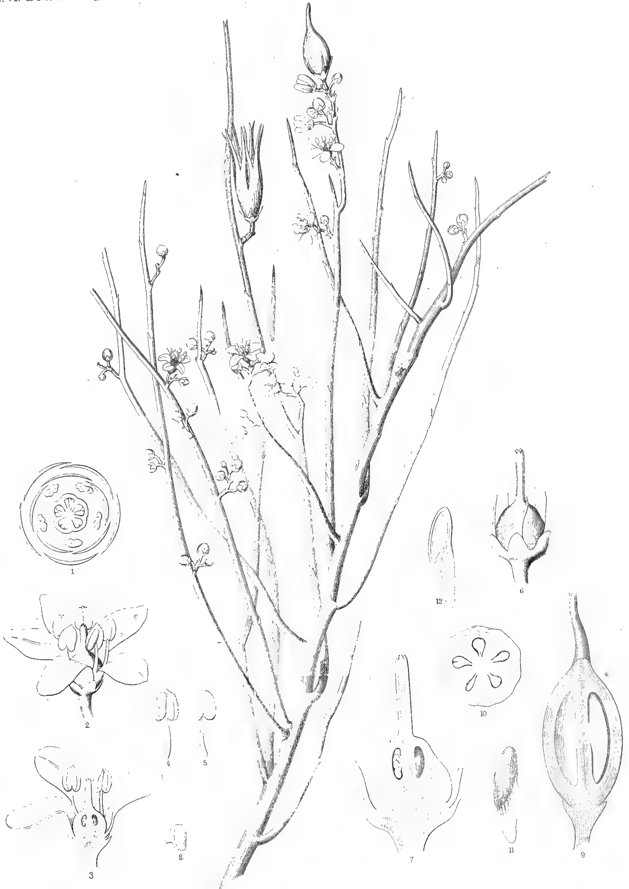
CANGTIA HOLACANTHA.
