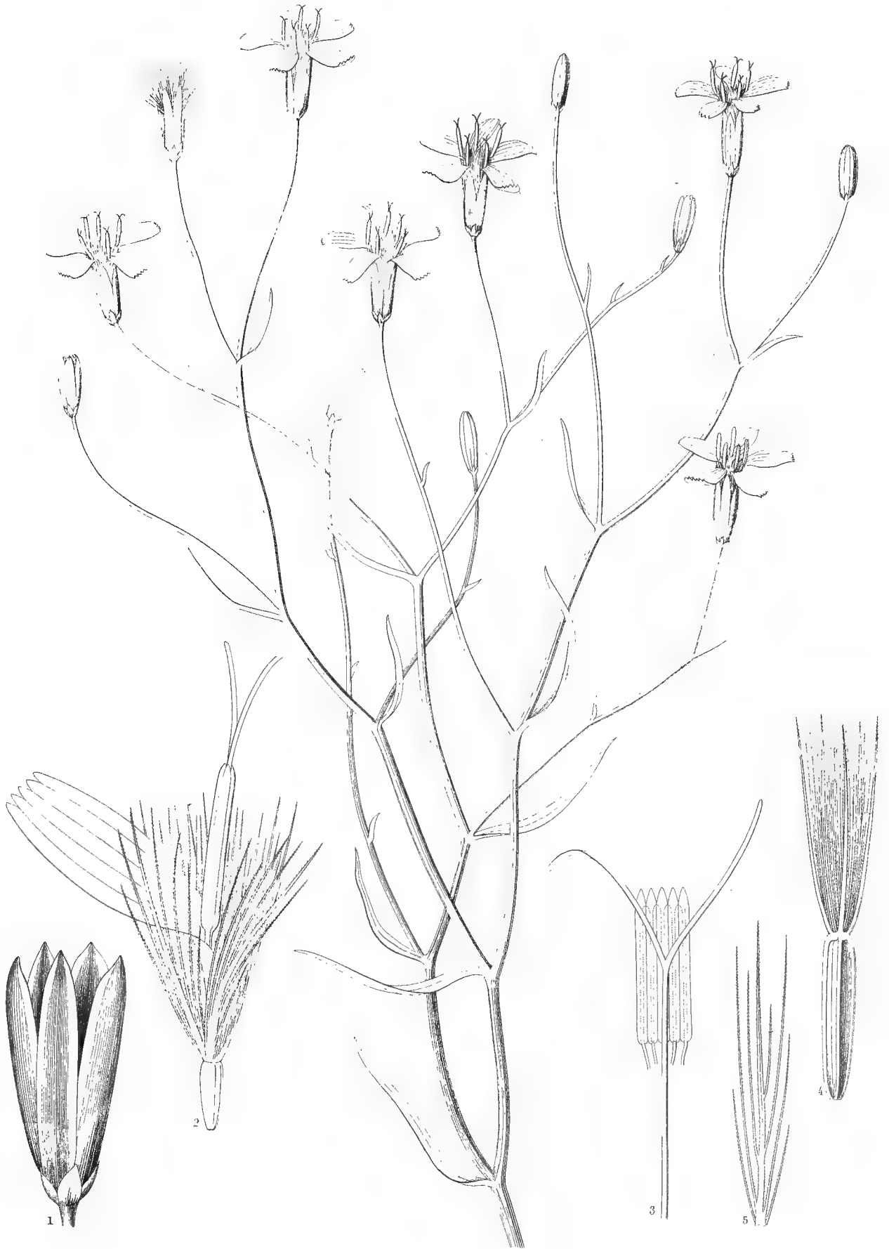
Figs. 1-2 CHÆTADELPHA WHEELERI.
