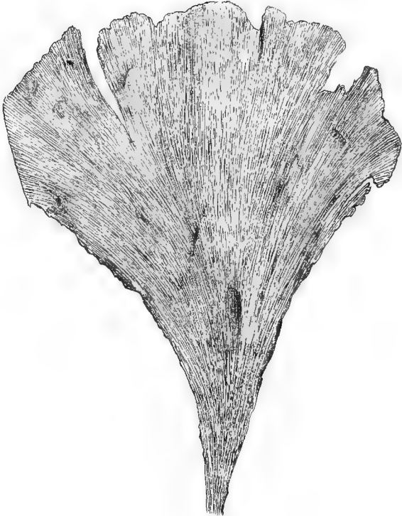
FIG. 665. Psygmophyllum flabellatum . (Brit. Mus. No. 40578; ca. \frac{2}{3} nat. size.) M. S.
