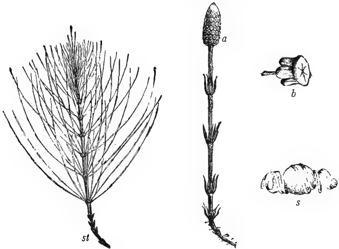
FIG. 299. — EUISETUM ARVENSE.
