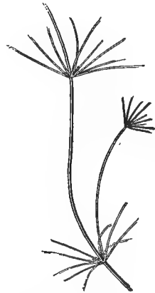
FIG. 270. — NITELLA.
