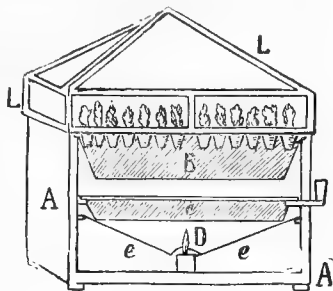
49. Propagating-oven.
