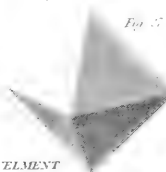
Regular Octahedron. Fig. 15.
