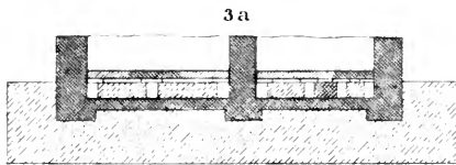
SCHNITT-E-F-
