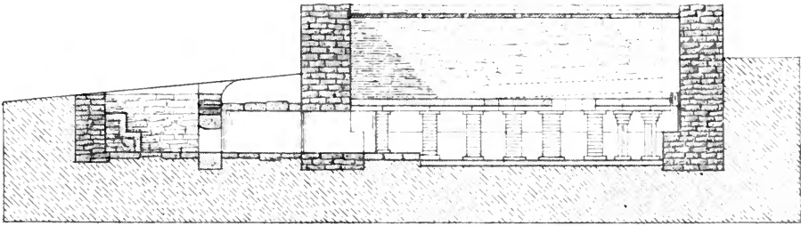
SCHNITT-A-B-
