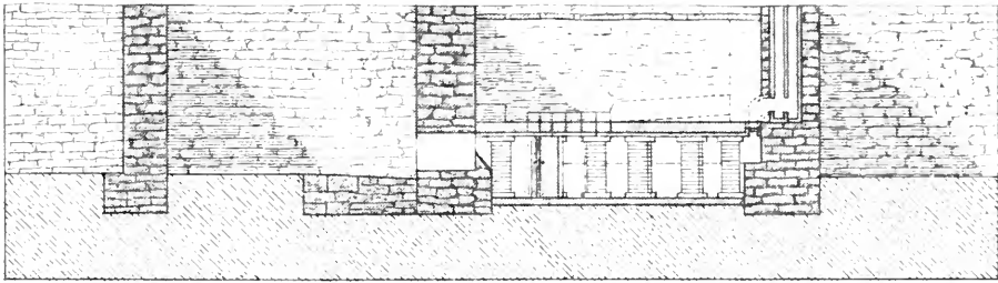
SCHNITT-C-D-
