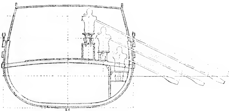
1692 Entwurf einer Triere von Lemaitre.
