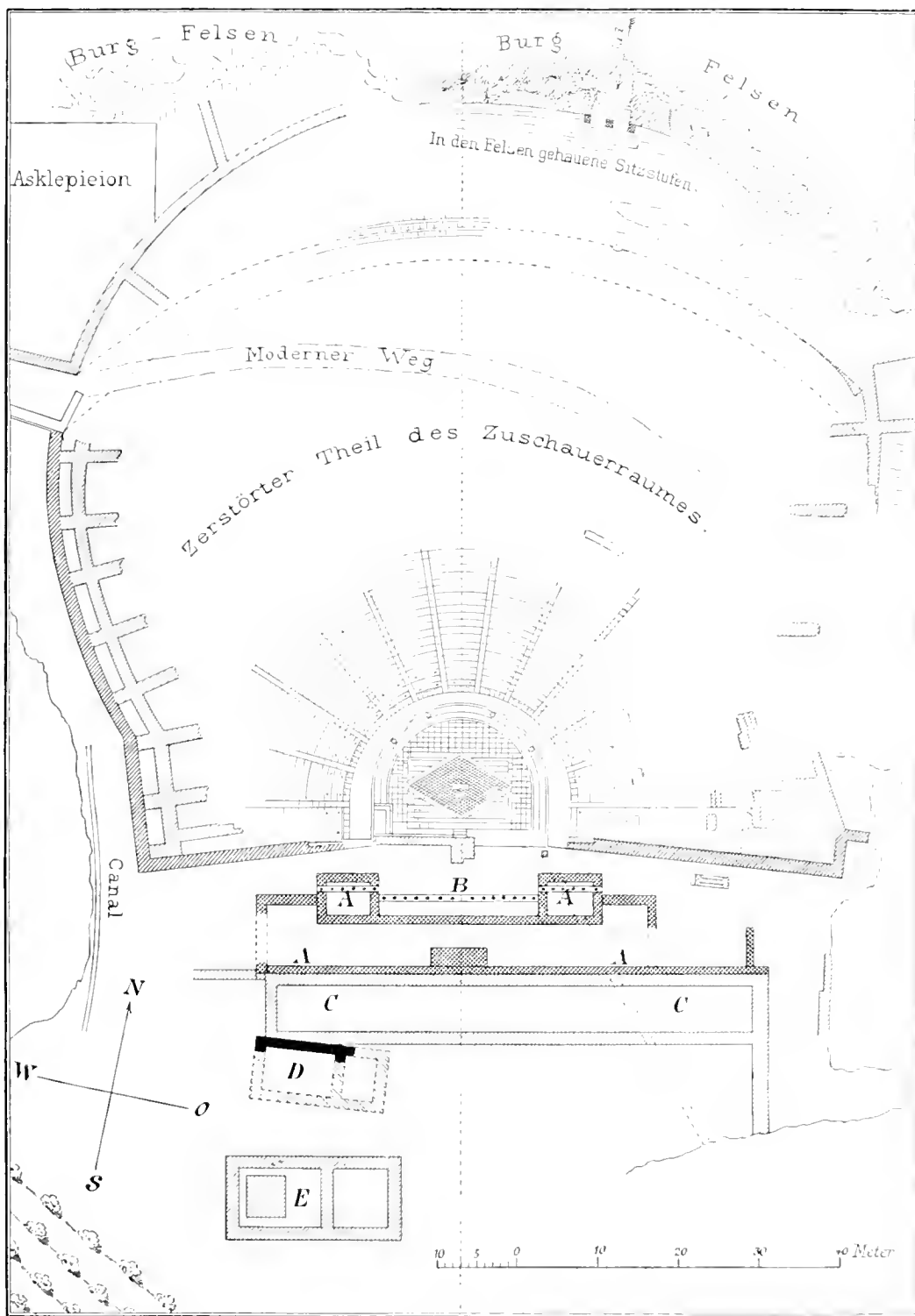
1816 Grundriss des Dionysos-Theaters zu Athen, nach Originalzeichnung. (Zu Seite 1736.)
