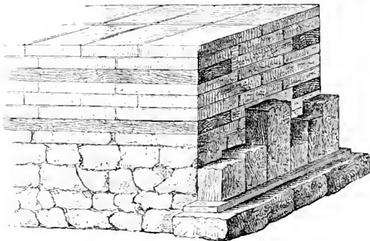
2004 Mauerbau.
