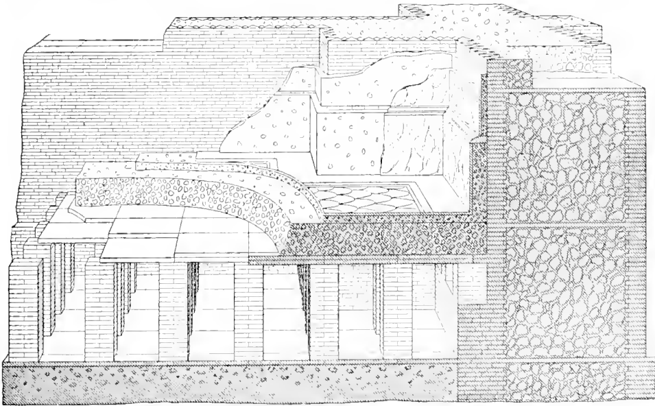
1852 Heizvorrichtung in den Badern; Konstruktion von A. Blouet. (Zu Seite 1765.)
