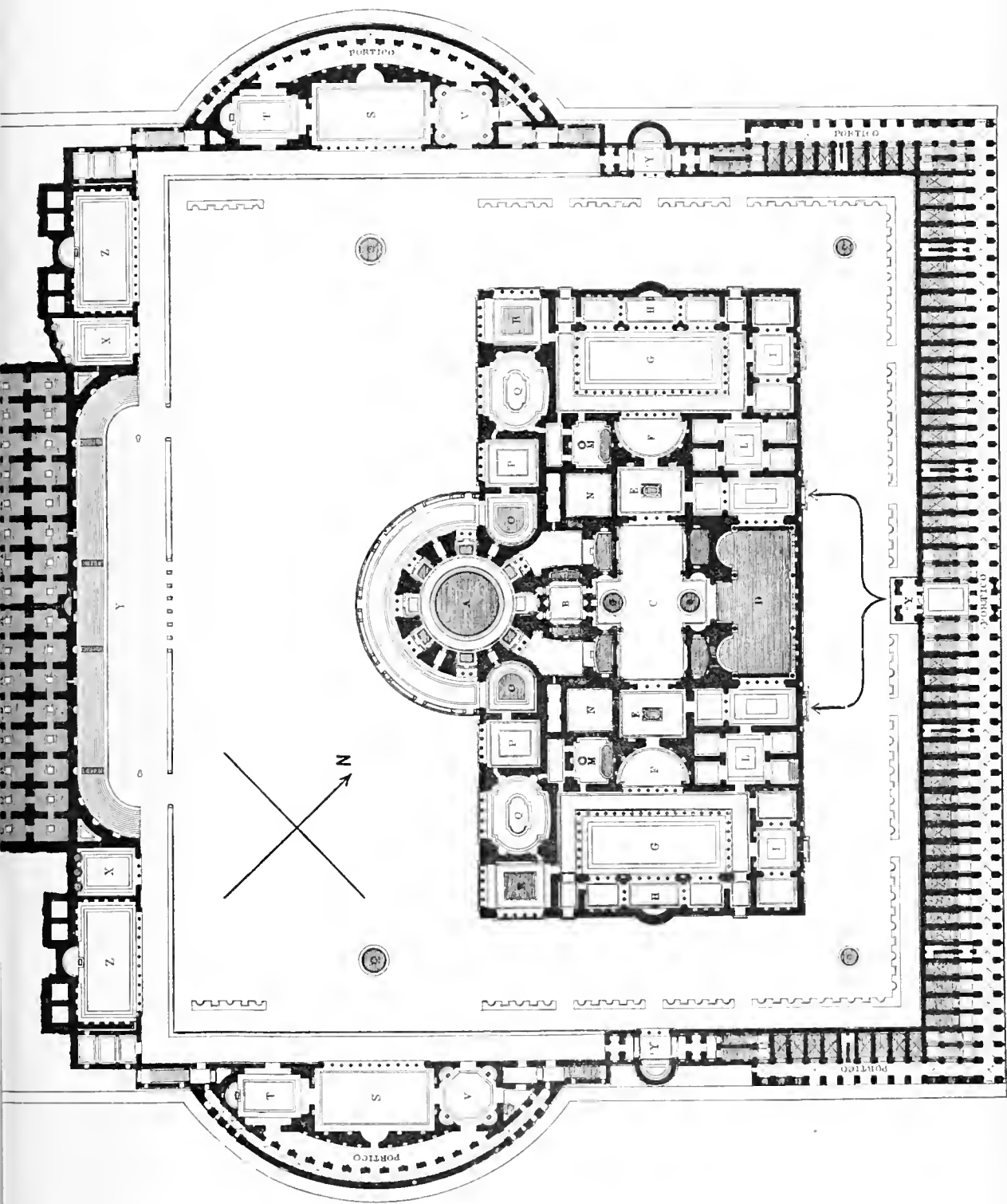
1855 Grundriss der Thermen des Caracalla in Rom. (Zu Seite 1771.)
