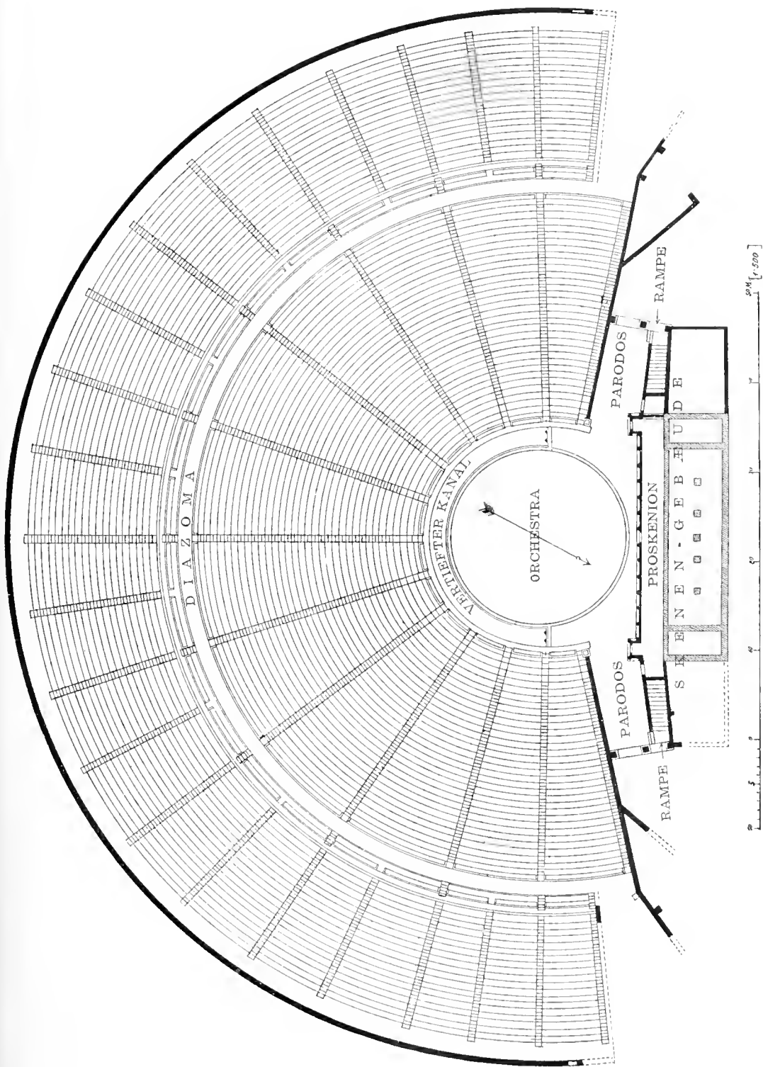
1814 Grundriss des Theaters zu Epidaurus. (Zu Seite 1734.)
