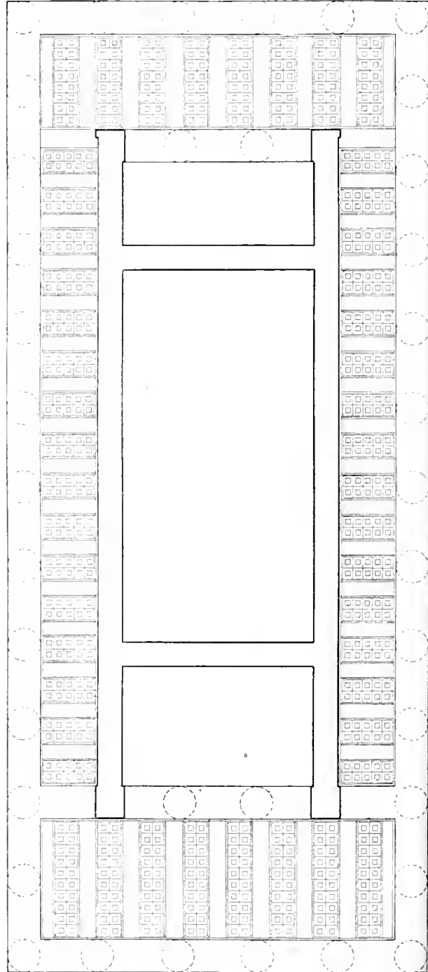
VNTERANSICHT DER PTERONDECKE
