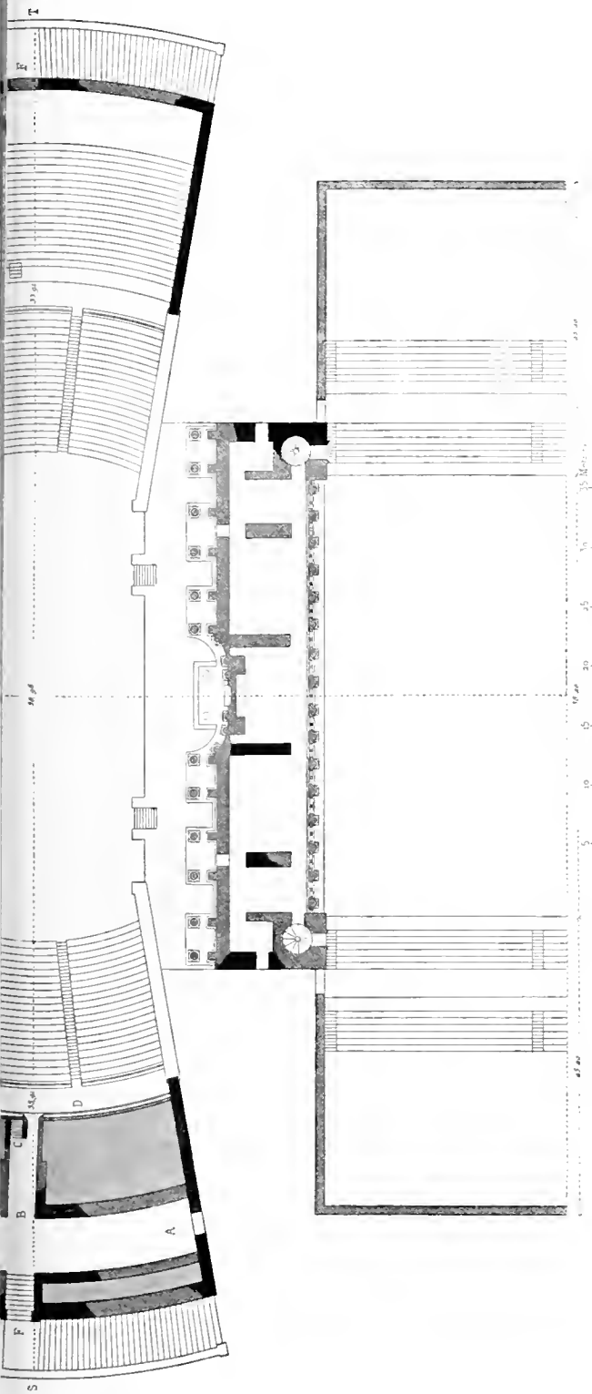
Grundriss des Theaters von Alzani nebst einem Teile vom anstossenden Stadion; vgl. Abb. 1865 auf Taf. LXV.
