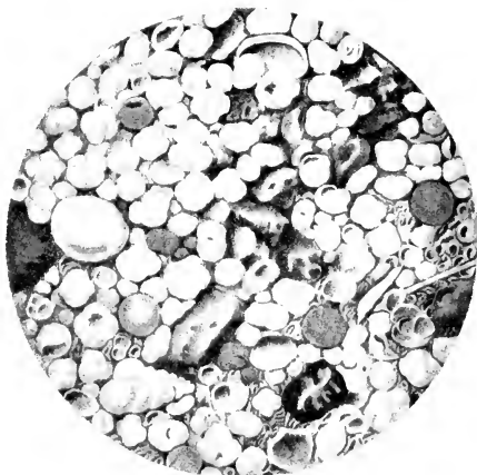
FIG. 139.—GLOBIGERINA OOZE.
