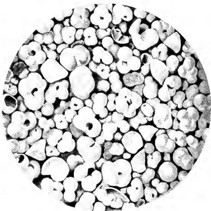
FIG. 138.—GLOBIGERINA OOZE.
