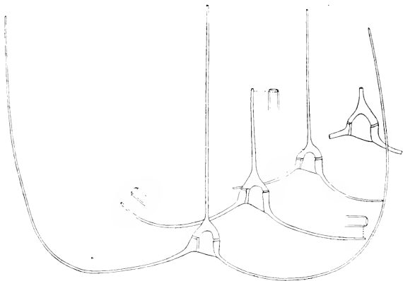
FIG. 227.— CERATIUM TRICHOCEROS .
