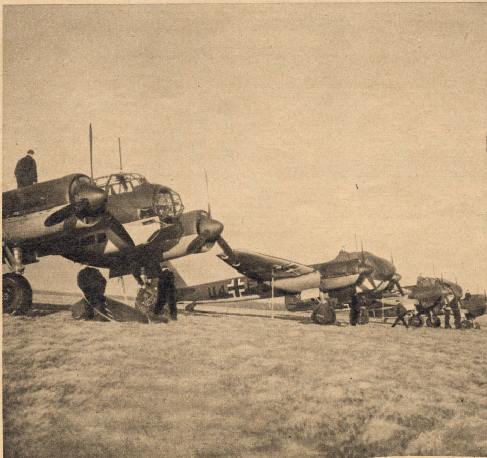
Durch die Einstieggondel geht die Besatzung an Bord des Horizontal- und Sturzbombers Ju 88, der mit den neuesten Errungenschaften der Kampftechnik ausgestattet ist und überall mit durchschlagendem Erfolg die Zentren der militärischen Widerstandskraft Englands angegriffen hat
